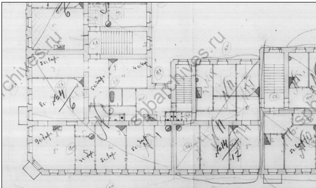
Илл. 8. План 3-4-го этажей. 1883 г. Фрагмент. ЦГИА СПб. Ф. 515. Оп. 4. Д. 2250. Л. 24 – 25.
