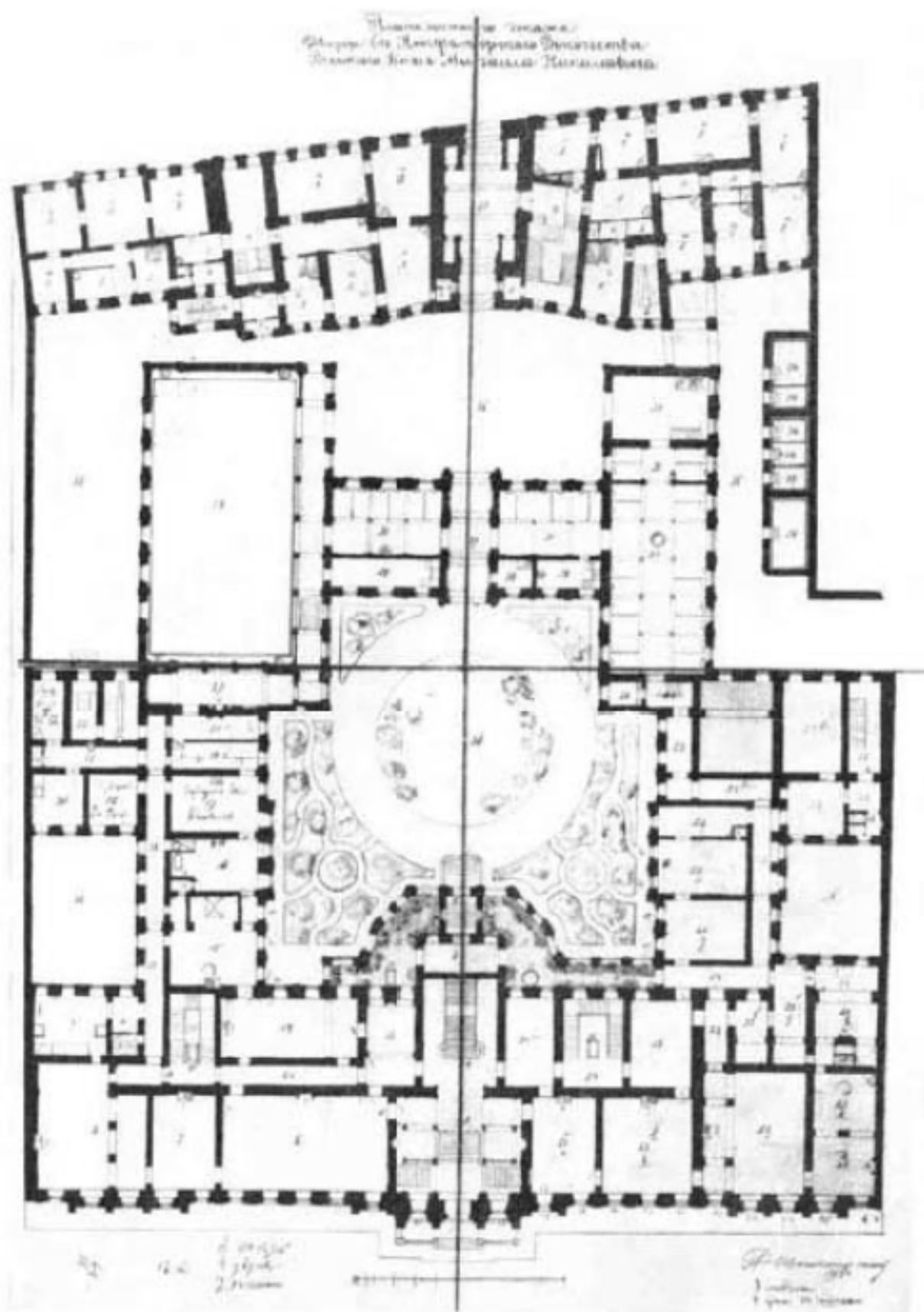
5. План первого этажа Ново-Михайловского дворца. Штакеншнейдер. 1859 г.
