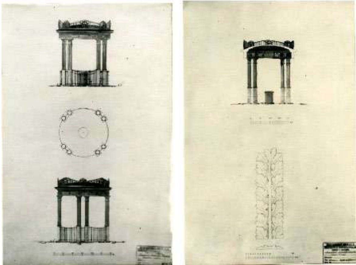
32. Соколов А.М. Беседка памятника великой княгине Александре Павловне. Обмерный чертеж. Бумага, тушь. 1940г. Архив ГМЗ «Павловск»
