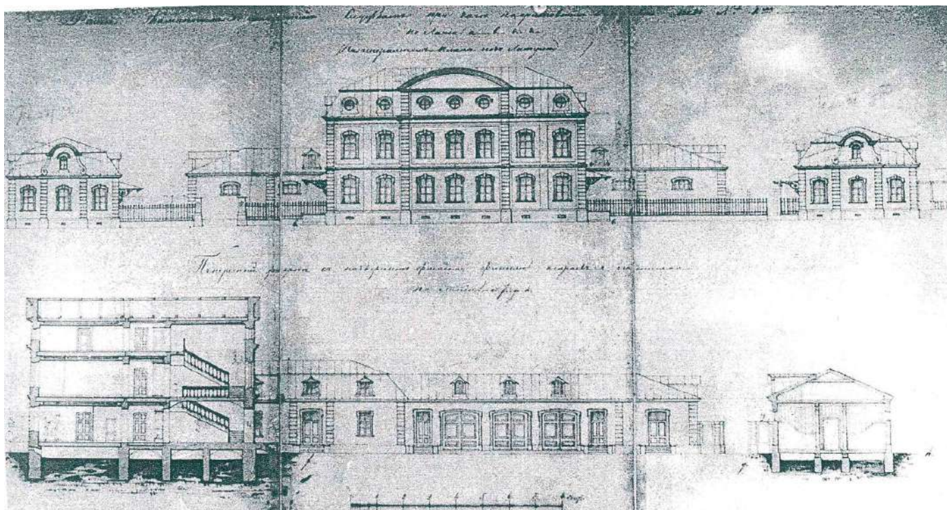
Илл. 13. Фасад и разрез каменных служб при главной даче острова. РГИА Ф. 1424 Оп. 2 Д. 179.
