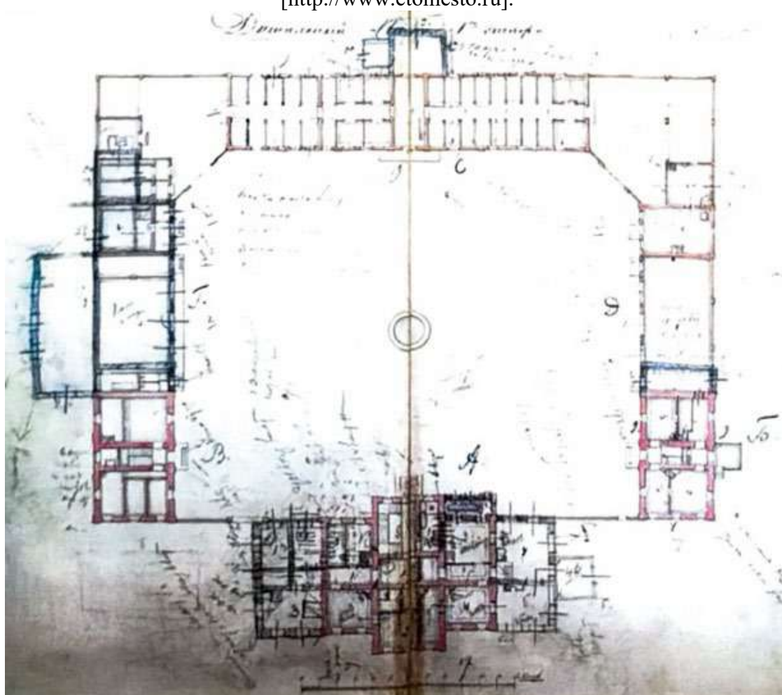
Илл. 11. Планы 1-го этажа каменных служб при главной даче острова. РГИА Ф. 1424 Оп. 2 Д. 179.
