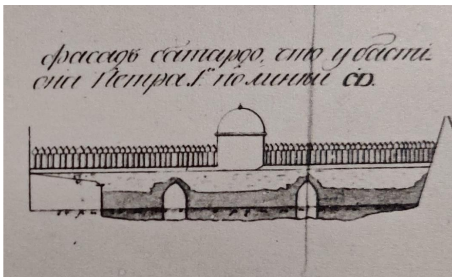
19. Фрагмент чертежа ботардо у Государева бастиона, ботардовых ворот, Невской пристани и др. частей СПб-й крепости. 1807 г. РГА ВМФ. Ф. 3/л. Оп. 34. Д. 2952.
