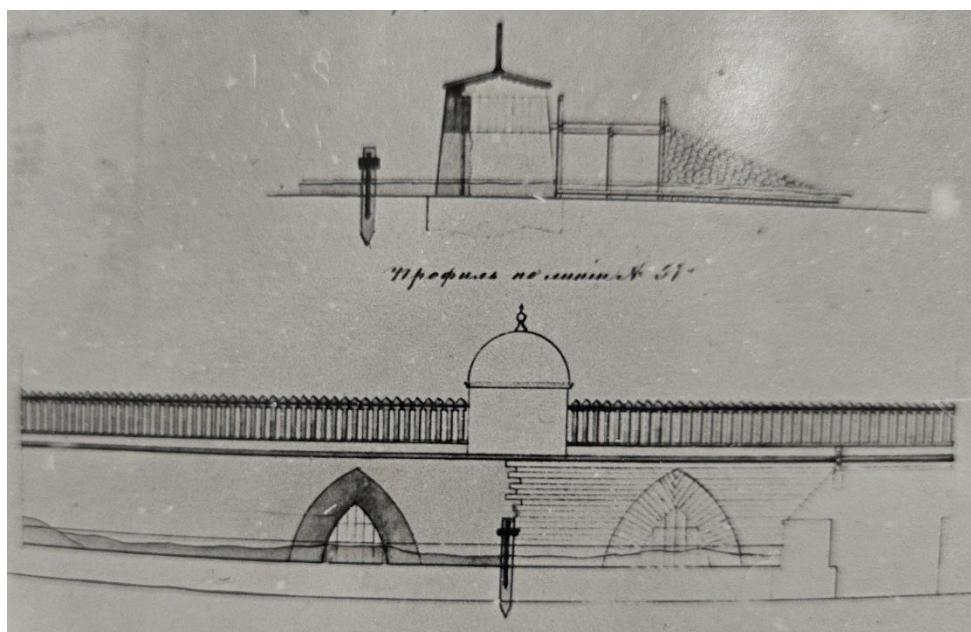
27. Фрагмент фасада и профиля ботардо у шпика бастиона Меншикова (Петра II). 1860 г. РГА ВМФ. Ф. 3/л. Оп. 35. Д. 4931.
