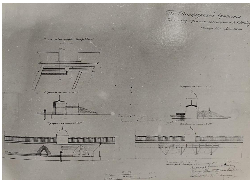
26. План, фасады и профили ботардо у шпика бастиона Меншикова (Петра II). 1860 г. РГА ВМФ. Ф. 3/л. Оп. 35. Д. 4931.
