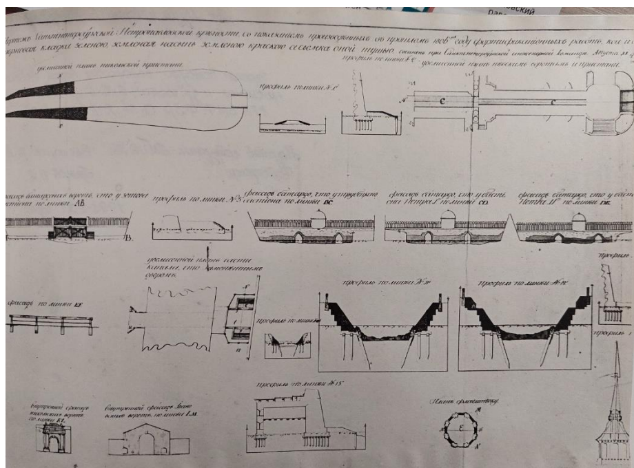
18. Чертеж ботардо, ботардовых ворот, Невской пристани и др. частей СПб-й крепости. 1807 г. РГА ВМФ. Ф. 3/л. Оп. 34. Д. 2952.
