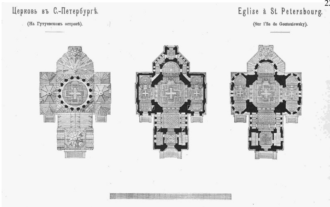
Илл. 3. Изображения из журнала "Зодчий". 1891г.— Citywalls.ru — архитектурный сайт Петербурга [Электронный ресурс]. URL: http://www.citywalls.ru/house3729
