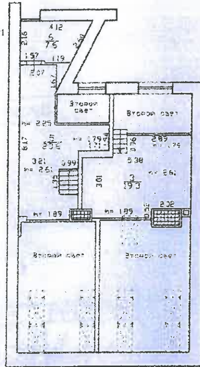
План мансарды
