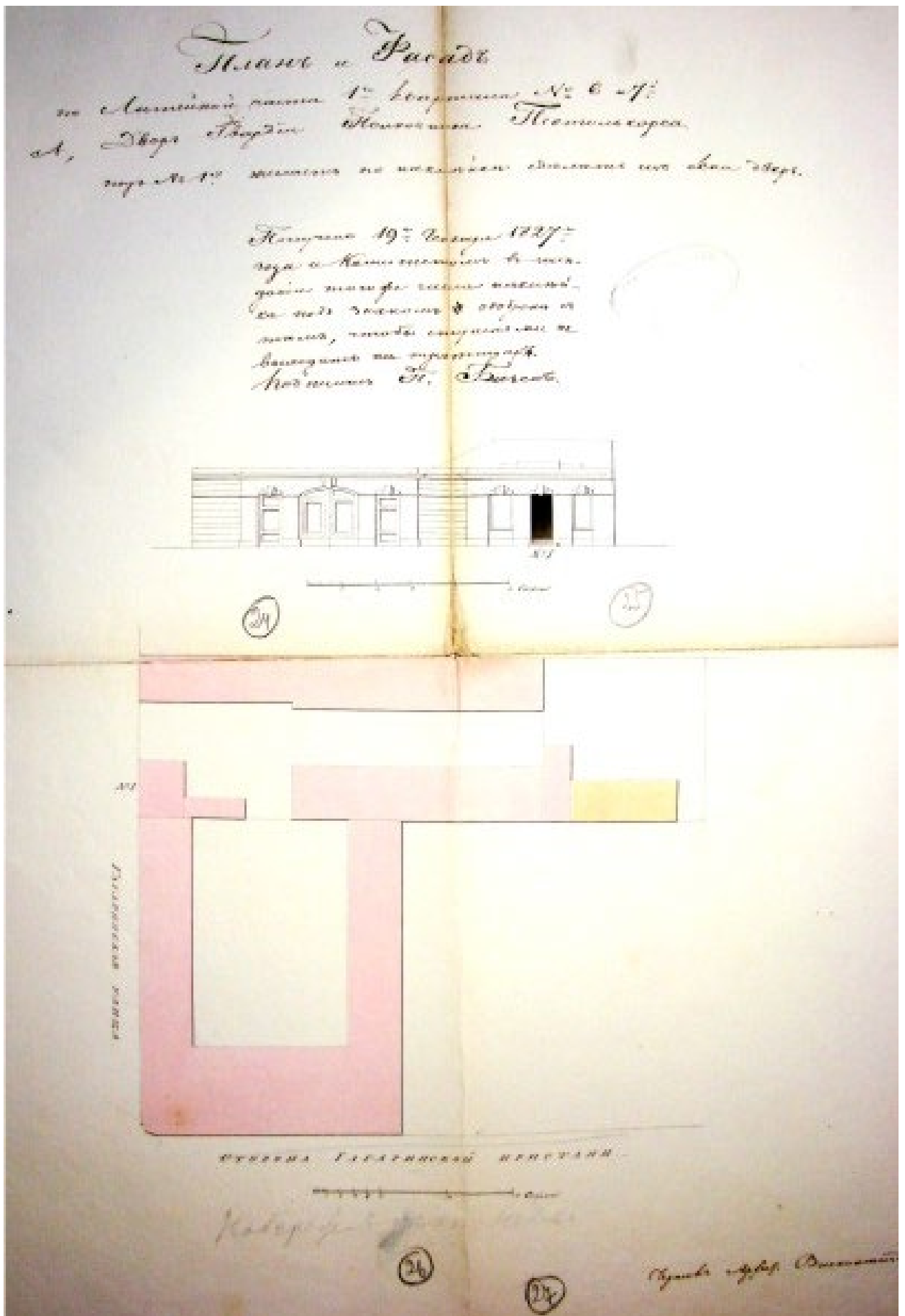
Илл. 5. План двора дома гвардии полковника Пестольхора. Арх. Д.И.Висконти. 1827 г. ЦГИА СПб. Ф. 513. Оп. 102. Д. 3989. Л. 5-8.
