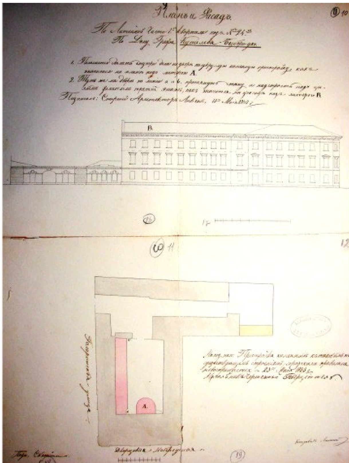
Илл. 6. План двора и фасад дома графа А.Г.Кушелева-Безбородко. Арх. И.П.Скотти. 1835 г. ЦГИА СПб. Ф. 513. Оп. 102. Д. 3989. Л. 9-12.
