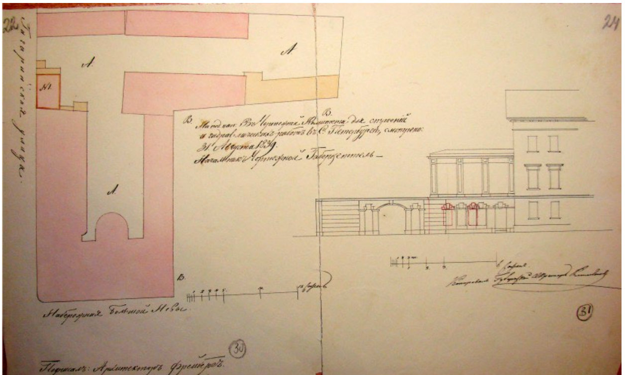
Илл. 7. План двора и фрагмент фасада дома графа А.Г.Кушелева-Безбородко. Проект галереи. Арх. Фрейберг. 1839 г. Арх. Фрейберг. 1839 г. – ЦГИА СПб. Ф. 513. Оп. 102. Д. 3989. Л. 22-24.
