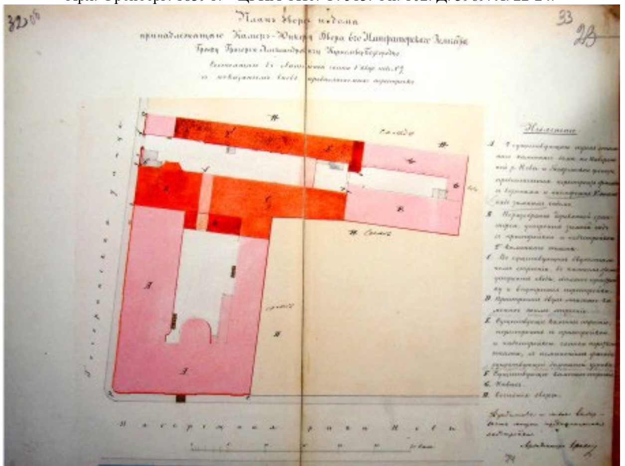
Илл. 8. Проект перестройки северного и надстройки 3-м этажом части южного дворового флигеля. Арх. Р.Р.Генрихсен. 1857 г. ЦГИА СПб. Ф. 513. Оп. 102. Д. 3989. Л.32 об.-33.
