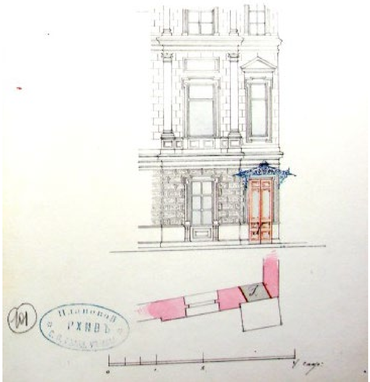
Илл. 15. Проект обращения окна в дверь в 1-м этаже лицевого дома. Арх. А.Бруни. 1880 г.
