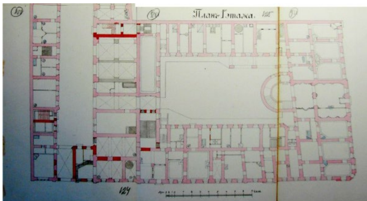
Илл. 18. Проект надстройки 2-го этажа на месте проездных ворот дома купца А.Г.Елисева. Фрагмент плана 1-го этажа. Арх. А.К.Гаммерштедт. 1893 г. ЦГИА СПб. Ф. 513. Оп. 102. Д. 3989. Л. 123-126.
