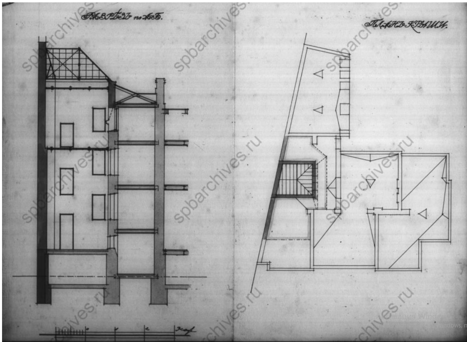
38. Разрез по А. Б. План крыши. Архитектор М. С. Ляевич, 18 мая 1912 г. ЦГИА СПб. Ф.513. Оп.102. Д.7800. Л. 41-42.
