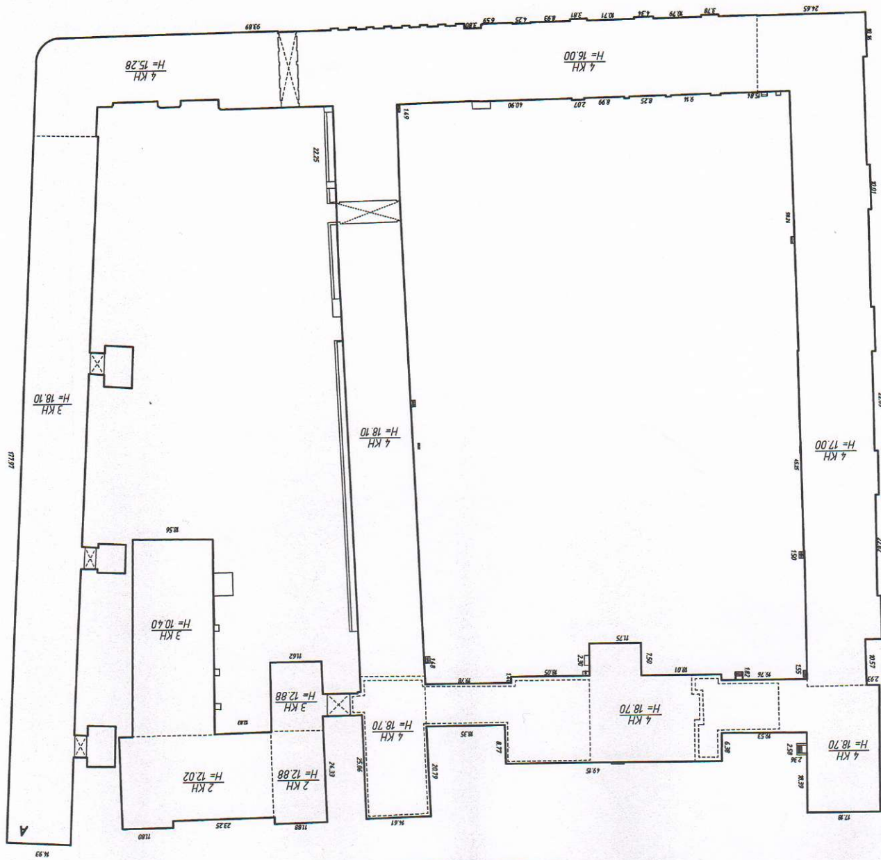
Ситцевый план строения по адресу: 2. Санкт-Петербург, улица Комсомола, дом 22, лит. А
