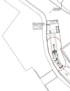
Схема устройства площадки и разработки грунта на 3 этапе
