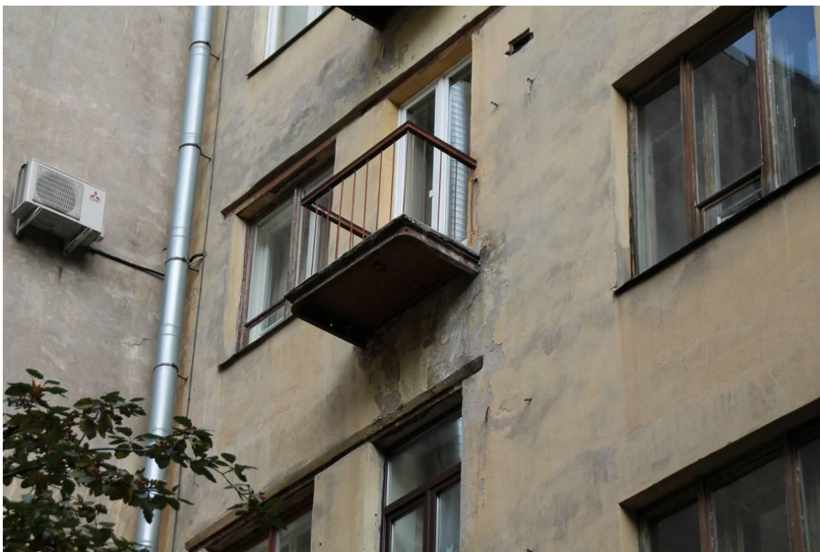
Рис. 9 Общее увлажнение, загрязнение, проявление сетки усадочных волосяных трещин на поверхности фасада. Деструкция штукатурного слоя. Коррозия металлических балок под балконной плитой. Повреждения балконной бетонной плиты и ограждения балкона.
