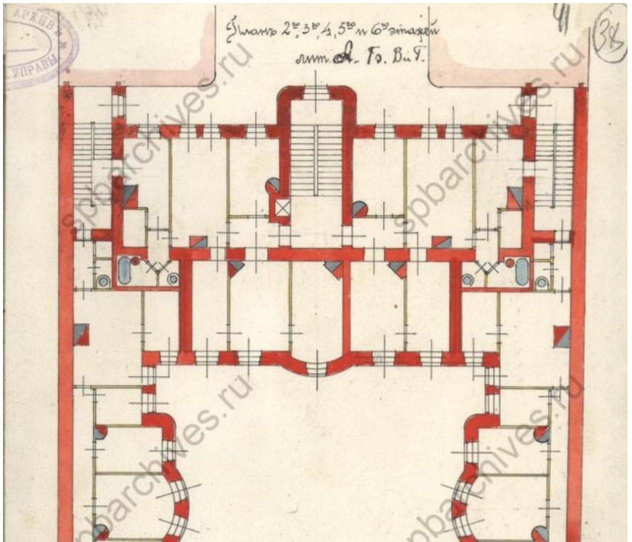
30. ЦГИА СПб. Фонд 513. Описание 102. Дело 4142 Чертежи дома на участке, принадлежавшем Н. П. Штакельберг, И. А. Захарову, М. Г. Гольмдорфу, М. М. Верховскому по Кирочной ул., 22. 1836-1910. План 2,3,4,5,6-го этажей. 1910г. Фрагмент.
