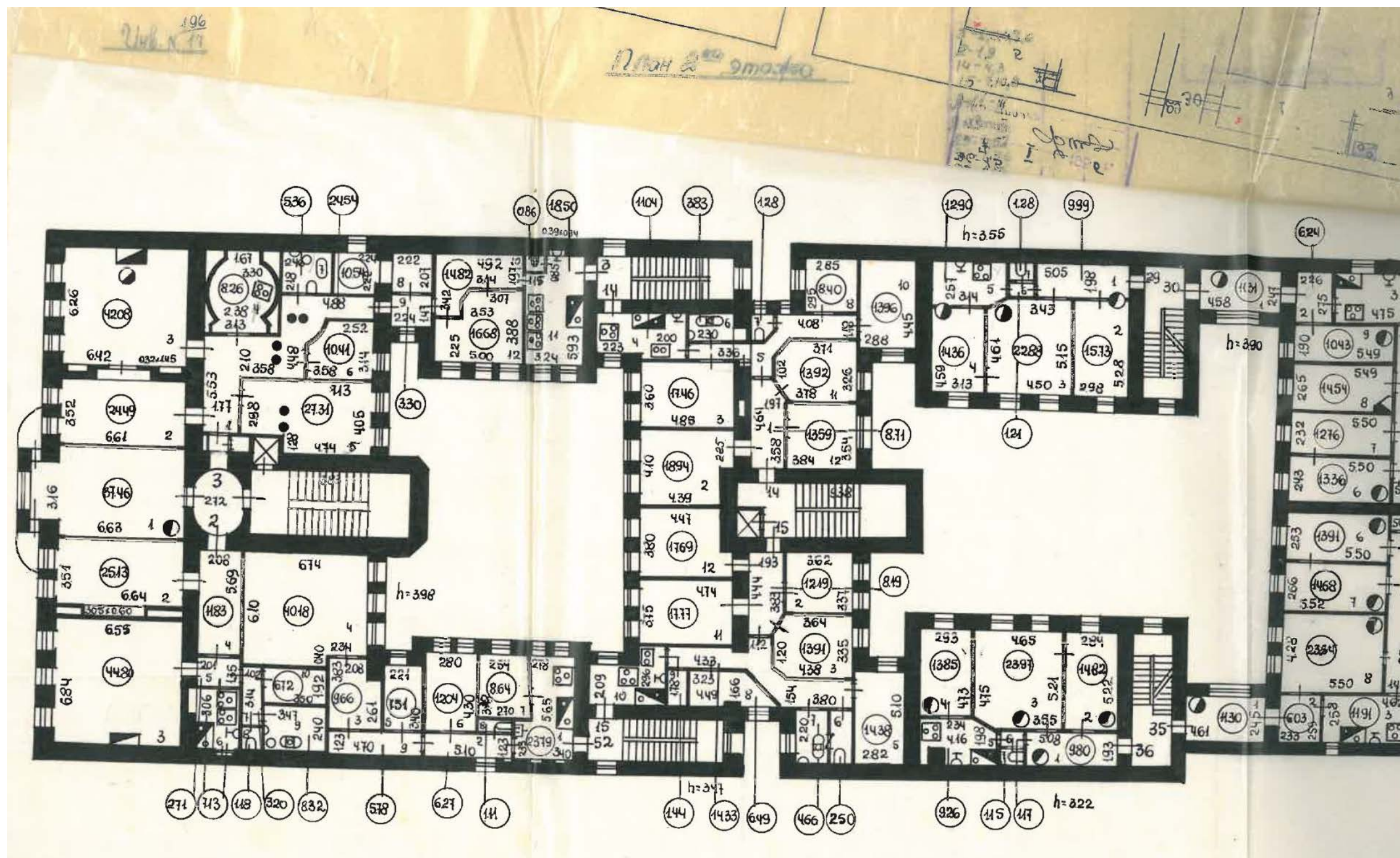
Материалы технической инвентаризации домовладения по адресу Кирочная, дом 22 за «1930-1953» годы. План 2-го этажа. 1953г.
