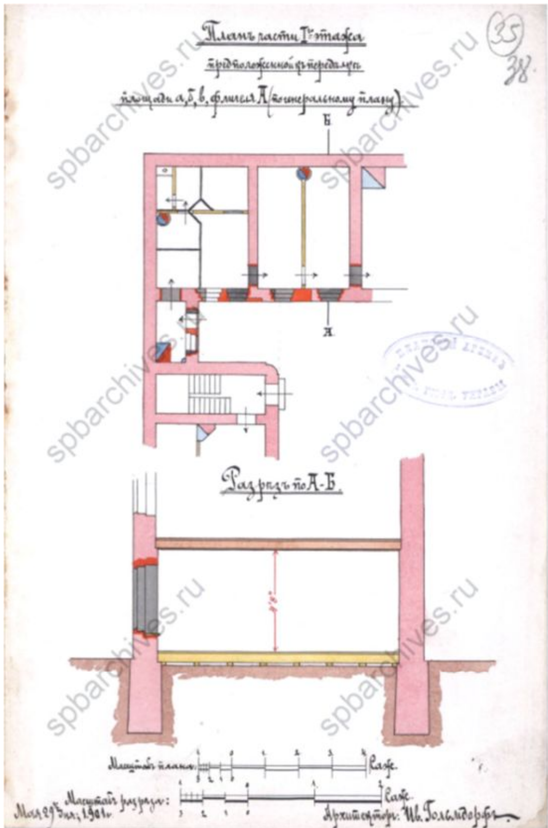
24. ЦГИА СПб. Фонд 513. Опись 102. Дело 4142 Чертежи дома на участке, принадлежавшем Н. П. Штакельберг, И. А. Захарову, М. Г. Гольмдорфу, М. М. Верховскому по Кирочной ул., 22. 1836-1910. Разрез и План части 1-го этажа, 1901г.
