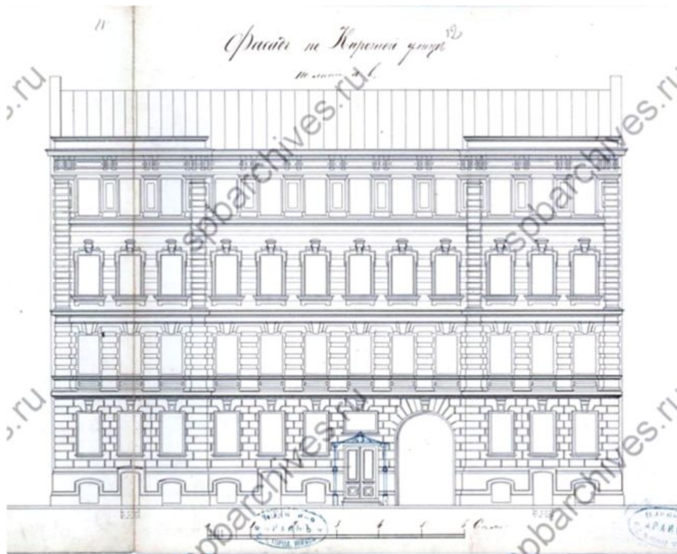
14. ЦГИА СПб. Фонд 513. Опись 102. Дело 4142 Чертежи дома на участке, принадлежавшем Н. П. Штакельберг, И. А. Захарову, М. Г. Гольмдорфу, М. М. Верховскому по Кировной ул., 22. 1836-1910., Фасад дома И.А.Захарова. 1881г.
