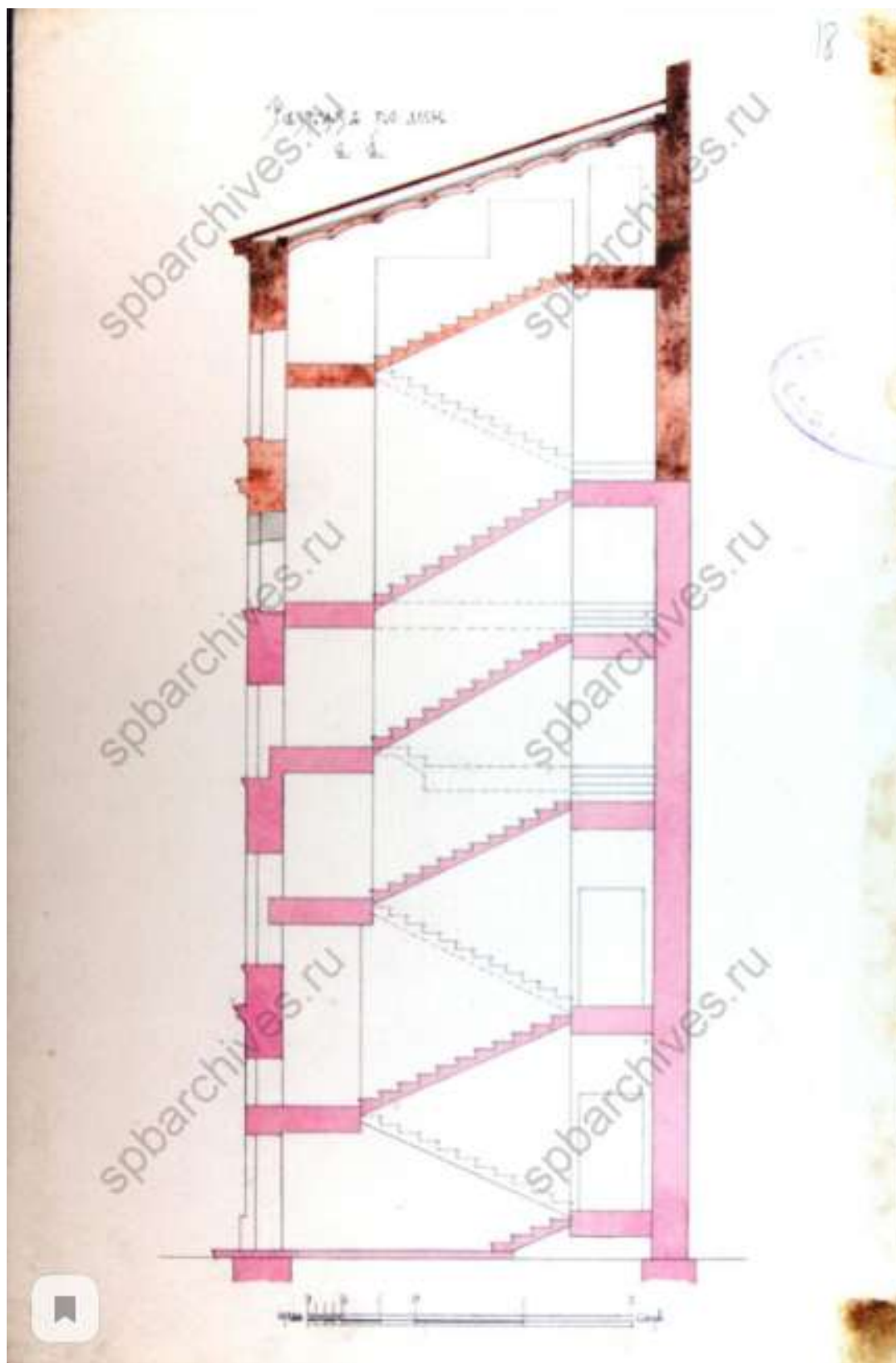
Илл. 15. Чертежи дома на участке, принадлежавшем А. и В. Голенищевым-Кутузовым, Гагариным, А.П. Гагарину по Михайловской пл., 3. Разрез по линии а-в [1899 г.] – ЦГИА СПб, Ф. 513, оп. 102, д.9797. 1841-1907 гг.
