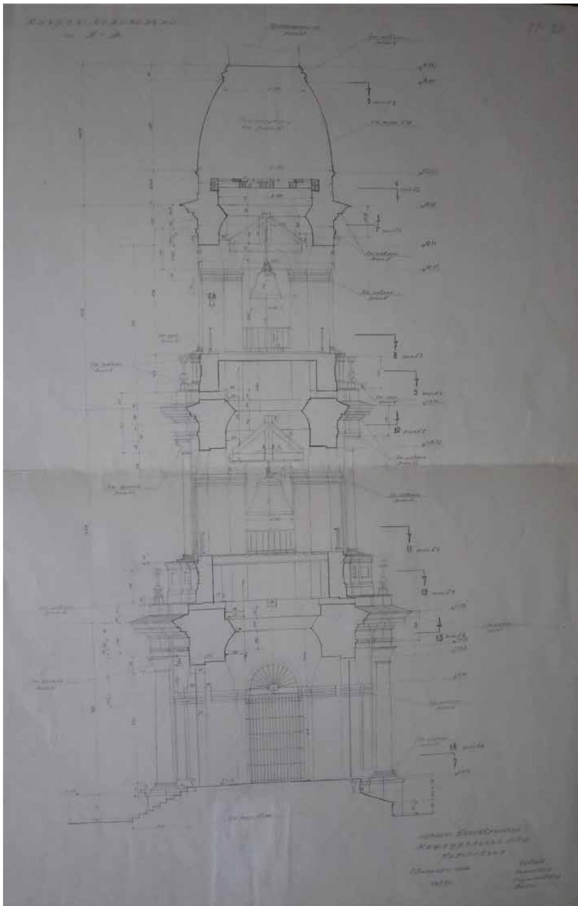
Илл. 56. Колокольня Николо-Богоявленского Морского собора. Разрез колокольни. Обмерный чертеж. Арх-ры: Савков В.М., Казанская Е.В., Корженевская Л.М., Якоби В.К. 1956 г. Архив КГИОП (п. 57, Г-14)
