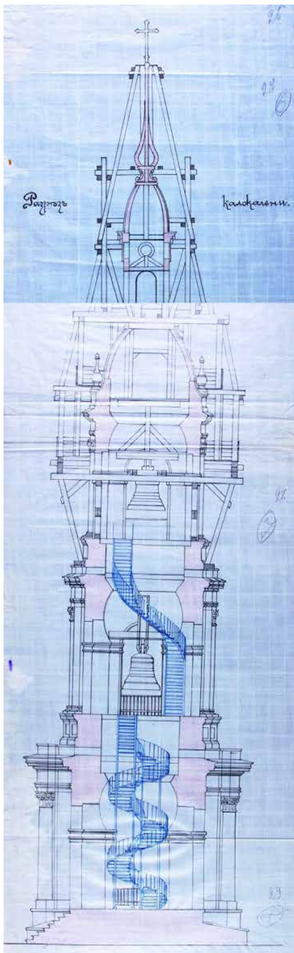
Илл. 20. Разрез колокольни церкви Св. Чудотворца Николая. 1870-е гг. ЦГИА СПб. Ф. 513. Оп. 102. Д. 3256а. Л. 26-29.
