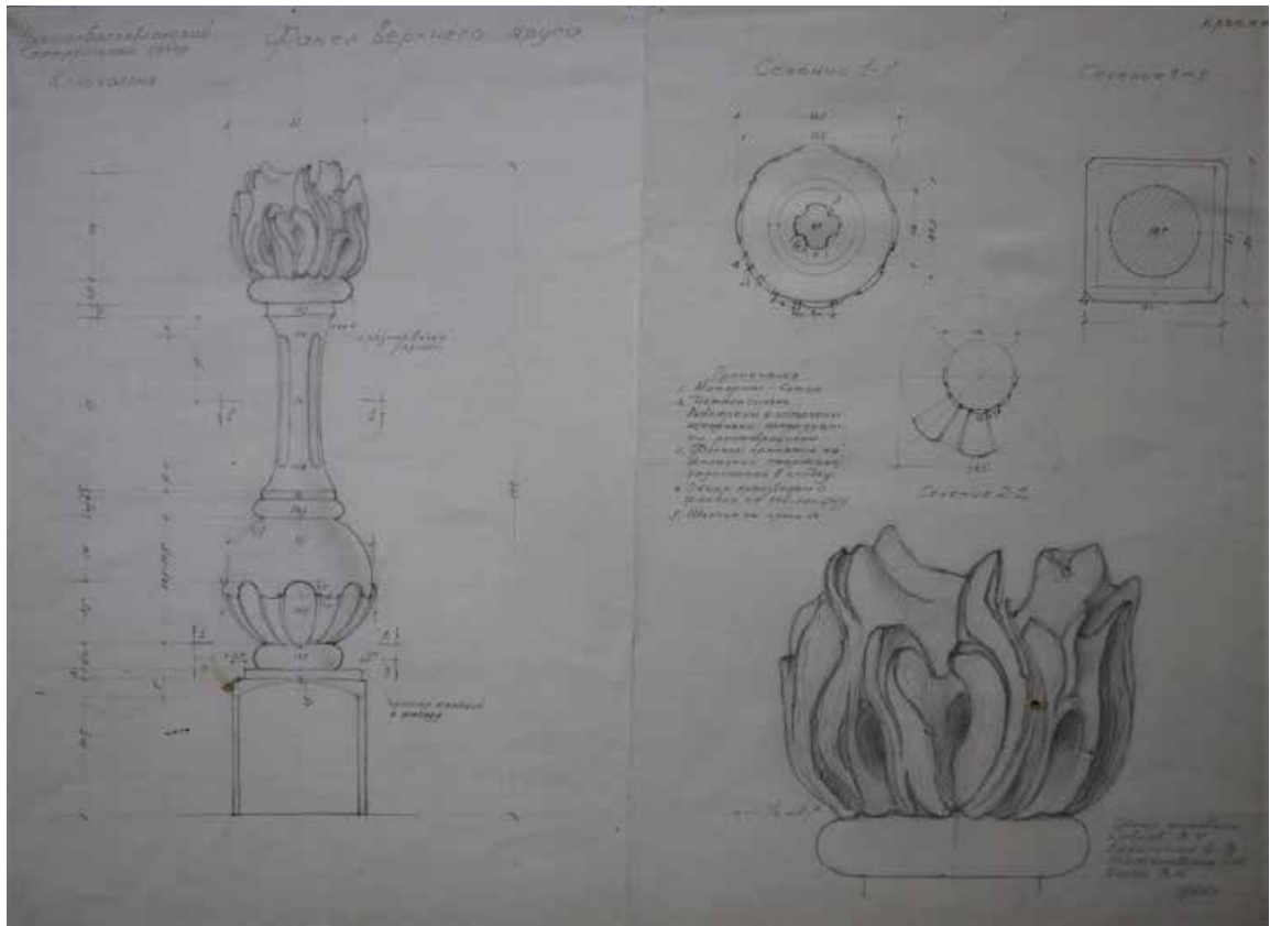
Илл. 57. Колокольня Никола-Богоявленского Морского собора. Факелы верхнего яруса. Обмерный чертеж. Арх-ры: Савков В.М., Казанская Е.В., Корженевская Л.М., Якоби В.К. 1956 г. Архив КГИОП (п. 57, Г-50)
