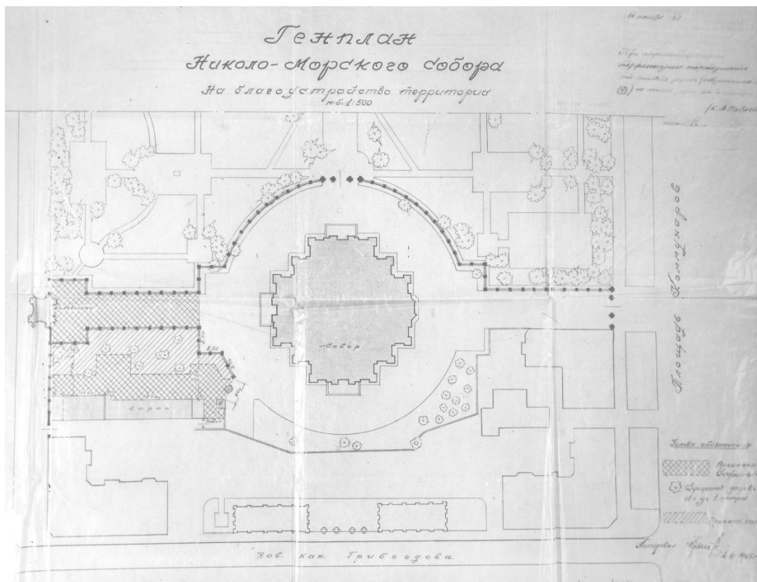
Илл. 65. «Генплан Николо-Морского собора на благоустройство территории». 1969 г. Архив КГИОП (п. 57, пр.-11)
