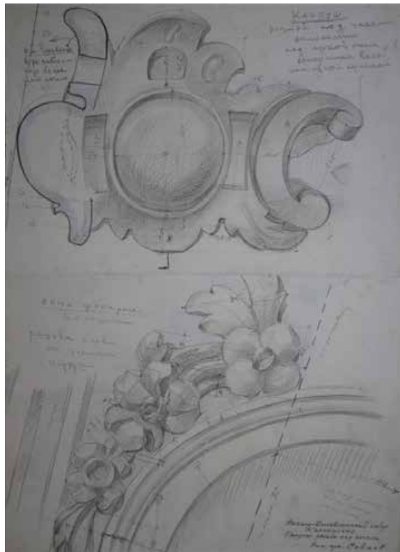
Илл. 60. Колокольня Николо-Богоявленского Морского собора. Картуш и резьба часов. Обмерный чертеж. Арх-р Савков В.М. 1956 г. Архив КГИОП (п. 57, Г-135, Г-136)
