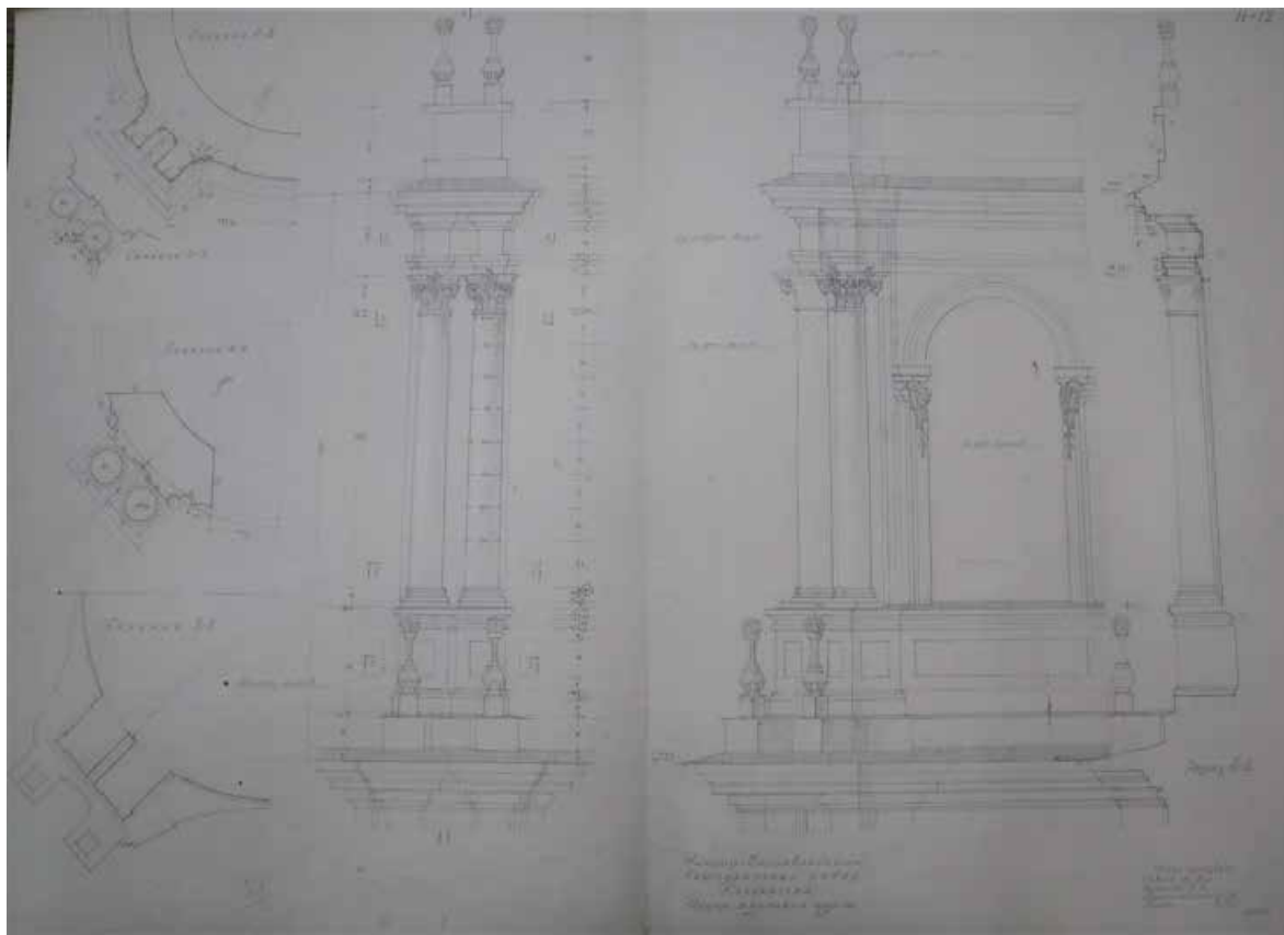
Илл. 59. Колокольня Николо-Богоявленского Морского собора. Ордер 3-го яруса. Обмерный чертеж. Арх-ры: Савков В.М., Казанская Е.В., Корженевская Л.М., Якоби В.К. 1956 г. Архив КГИОП (п. 57, Г-143)
