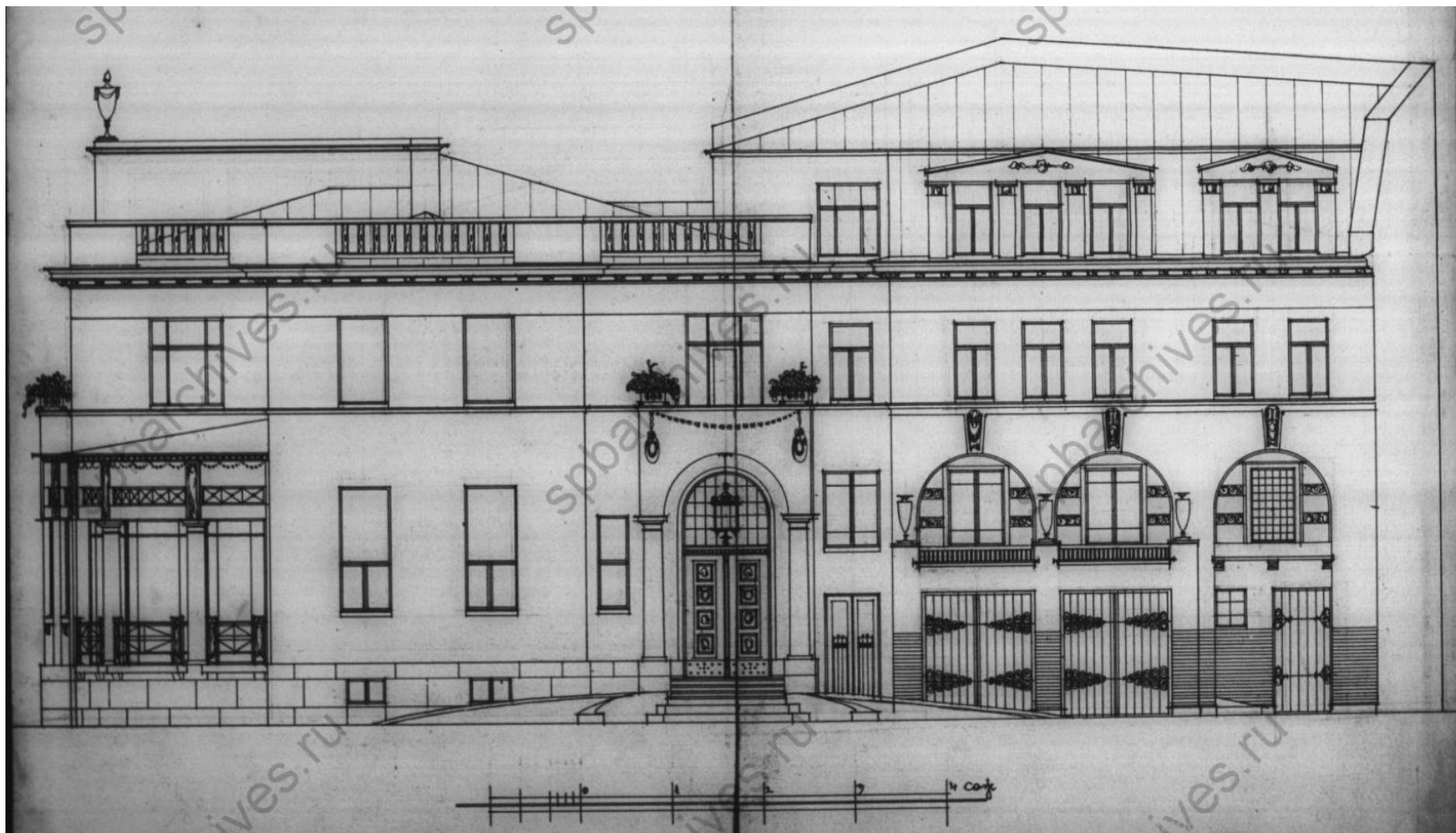
17. Особняк М.К. Покотиловой. Восточный фасад по Каменноостровскому проспекту. Архитектор М.С. Лялевич, 10 марта 1909 г. ЦГИА СПб. Ф.513. Оп.102. Д.7800. Л. 23-24.
