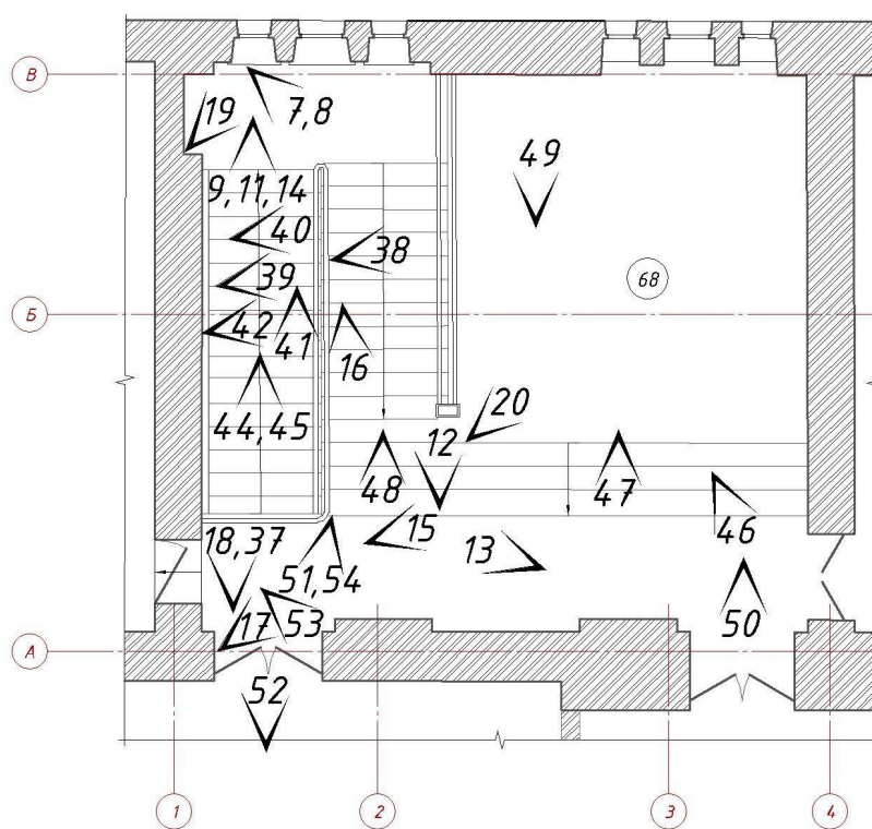
План 2 этажа
