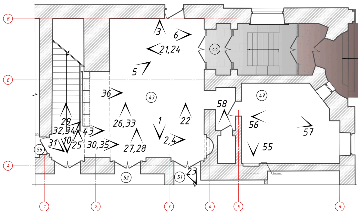
План 1 этажа
