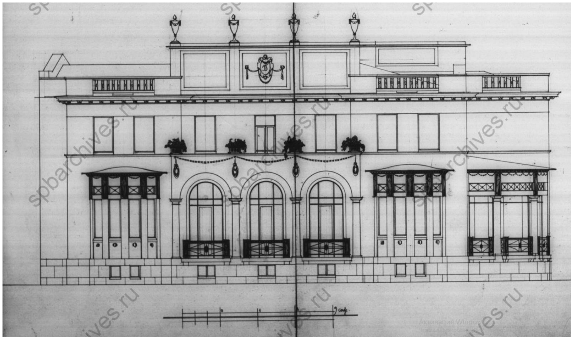
16. Особняк М.К. Покотиловой. Восточный фасад по Каменноостровскому проспекту. Архитектор М.С. Лялевич, 10 марта 1909 г. ЦГИА СПб. Ф.513. Оп.102. Д.7800. Л. 21-22.
