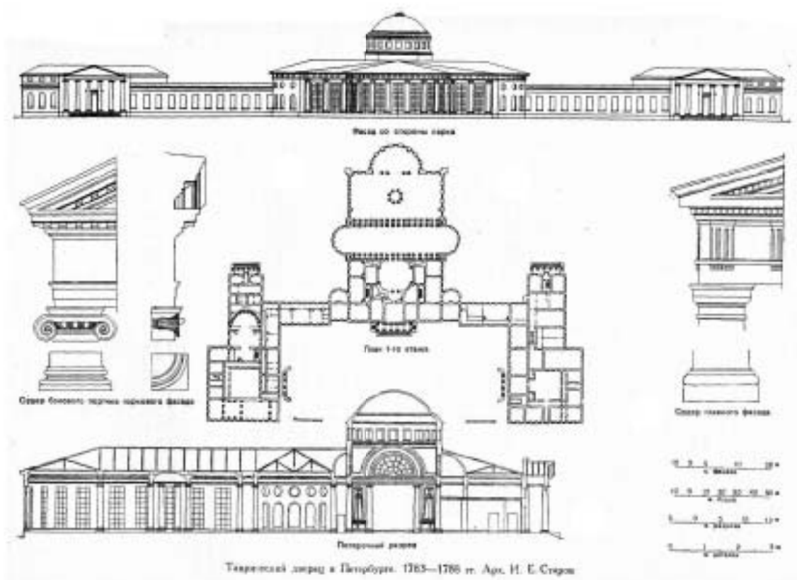
9. Таврический дворец в Санкт-Петербурге. Арх. И.Е. Старов. Главный фасад, план первого этажа, поперечный разрез, детали.
