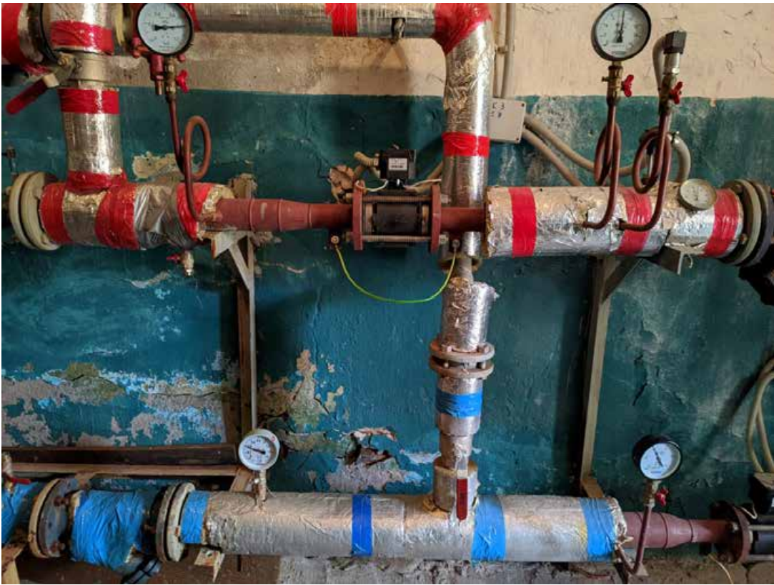
Фото 2. ИТП в помещении 17-Н в здании по адресу: г. Санкт-Петербург, 4-я линия, 35-37
