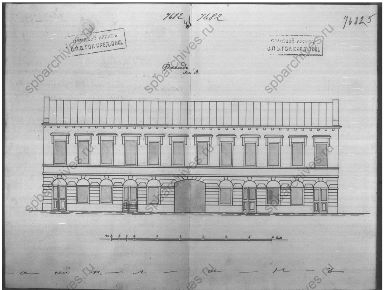
Илл. 15. Фасад дома В.Д. Залемана по 4-й линии, лит. А. 1904 г. ЦГИА СПб. Ф. 515. Оп. 4. Д. 2707. Л. 4-5.
