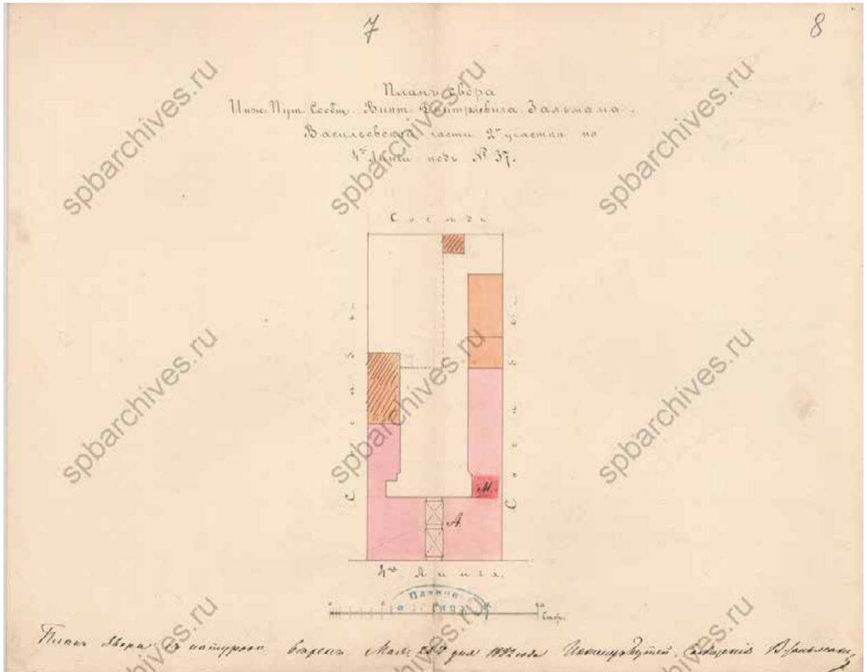
Илл. 13. План двора инженера путей сообщения Виктора Дмитриевича Зальмана Васильевской части 2-го участка по 4-й линии под № 37. 1882 г. ЦГИА СПб. Ф. 513. Оп. 102. Д. 1554. Л. 7-8.
