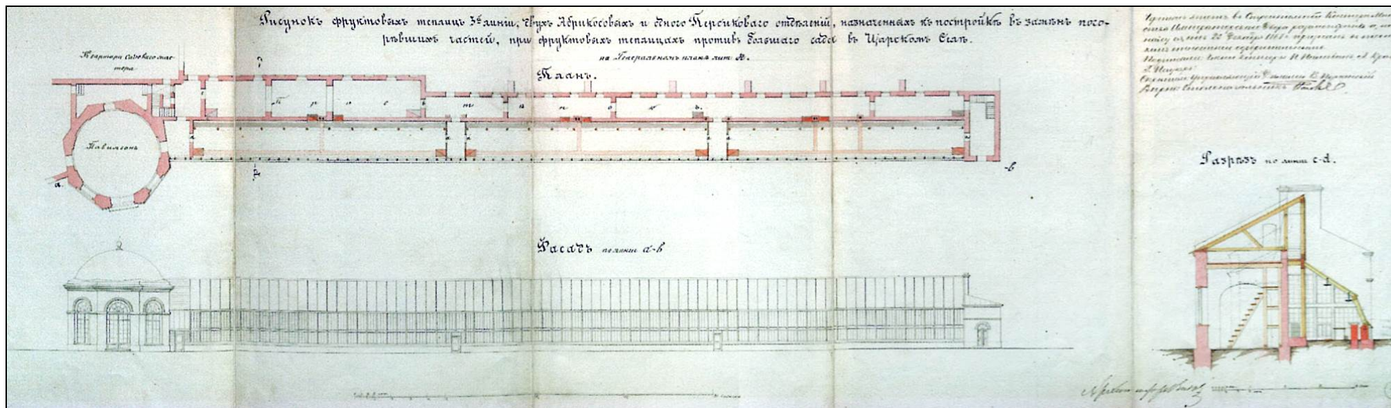
Илл. 8. 3-я линия фруктовых теплиц. План, фасад и разрез восточной части. Проект восстановления после пожара 1868 г. 3-х отделений: Двух Абрикосовых и одного Персикового. Арх. А.Ф.Видов. ЕД-1017.
