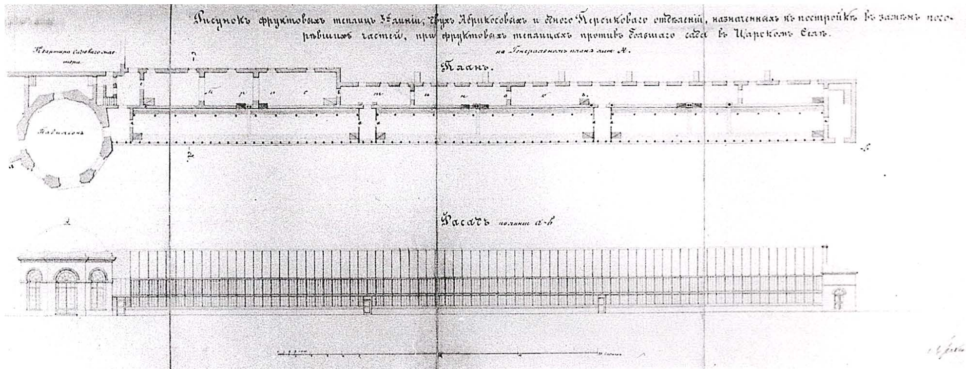
Илл. 10. 3-я линия фруктовых теплиц. План и южный фасад восточной половины 3-й линии: двух Абрикосовых и одного Персикового, назначенных к постройке взамен сгоревших. 1868 г. Арх. А.Ф.Видов. ЕД-1017.
