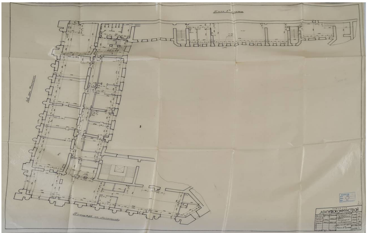
22. Типография им. Володарского. План 3-го этажа. Разрез. 1955. ЦГАНТД. Ф. 46. Оп. 3-8. Д. 36.
