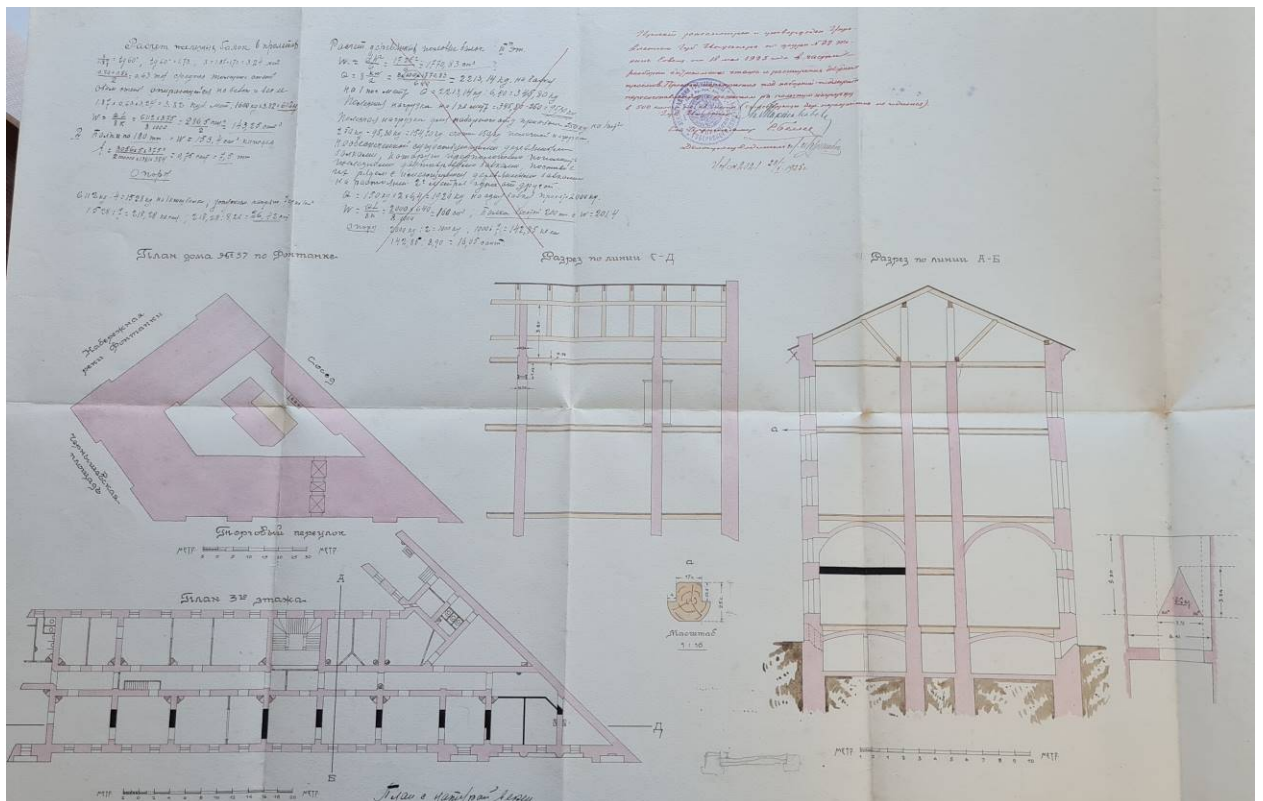
20. К проекту перепланировки части здания бывш. МВД. 1925. ЦГАНТД. Ф. 192. Оп. 3-1. Д. 265.
