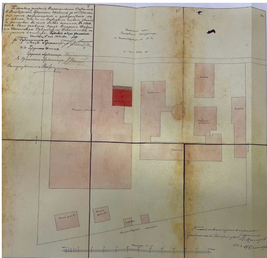
15. Генеральный план Петровкой бумагопрядильной и ткацкой мануфактуры с показанием нового машинного здания. 1913 г. Гр. Инж. П.Макаров. ЦГИА СПб, ф. 256, оп. 31, д. 602
