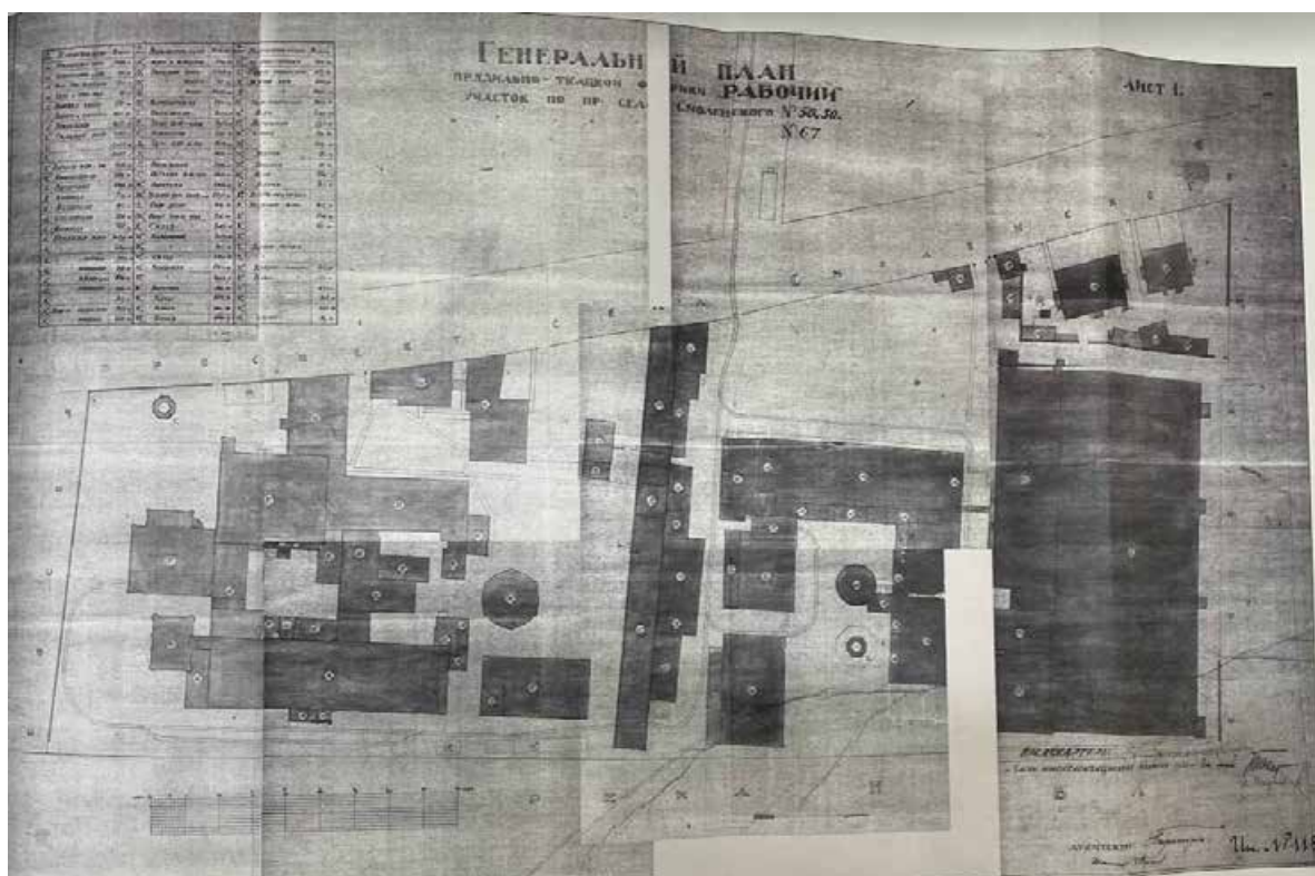
17. Генеральный план прядельно-ткацкой фабрики «Рабочий». 1925 г. ЦГАНТД СПб ф. Р-192, оп. 3-1, д. 3975
