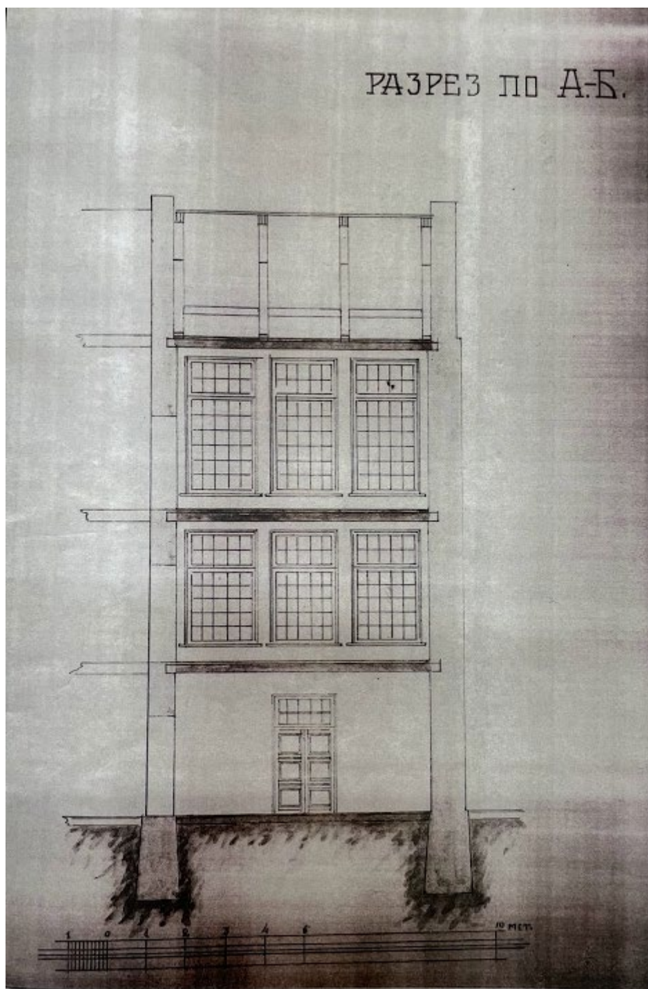
20. Проект постройки Продевального отделения фабрики №2 (Петровской): разрез. 1928 г. ЦГАНТД СПб, Ф. Р-192, оп. 3-1, д. 1413
