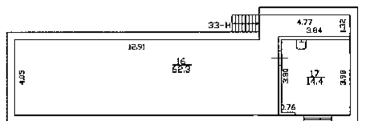
План антресоли
