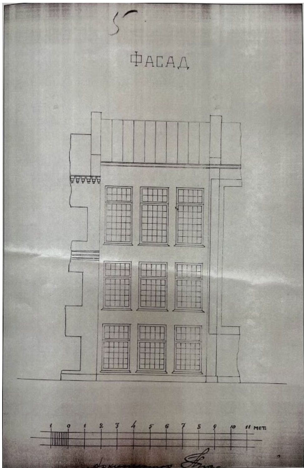
19. Проект постройки Продевального отделения фабрики №2 (Петровской): фасад. 1928 г. ЦГАНТД СПб, Ф. Р-192, оп. 3-1, д. 1413
