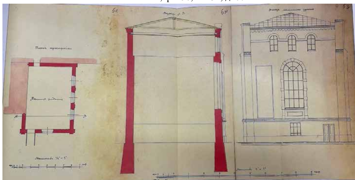
16. План машинного отделения, разрез по А-В, фасад машинного здания Петровской бумагопрядильной и ткацкой мануфактуры. 1913 г. Гр. Инж. П.Макаров. ЦГИА СПб, ф. 256, оп. 31, д. 602
