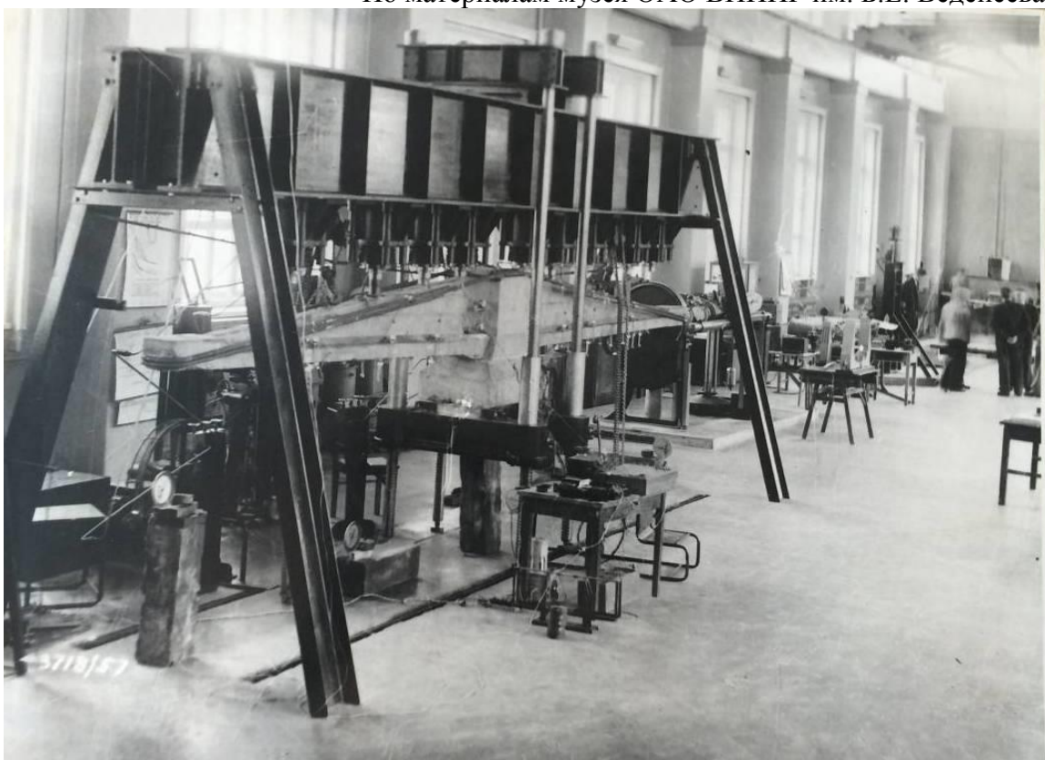
62. Испытание моделей подпорных стен. 1960-е гг. По материалам музея ОАО ВНИИГ им. Б.Е. Веденеева.
