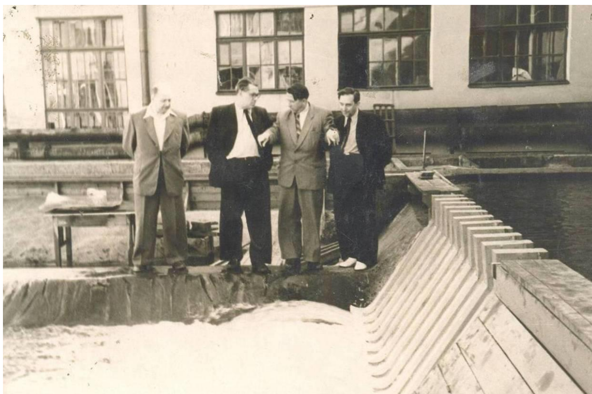
56. Проверка работы Братской ГЭС по модели. Фото 1954 гг. По материалам музея ОАО ВНИИГ им. Б.Е. Веденеева.
