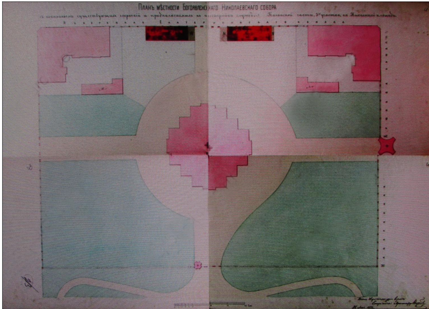
Ил. 17. План местности Богоявленского Николаевского собора с указанием существующих строений и предполагаемых к постройке служб Казанской части 3-го участка на Николаевской площади. 1875 г.
