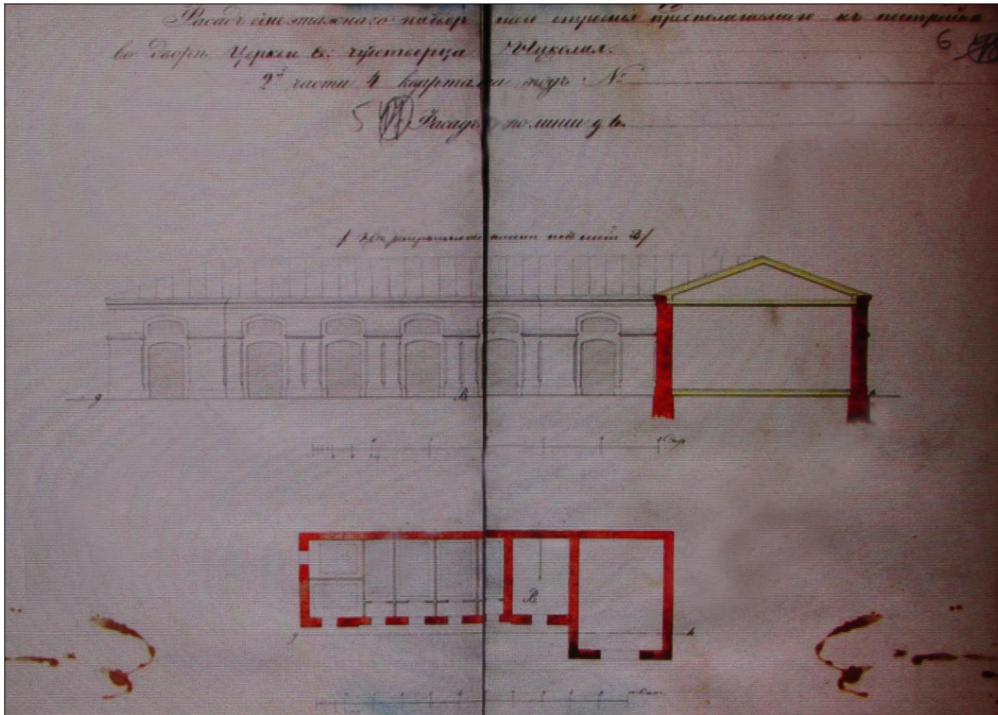
Ил. 14. Фасад одноэтажного надворного строения, предполагаемого к постройке во дворе церкви св. Николая Чудотворца 2-й части 4-го квартала. Арх. Карпов. 1861 г. ЦГИА СПб. Ф. 513. Оп. 102. Д. 3256 А . Л. 5 – 6.
