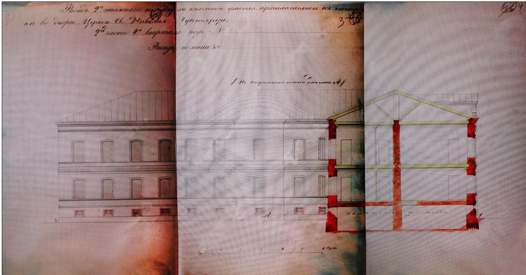
Ил. 13. Фасад двухэтажного каменного флигеля, предполагаемого к постройке во дворе церкви св. Николая Чудотворца 2-й части 4-го квартала. Арх. Карпов. 1861 г. ЦГИА СПб. Ф. 513. Оп. 102. Д. 3256 А . Л. 2 – 4.
