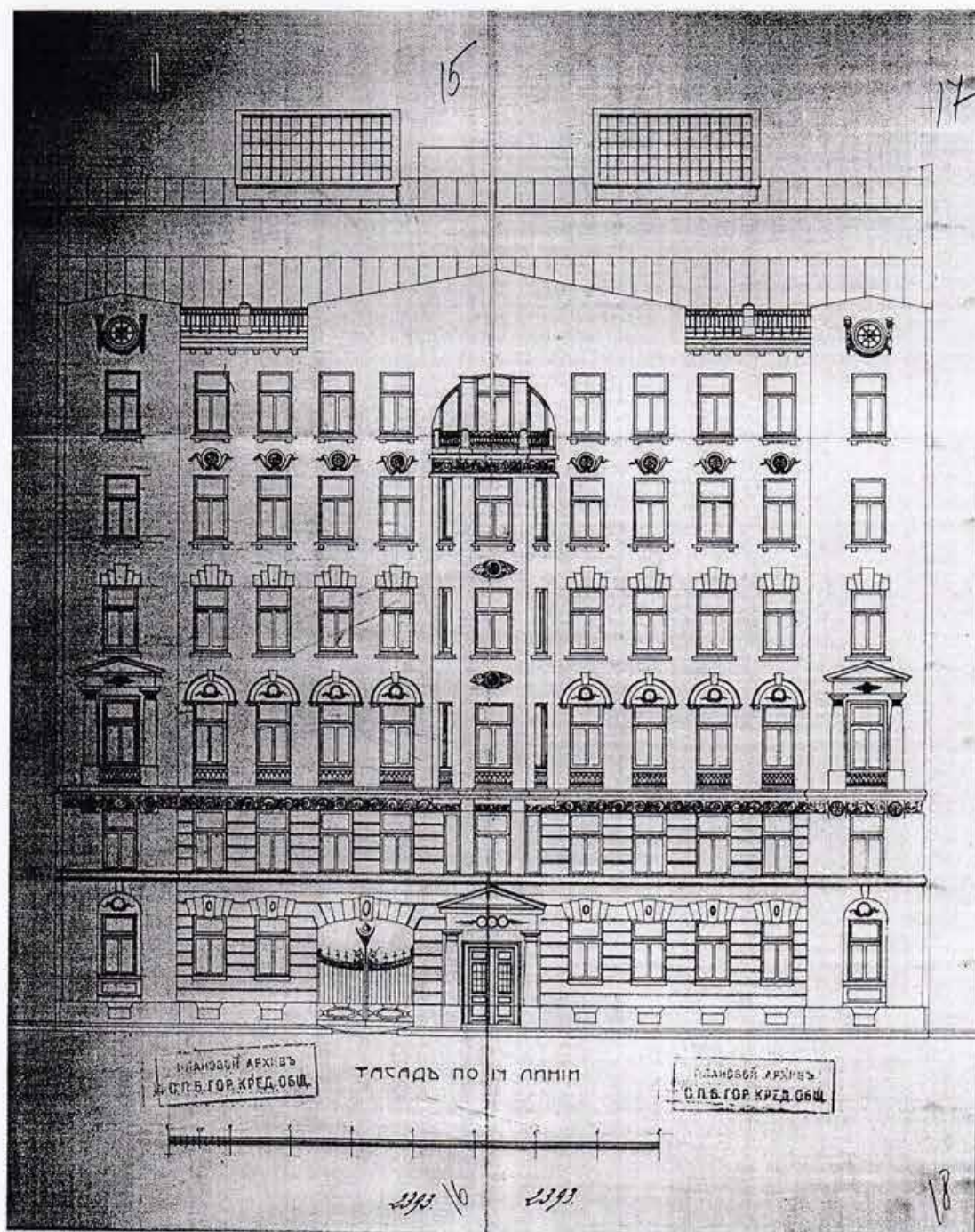
Илл.7. Лицевой фасад доходного дома Е.М.Семеновой. Фиксационный чертеж. 1912 г. ЦГИА СПб. Ф.515.Оп 4.Д.2908.Л.15-18.
