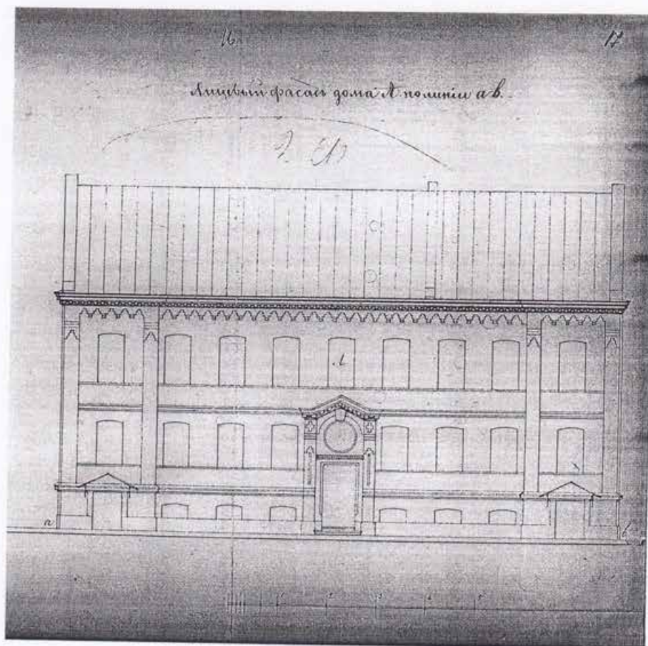
Илл.2. Лицевой фасад дома А (на участке К.К.Циглера). Ныне д. 31-33, лит.О по 14 линии В.О. ЦГИА СПб.Ф.513 Оп.102, Д.1866 .Л.16-17.
