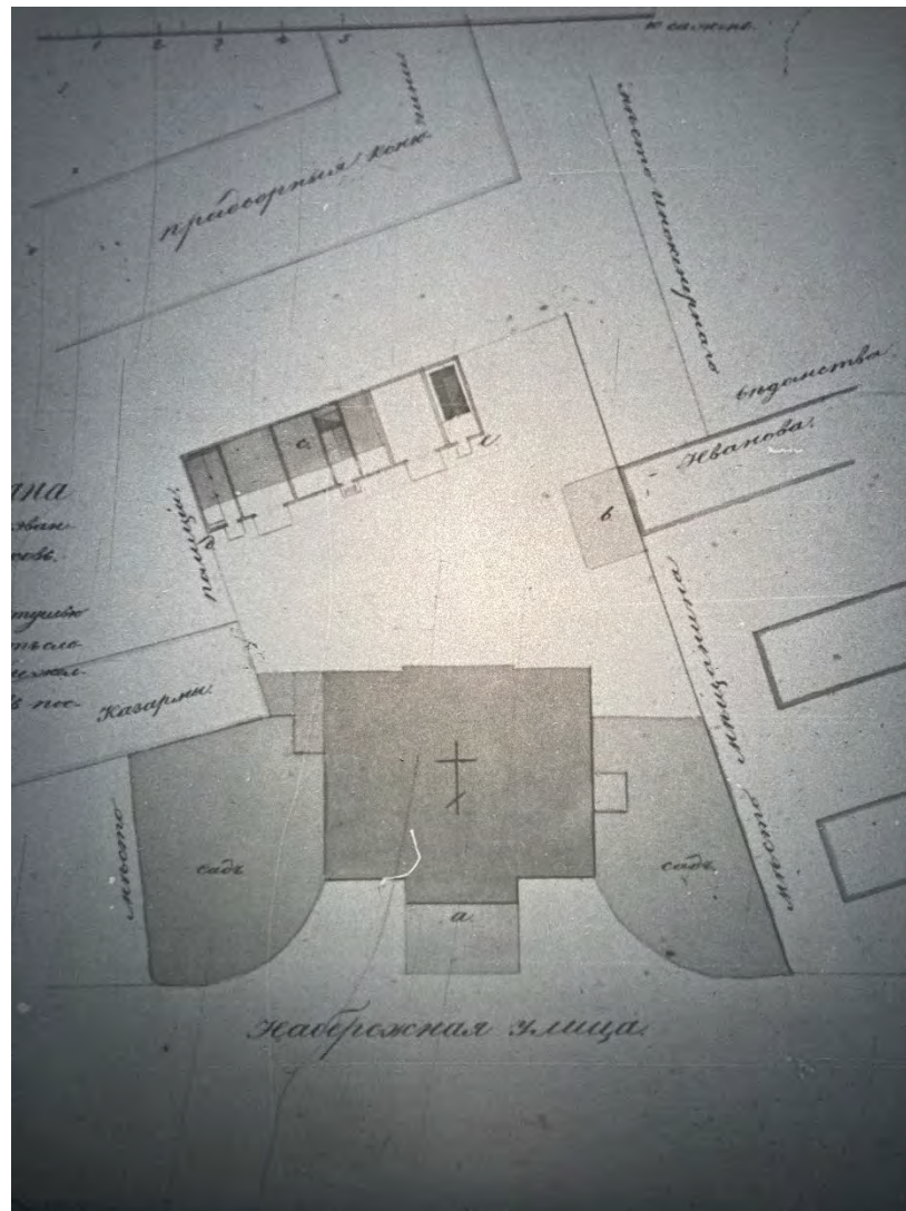
Иллюстрация 21. Фасад и план по которому желает Совет Царскосельской Евангелической Церкви построить службы с мезонином на месте под № 99. 1835 г. РГИА.
