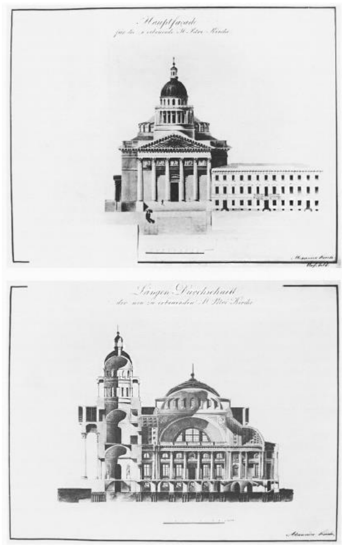
Илл. 3. Конкурсный проект здания церкви св. ап. Петра. Арх. А.Ф. Крих. 1832.
