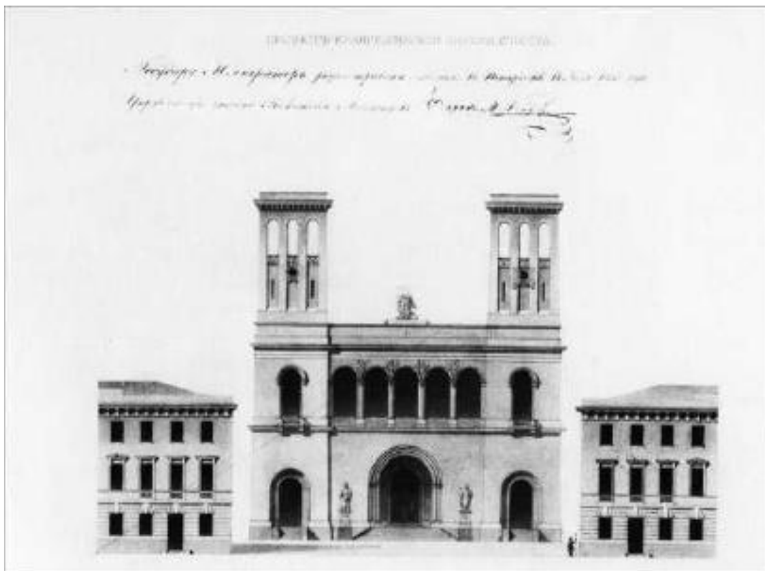
Илл. 4. Проект фасада церкви св. ап. Петра с фрагментами домов по Невскому проспекту. Арх. А.П. Брюллов. 1833.
