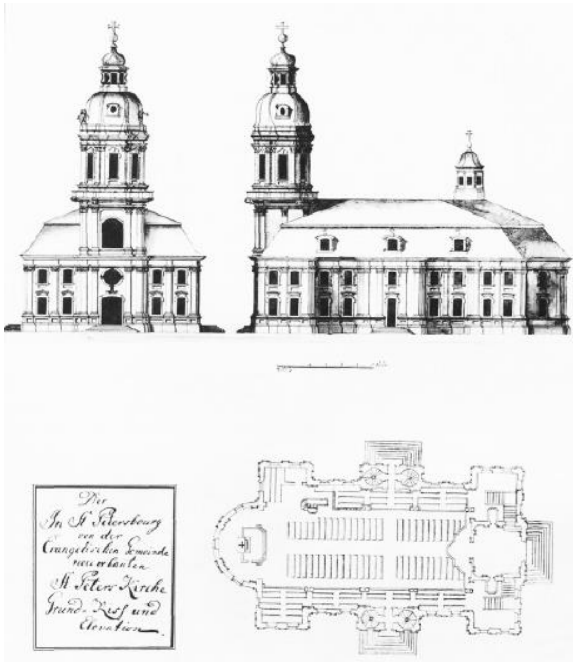
Илл. 1. Здание первой лютеранской церкви св. Петра на Невском проспекте. Фасады и план. 1710-е гг.
