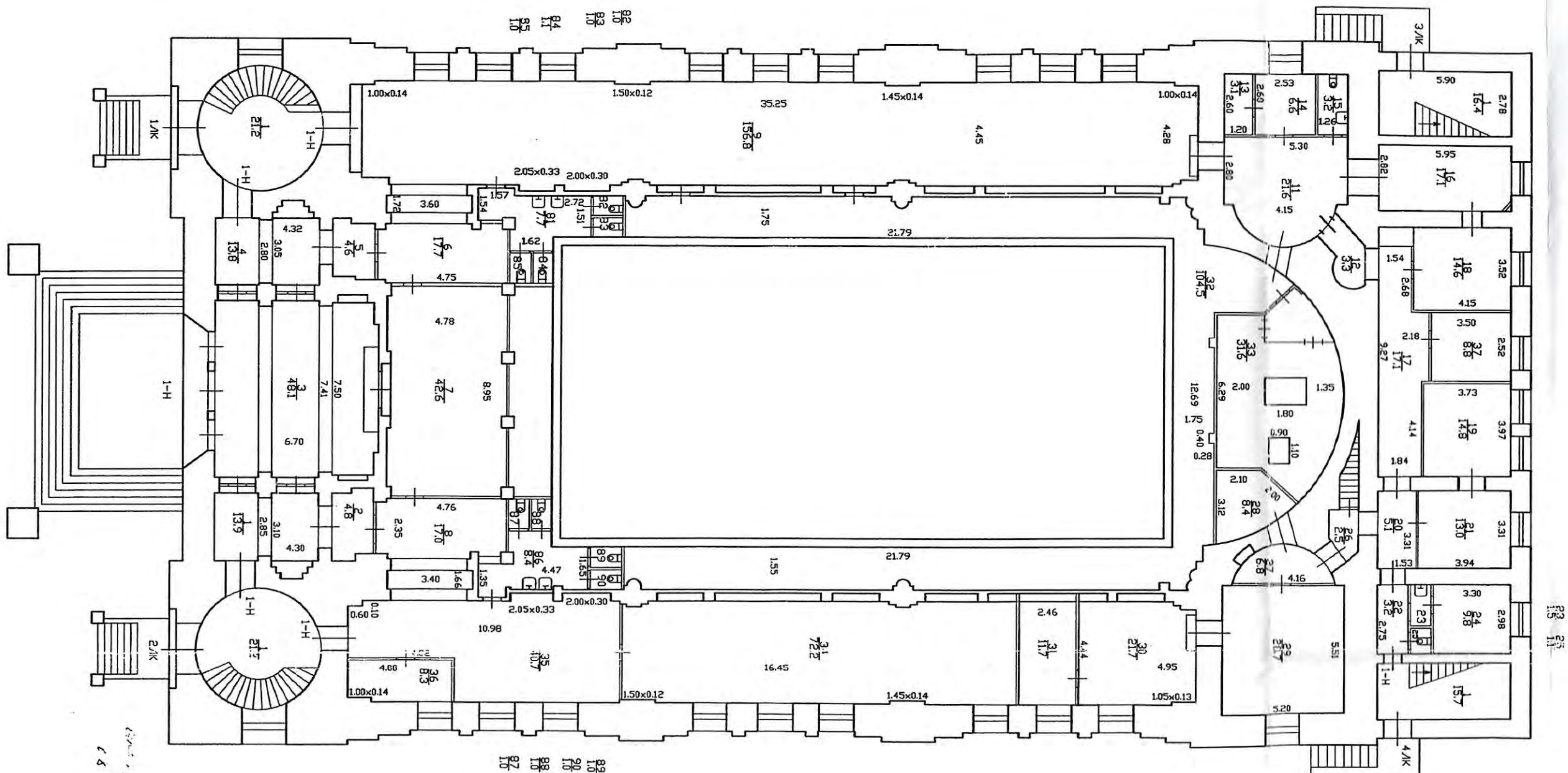
План 1 этажа
