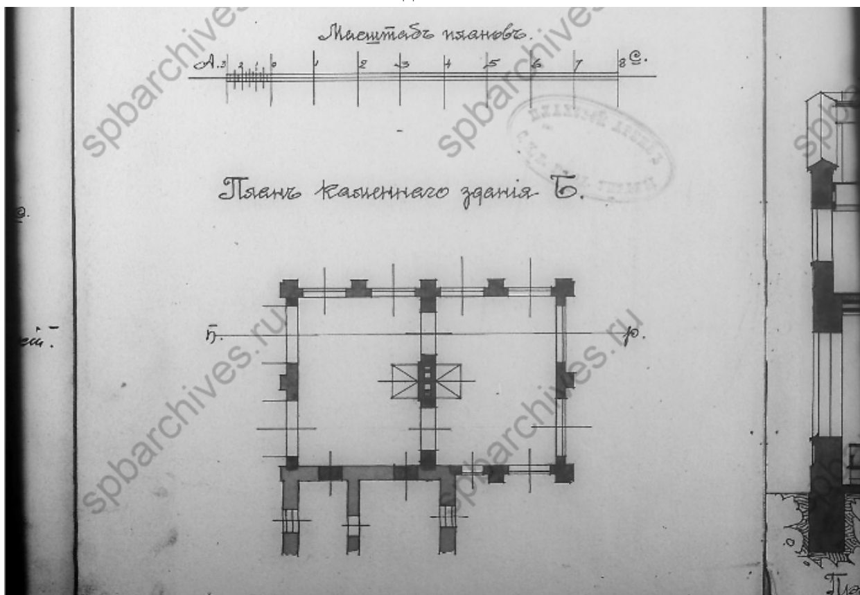
10. План каменного здания. Б. Проект от 17.05.1902 г. — ЦГИА СПб ф.513 оп.102 д.9088.
