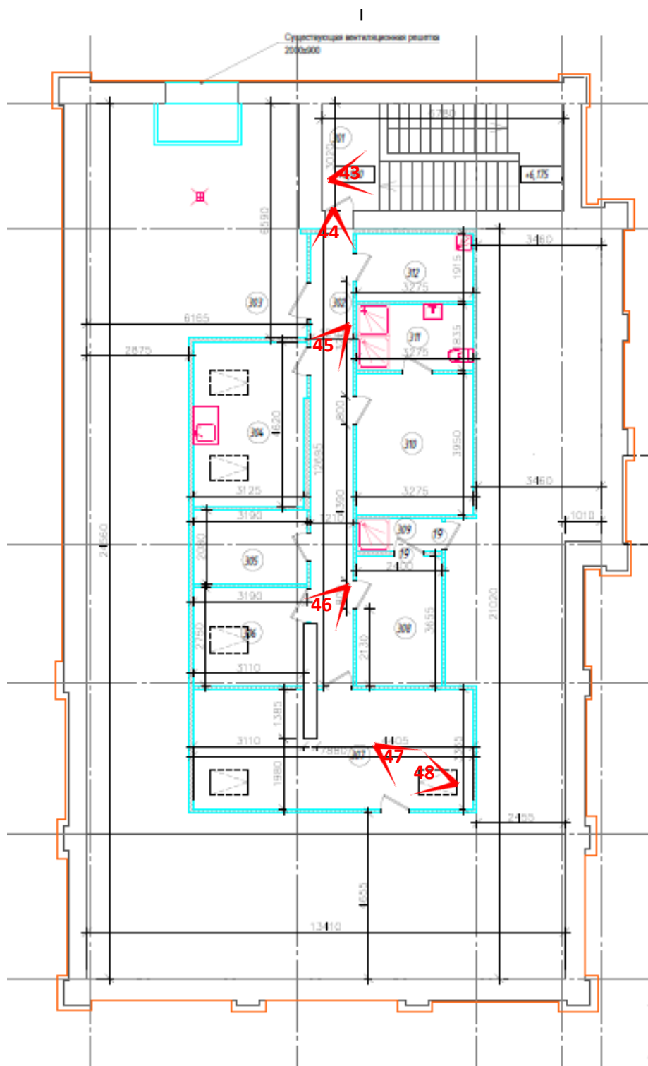
Рисунок 4. Схема фотофиксации на плане мансардного этажа
