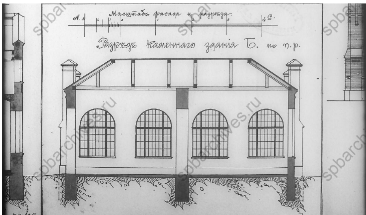
11. Разрез каменного здания. Б. Проект от 17.05.1902 г. — ЦГИА СПб ф.513 оп.102 д.9088.
