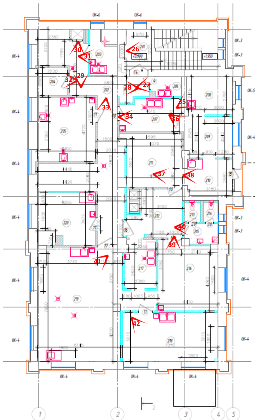
Рисунок 3. Схема фотофиксации на обмерном плане 2 этажа
