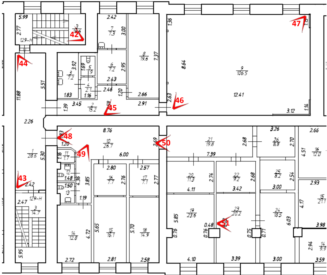
Рисунок 5. Схема фотофиксации на фрагменте плана 2 этажа, пом. 129-Н
