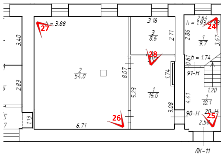
Рисунок 2. Схема фотофиксации на фрагменте плана 1 этажа, пом. 90-Н
