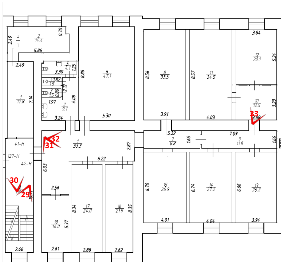
Рисунок 3. Схема фотофиксации на фрагменте плана 2 этажа, пом. 42-Н
