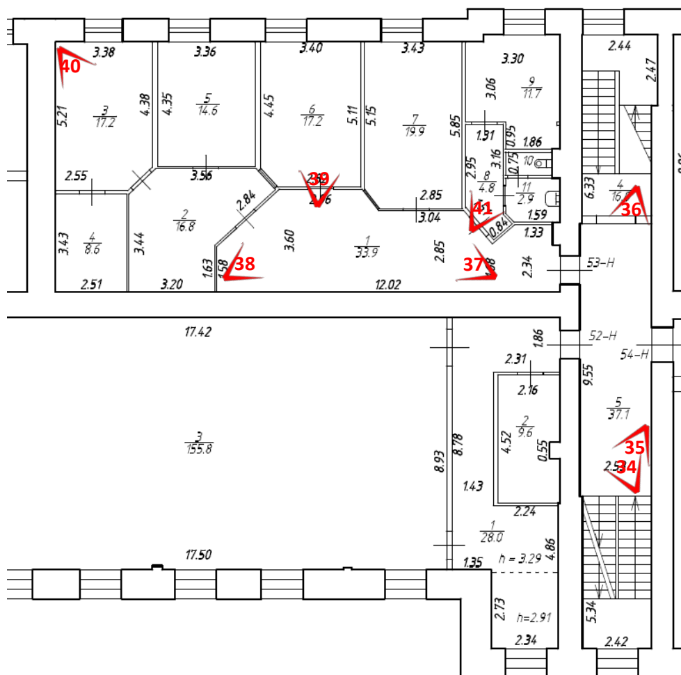
Рисунок 4. Схема фотофиксации на фрагменте плана 2 этажа, пом. 53-Н
