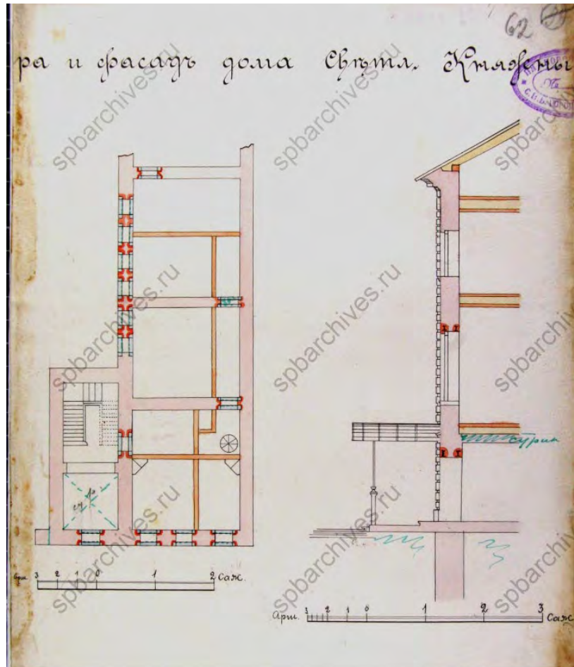
16. Дом княжны М.А. Чернышевой. 1910. ЦГИА СПб. Ф. 513. О. 102. Д. 84.
