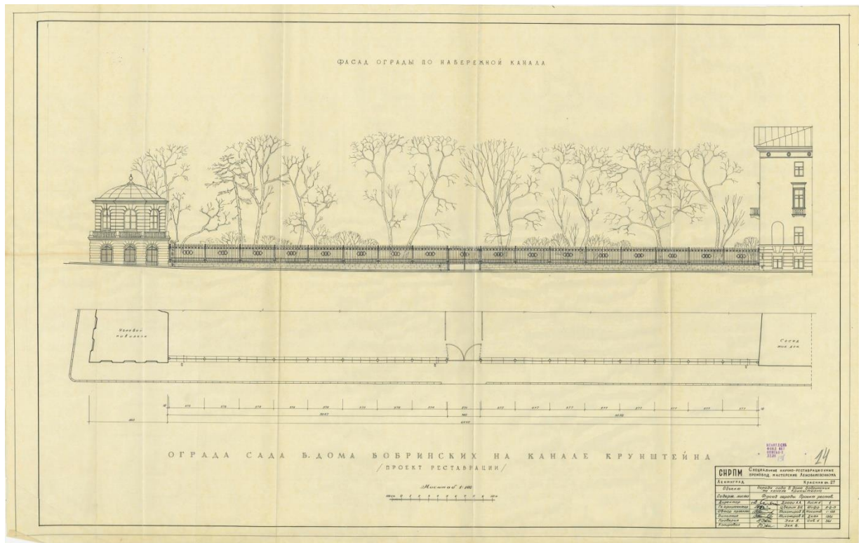
11. Проект реставрации фасада ограды по Адмиралтейской набережной (Крунштейна). 1961 год. Ист.: Архив ЦГАНДТ. Фонд. 467 Описание. 33 Дело.131
