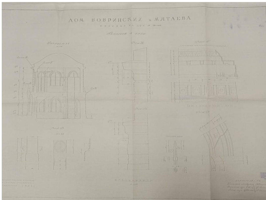
10. Разрезы, элементы фасада Садового павильона. 1946г.
