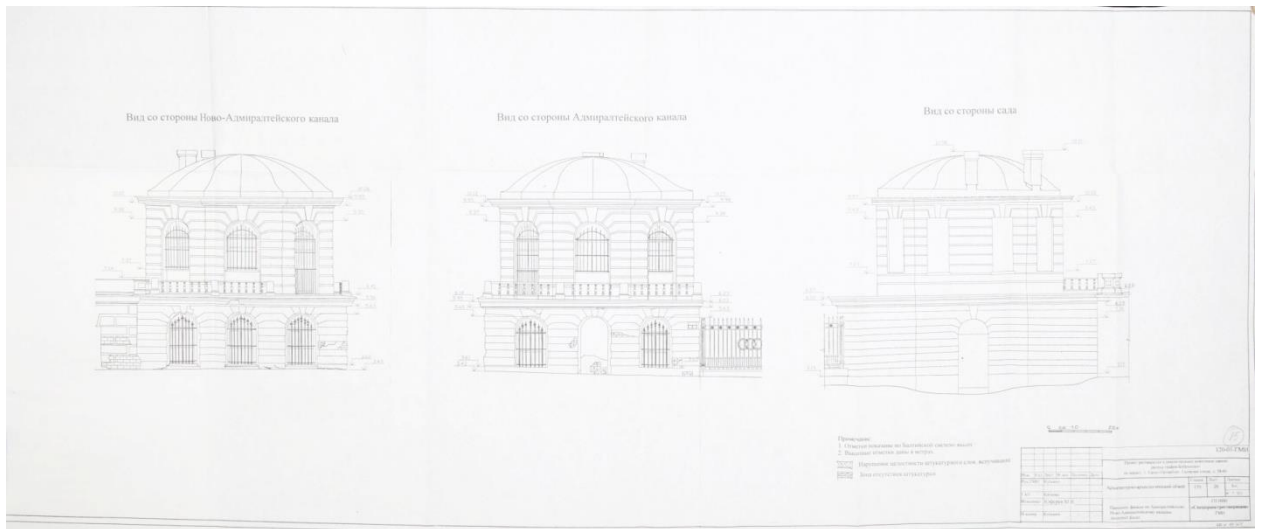
17. Обмерные планы фасадов Садового павильона со стороны Ново-Адмиралтейского, Адмиралтейского каналов и со стороны сада. 2001 год. Ист.: Архив ЦГАНДТ. Фонд. Р.-467 Описание. 33 Дело. 130.
