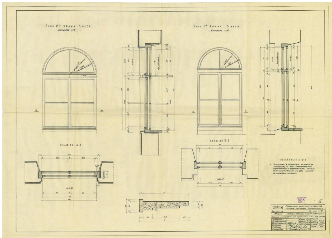
12. Проект реставрации оконных проемов Садового павильона. 1961 год. Ист.: Архив ЦГАНДТ. Фонд. 467 Описание. 33 Дело.131
