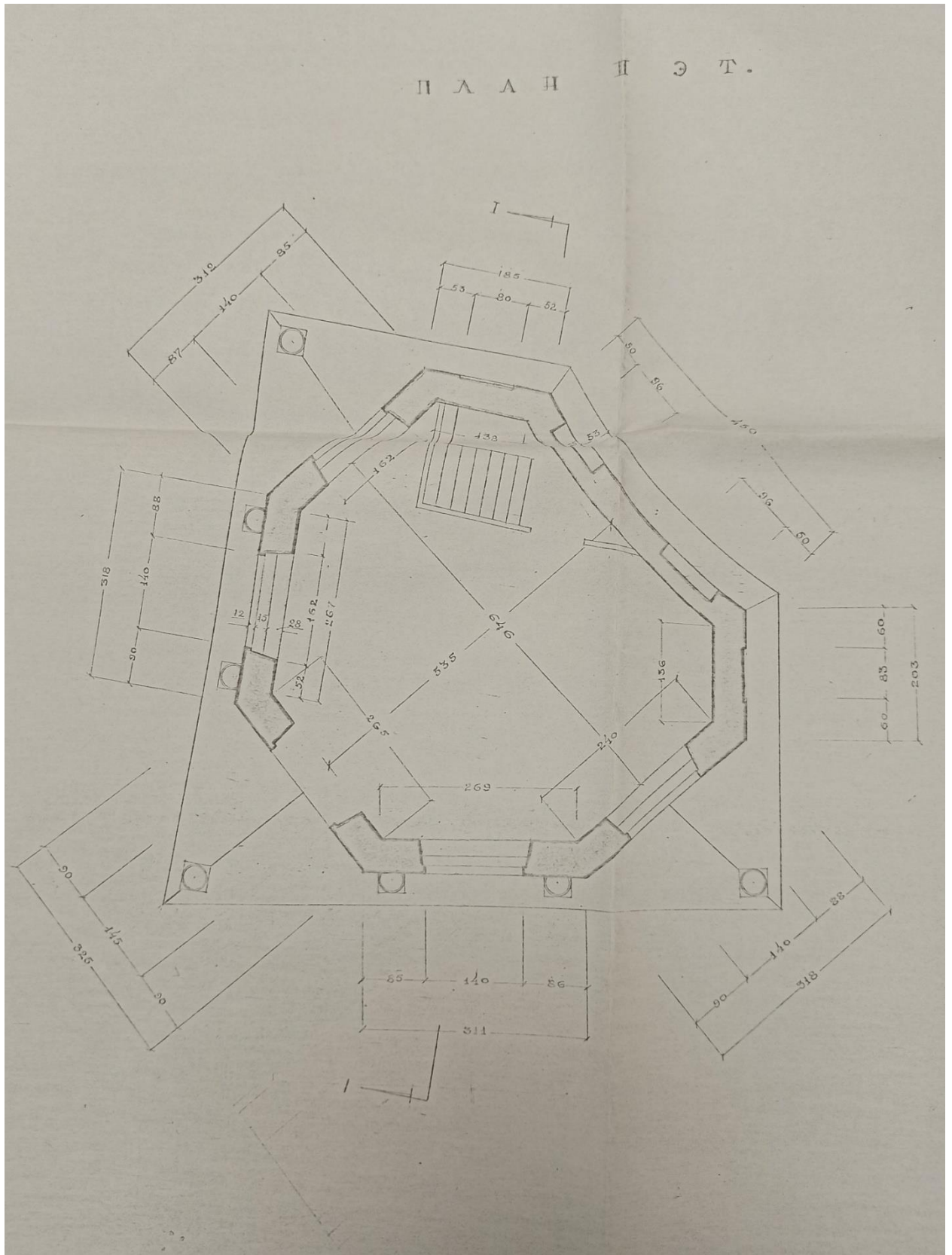
3. Фрагмент обмерного плана. План 2-го этажа. 1946 год. Ист.: Архив ЦГАНДТ. Фонд. Р.-468 Описание. 33 Дело. 128.
