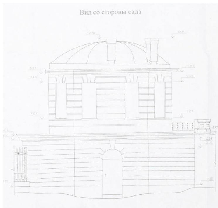
20. Фрагмент обмерного плана фасада Садового павильона со стороны сада. 2001 год. Ист.: Архив ЦГАНДТ. Фонд. Р.-467 Описание. 33 Дело. 130
