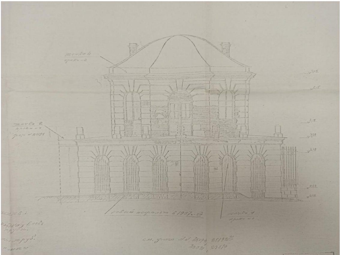
6. Фрагмент обмеров фасада зданий по Ново-Адмиралтейскому каналу. 1946 год.
