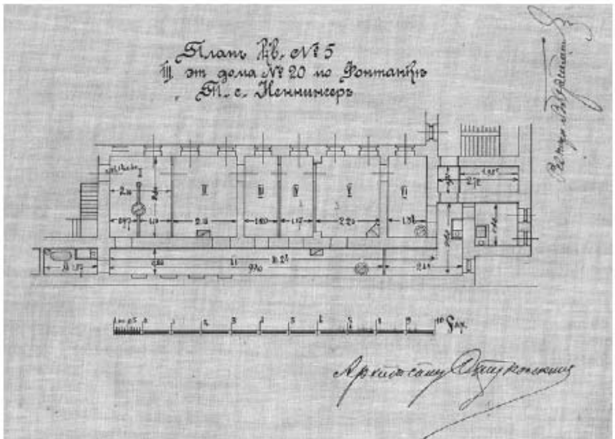
22. План квартиры № 5 III этажа дома № 20 по Фонтанке. Т. С. Ненninger. Арх. Н. Т. Стуколкин. РГИА. Ф. 475. Оп. 2. Д. 158. Л. 24
