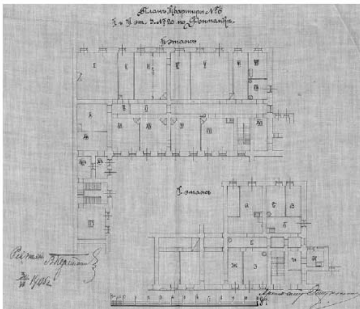
18. План квартиры № 6 I и II эт. д. № 20 по Фонтанке. Арх. Н. Т. Ступолкин. 1905 г. РГИА. Ф. 475. Оп. 2. Д. 158. Л. 15а.
