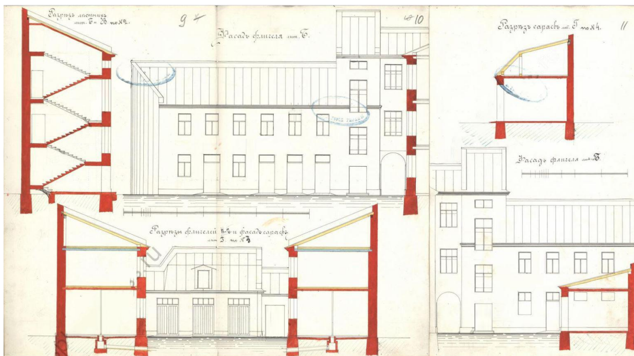
Илл 11. Разрез лестницы лит. Б и В по №2; Фасад флигеля лит. Б; Разрез сарая лит. Г по №4; Разрезы флигелей В и Б и фасад сарая лит. Г по №3; Фасад флигеля лит. Б. ЦГИА СПб, ф.513 оп.102 д.5093
