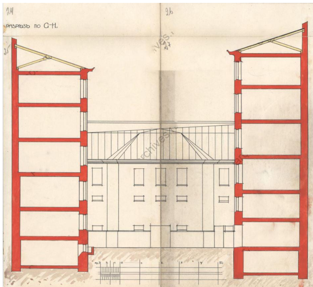
Илл 16. Разрез по G-H. ЦГИА СПб, ф.513 оп.102 д.5093
