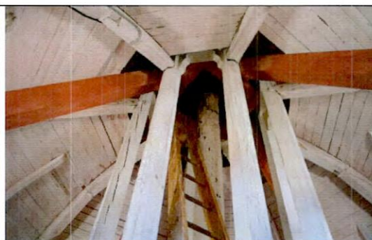
7. Деревянные конструкции купола
