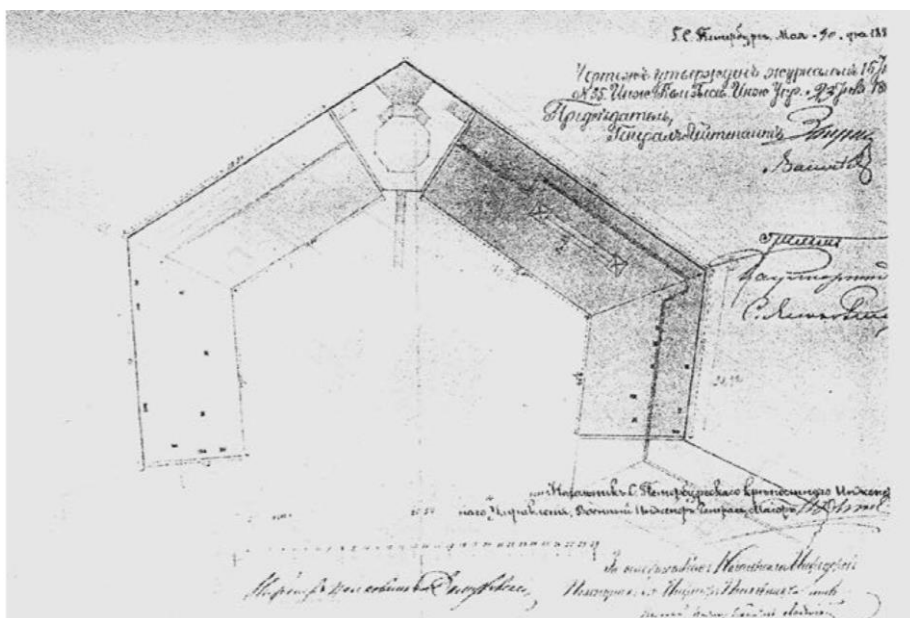
22. План Флажоточной башни. Деталь проектного чертежа по устройству металлического покрытия бастиона Нарышкина. 1887 г. РГА ВМФ. Ф. 3л. Д. 5936.
