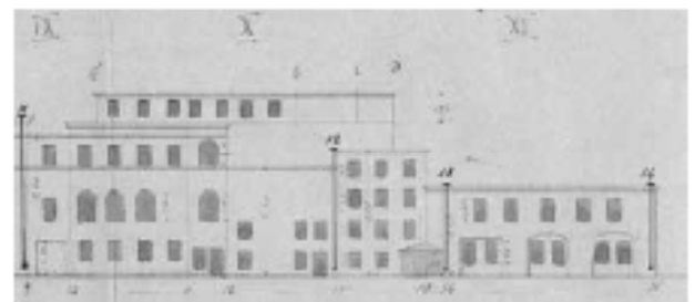
17. Дворовый фасад дома № 20 по набережной р. Фонтанки (развертка). Арх. Н. Т. Стуколкин. 1907 г. РГИА. Ф. 475. Оп. 2. Д. 158. Л. 2. Фрагмент.
