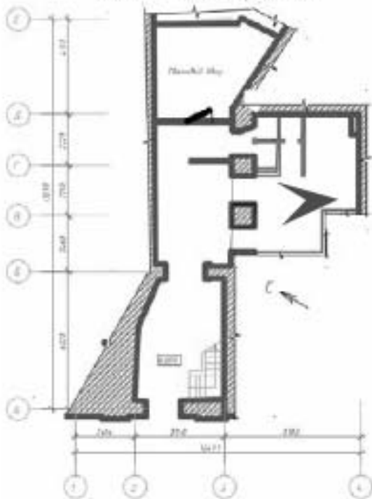
План 1 этажа на олт. 0.000
