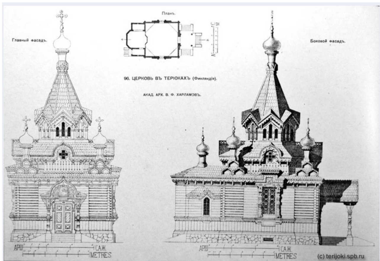
Илл. 2. Деревянная церковь Казанской иконы Божьей Матери в Териоках. Чертежи. // Барановский Г.В. Архитектурная энциклопедия второй половины XIX. Том 1. Арт-Родник, 2006 г.
