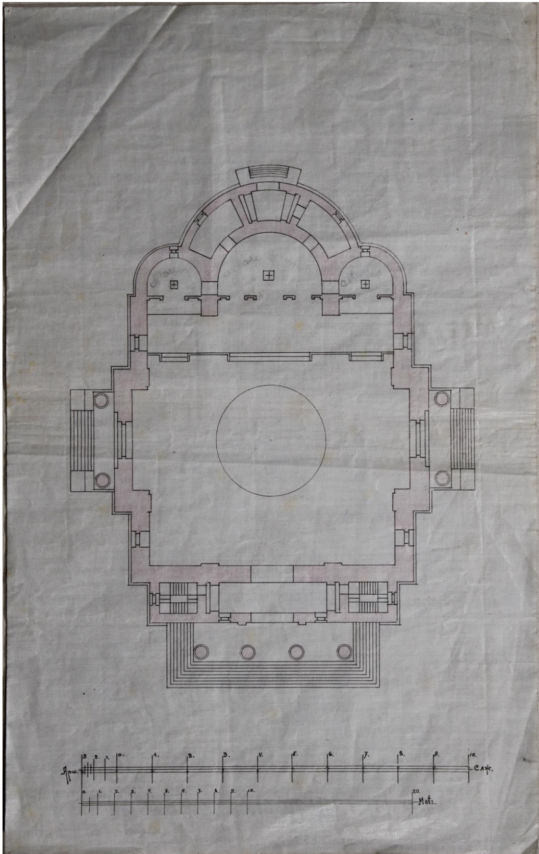
Илл. 3. Церковь Казанской иконы Божьей Матери в Териоках. Чертежи. //Национальный архив Миккели. Шифр: Ja 1
