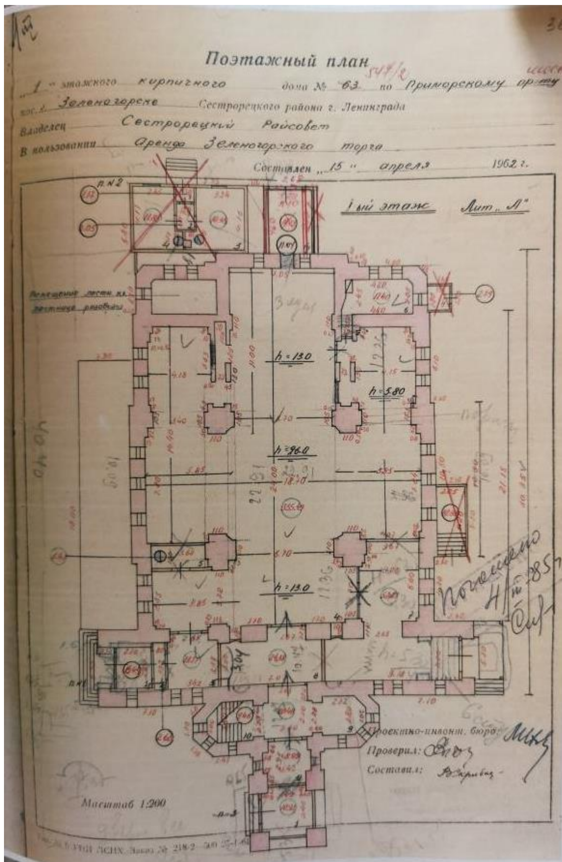
Илл. 12. Поэтажный план дома №63 (547/2) по Приморскому пр. (шоссе) г. Зеленогорск. 1-й этаж. 15 апреля 1962 г.//Архив ПИБ ГУИОН «Северное».
