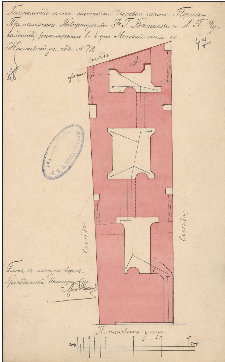
Илл. 10. Генеральный план застройки дворового места Торгово-промышленного товарищества Ф.Г. Бажанова и А.П. Чуваждиной, расположенного в 4-м участке Московской части по Николаевской ул. под № 72. 1907 г. ЦГИА СПб. Ф. 513. Оп. 102. Д. 5093. Л. 47.
