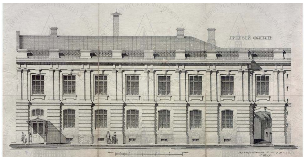
Илл. 9. Лицевой фасад нового здания (флигеля) в Таможенном переулке. СПФ АРАН Ф.4. Оп.22. Д.15. Л.3. Справа внизу подпись: «Архитектор Р.Р. Марфельд. 22.XI.1887».
