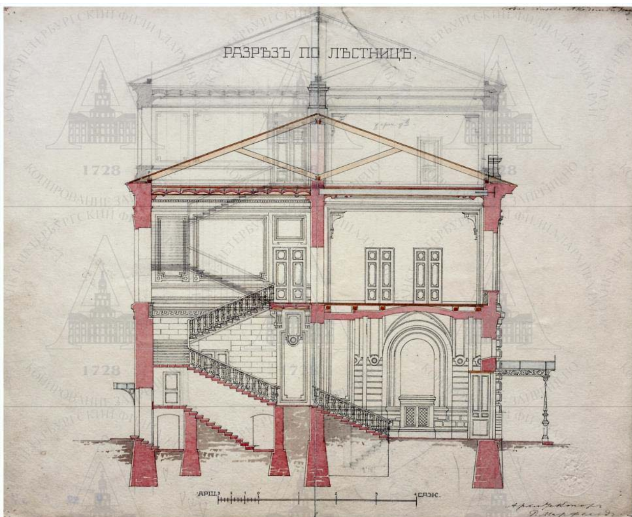
Илл. 10. Разрез по лестнице нового здания в Таможенном переулке. 1900-е гг. СПФ АРАН. Ф.4. Оп.22. Д.15. Л.4.
