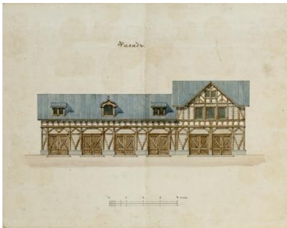
Илл. 14. Чертеж. Особняк графа В.В. Гудовича. Службы. Фасад. Проект Данини Сильвио А.// https://goskatalog.ru/ № 3212485. Номер по КП (ГИК): ЦС КП-14564/6. Инвентарный номер: ЕД-1381/6-ХІІІ
