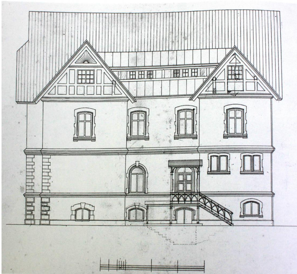
Илл. 10. Особняк В.В. Гудовича. Задний южный фасад (черновой вариант). Эскиз Сильвио Данини. 1900 г.//Козлов А.В. Сильвио Данини. — Санкт-Петербург, Издательский Дом «Коло», 2010
