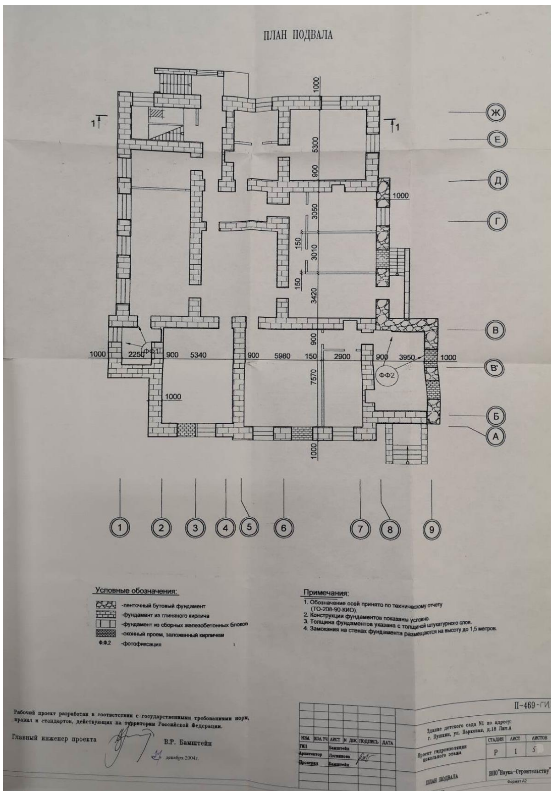
Илл. 9. План подвала здания по ул. Парковая, д.18, лит. А.// Архив КГИОП. п. 226-Г-61. пр.3. «Проект гидроизоляции цокольного этажа здания детского сада №1 по адресу: г. Пушкин, ул. Парковая, д.18, лит. А.». шифр: П-469. СПб. 2004 г.
