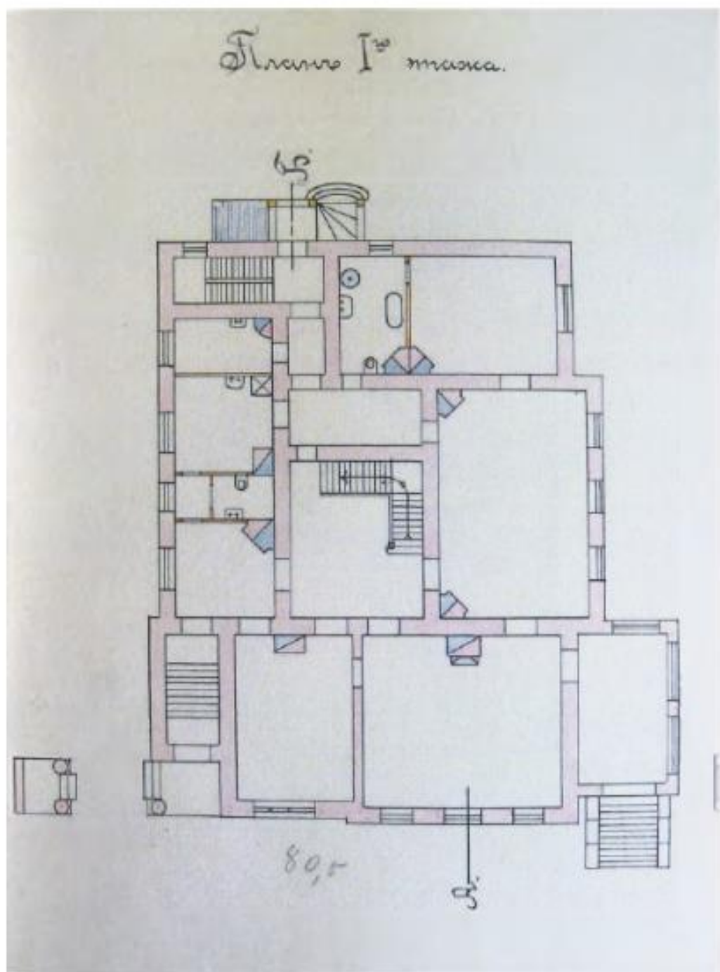
Илл. 5. План первого этажа лит. А. 1910 г. //ЦГИА СПб. Ф.1546. Оп.5. Д.1776. Волконская ул. № 18, Гудович В.В.
