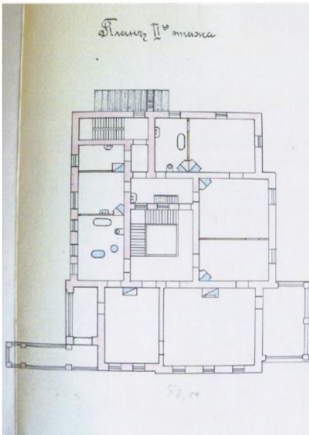
Илл. 6. План второго этажа лит. А. 1910 г. //ЦГИА СПб. Ф.1546. Оп.5. Д.1776. Волконская ул. № 18, Гудович В.В.
