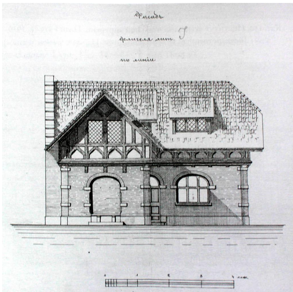
Илл. 12. Особняк В.В. Гудовича. Служебный флигель, фасад. Эскиз Сильвио Данини. 1900 гт./Козлов А.В. Сильвио Данини. — Санкт-Петербург, Издательский Дом «Коло», 2010
