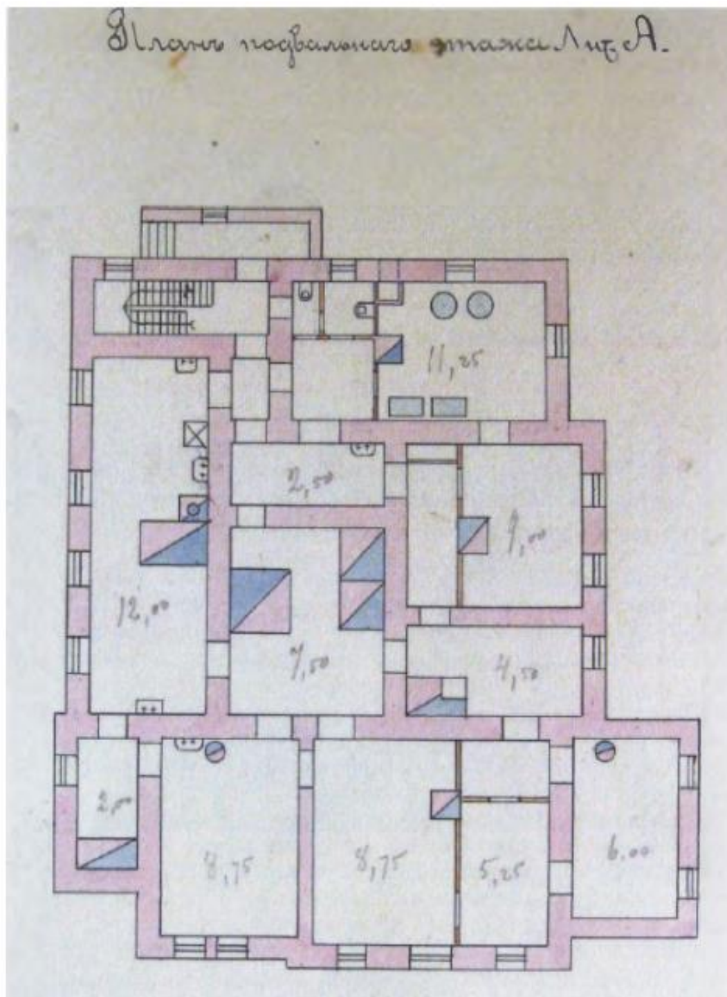
Илл. 4. План подвального этажа лит. А. 1910 г. //ЦГИА СПб. Ф.1546. Оп.5. Д.1776. Волконская ул. № 18, Гудович В.В.
