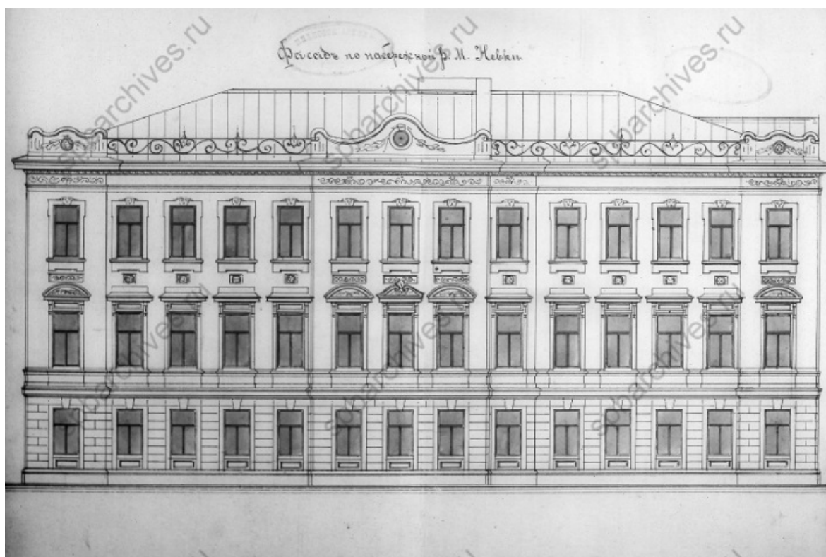
Илл. 10. Объект культурного наследия регионального значения «Особняк-контора и здание библиотеки лесопильного производства Ф.Я. и Н.Я. Колобовых». Чертеж фасада по набережной р. М. Невки Особняка-конторы. ЦГИА СПб. Фонд 513.Опись 102. Дело 8017
