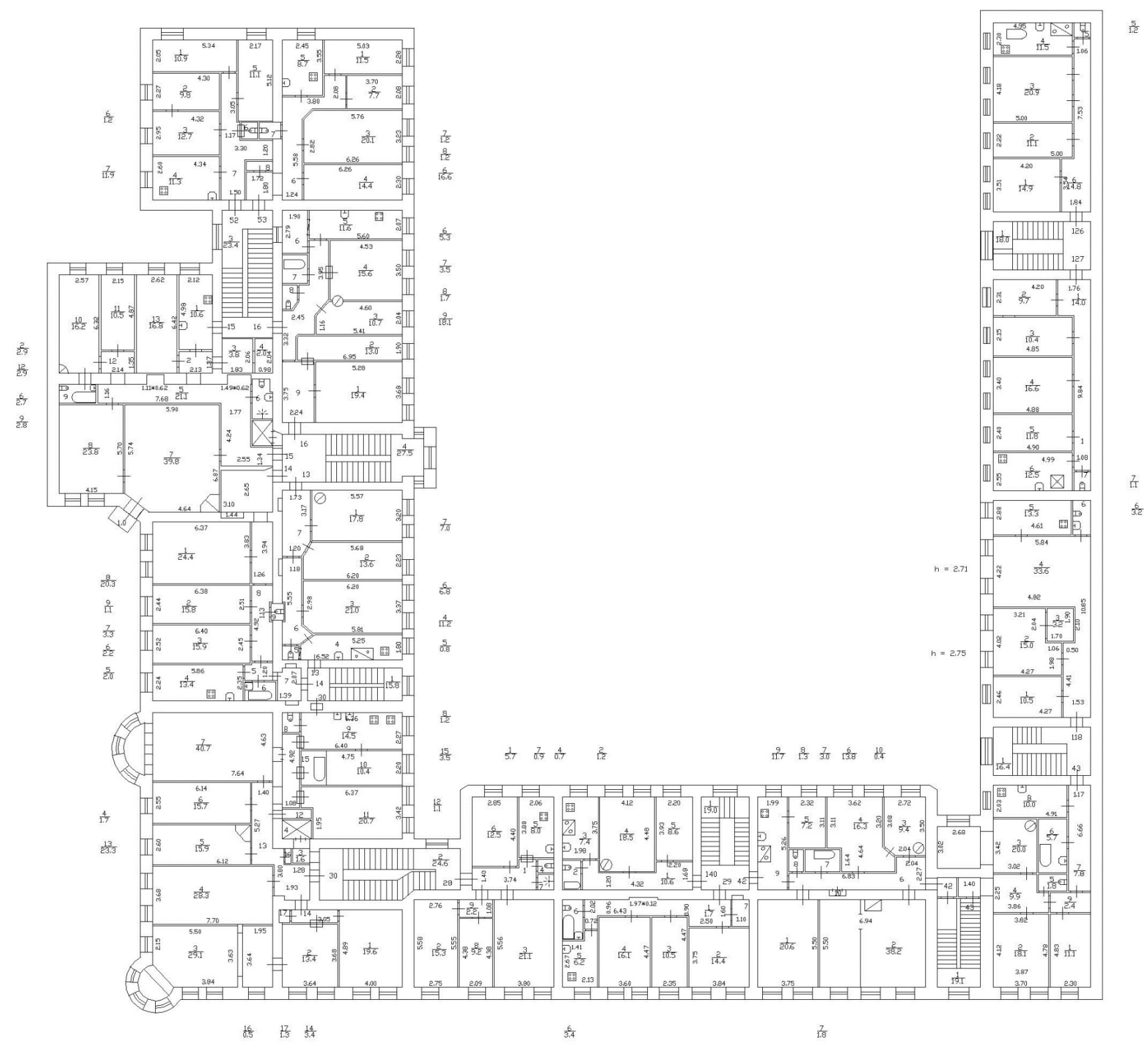
План 4 Этажа
