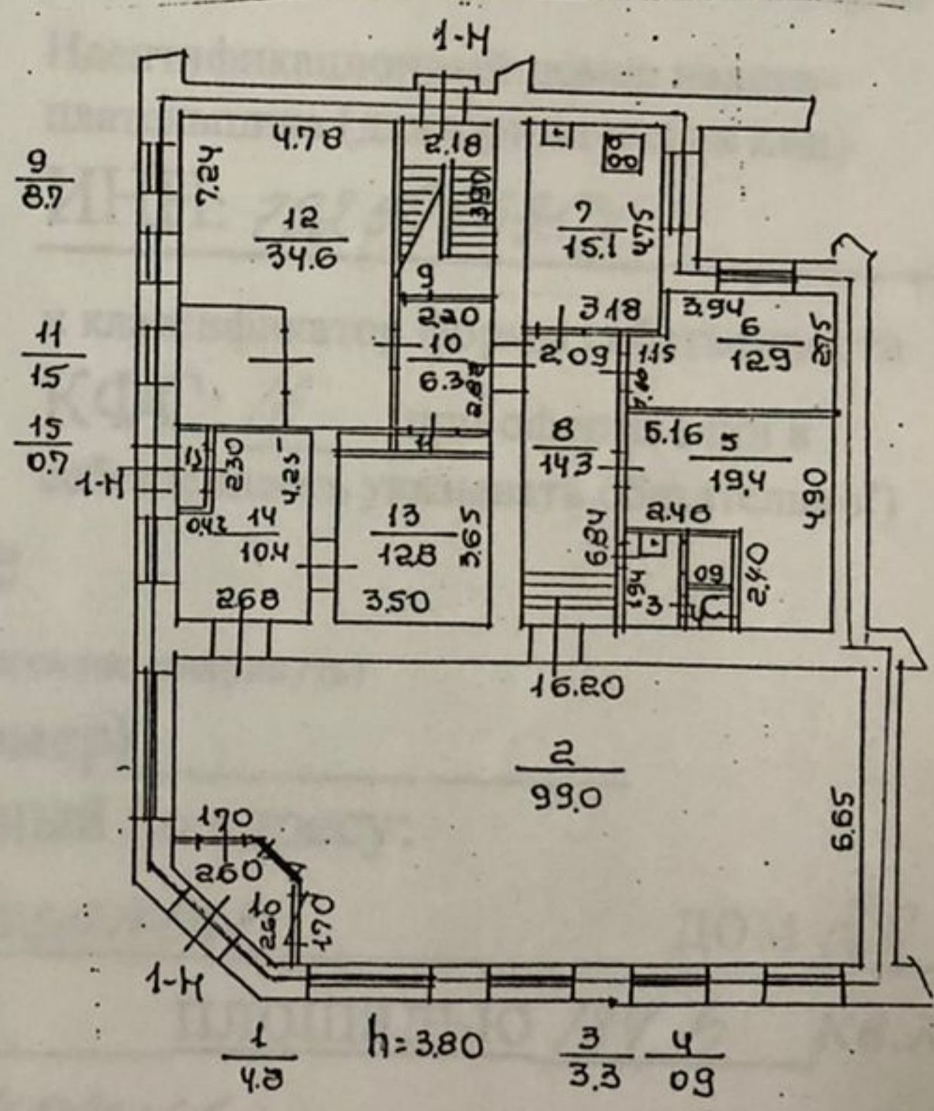
план 1 этажа
