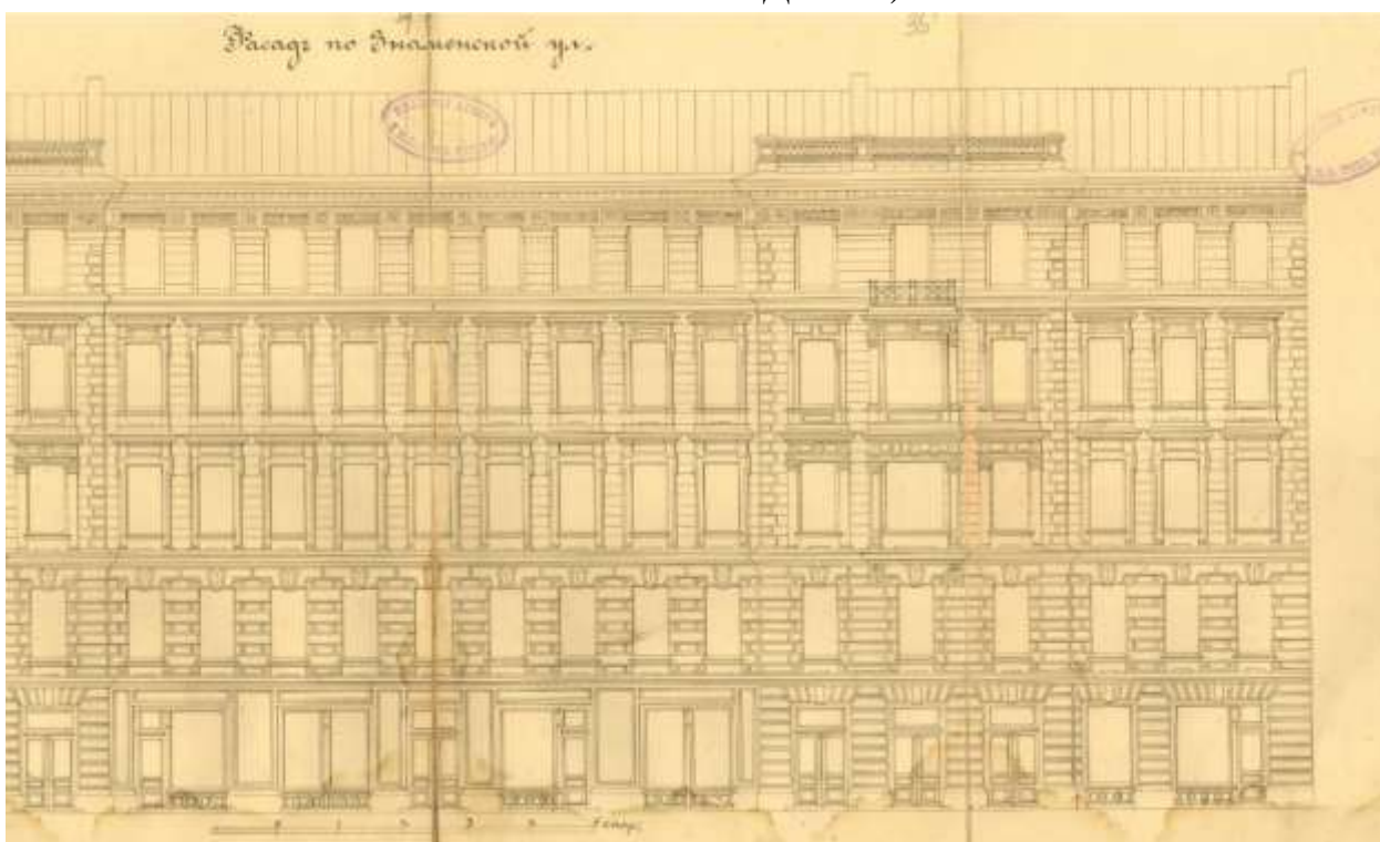
6. Фасад по Знаменской ул. Архитектор А.В. Иванов. 1897 г. (ЦГИА СПб. Ф. 513. Оп. 102. Д. 4061).
