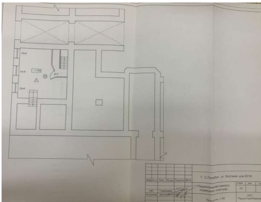
15. План цокольного этажа. Перепланировка нежилого помещения в ресторан. Рабочий проект перепланировки нежилых помещений по адресу: С-Пб, ул. Восстания, д. 20/16, пом. 1-Н под размещение кафе-ресторана. 2003 г. (архив КГИОП П-1500-В).
