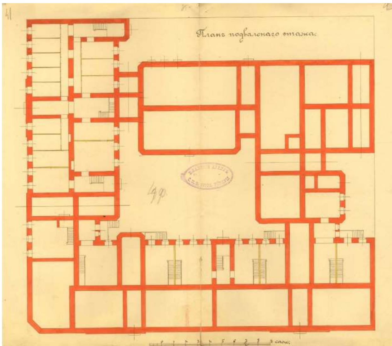
7. План подвального этажа. 1897 г. (ЦГИА СПб. Ф. 513. Оп. 102. Д. 4061).
