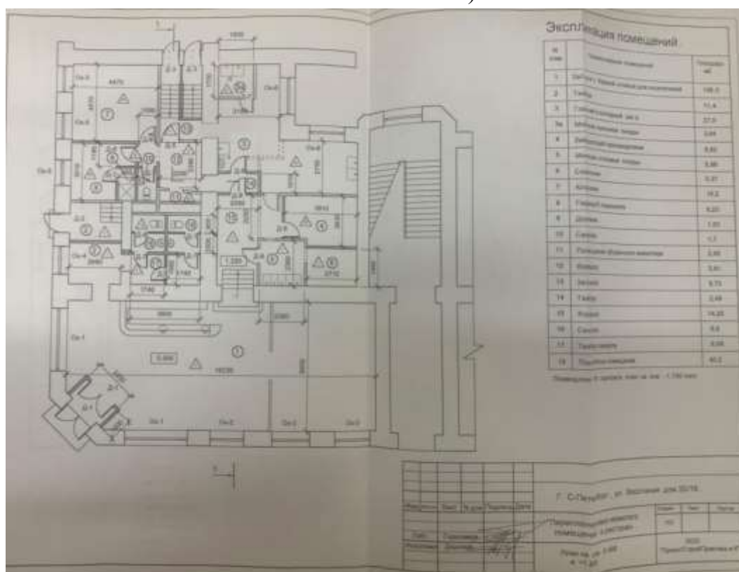
16. План первого этажа. Перепланировка нежилого помещения в ресторан. Рабочий проект перепланировки нежилых помещений по адресу: С-Пб, ул. Восстания, д. 20/16, пом. 1-Н под размещение кафе-ресторана. 2003 г. (архив КГИОП П-1500-В).
