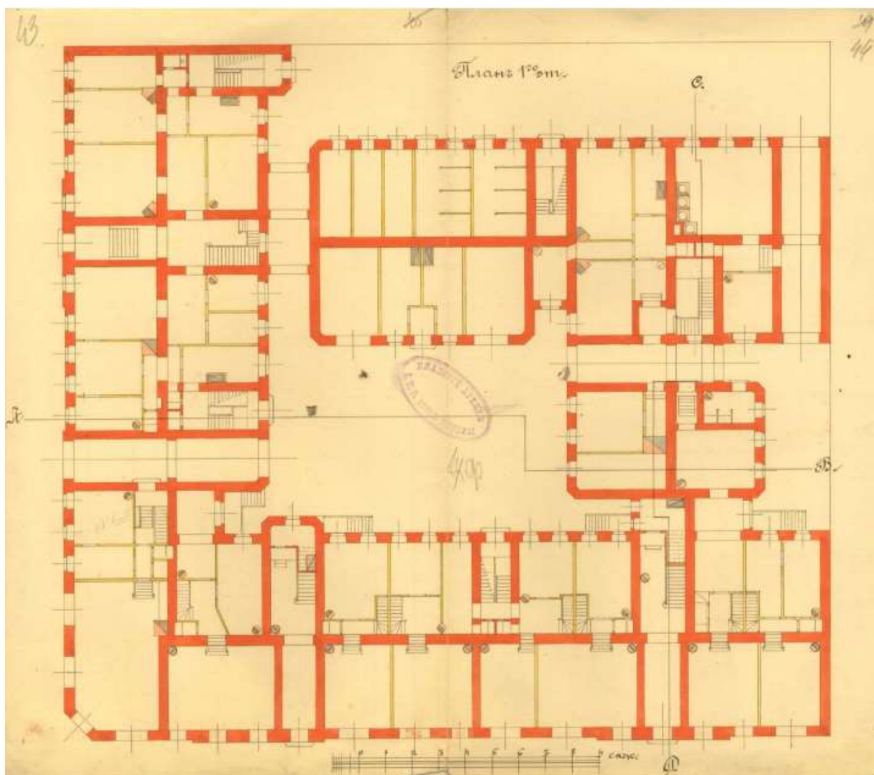
8. План 1-го этажа. 1897 г. (ЦГИА СПб. Ф. 513. Оп. 102. Д. 4061).
