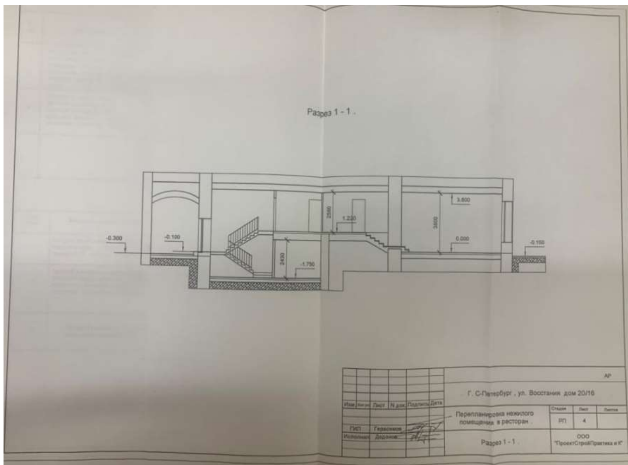
17. Разрез 1-1. Перепланировка нежилого помещения в ресторан. Рабочий проект перепланировки нежилых помещений по адресу: С-Пб, ул. Восстания, д. 20/16, пом. 1-Н под размещение кафе-ресторана. 2003 г. (архив КГИОП П-1500-В).
