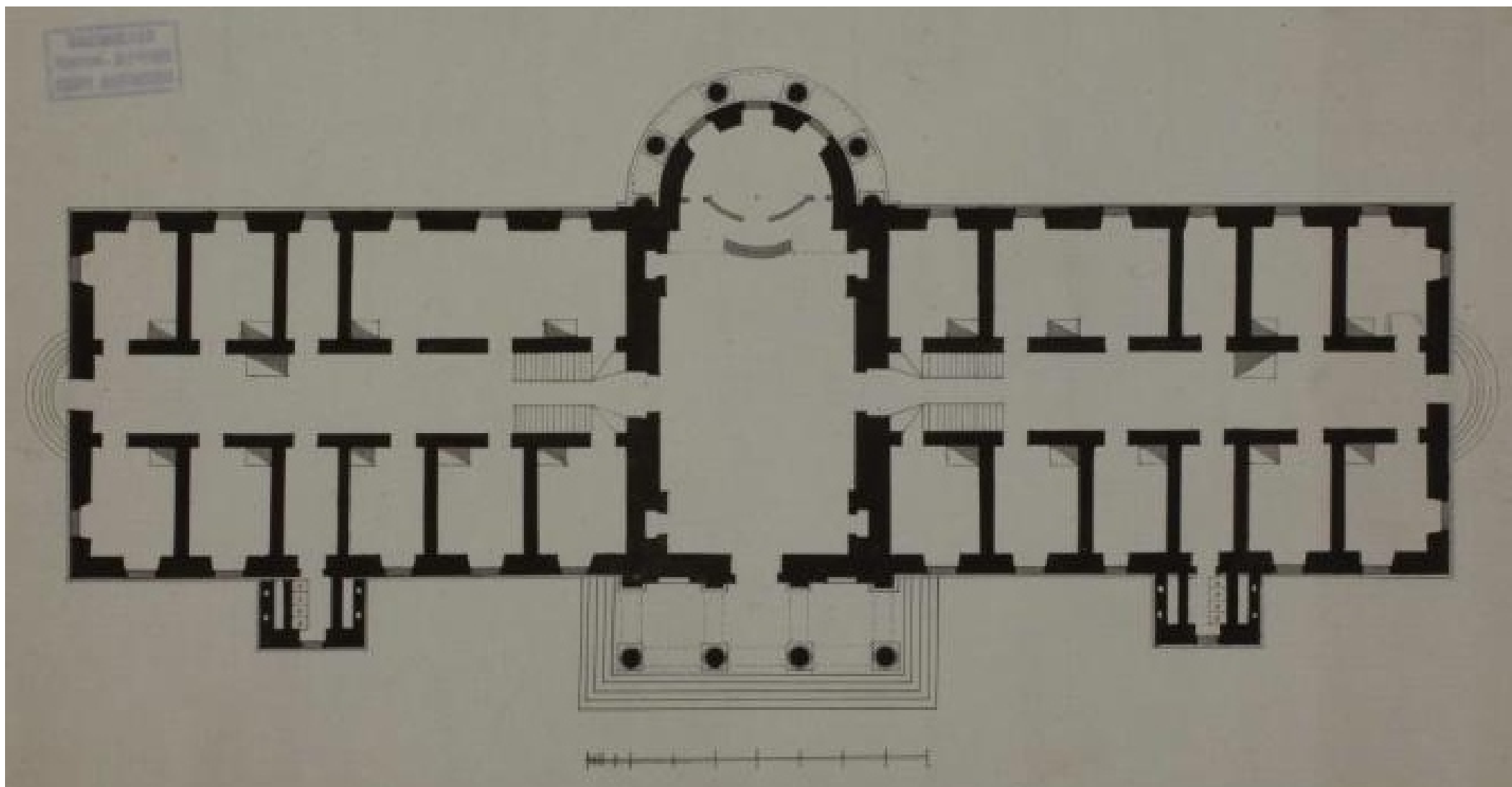
Ил. 13. Кваренги Джакомо (?). Павловск. Мариинский госпиталь. Проект перестройки. План 1-го этажа. Первая половина XIX века /1809 г.?! Хранится: ФГБУК «Государственный музей-заповедник «Павловск», № Ч-440.
