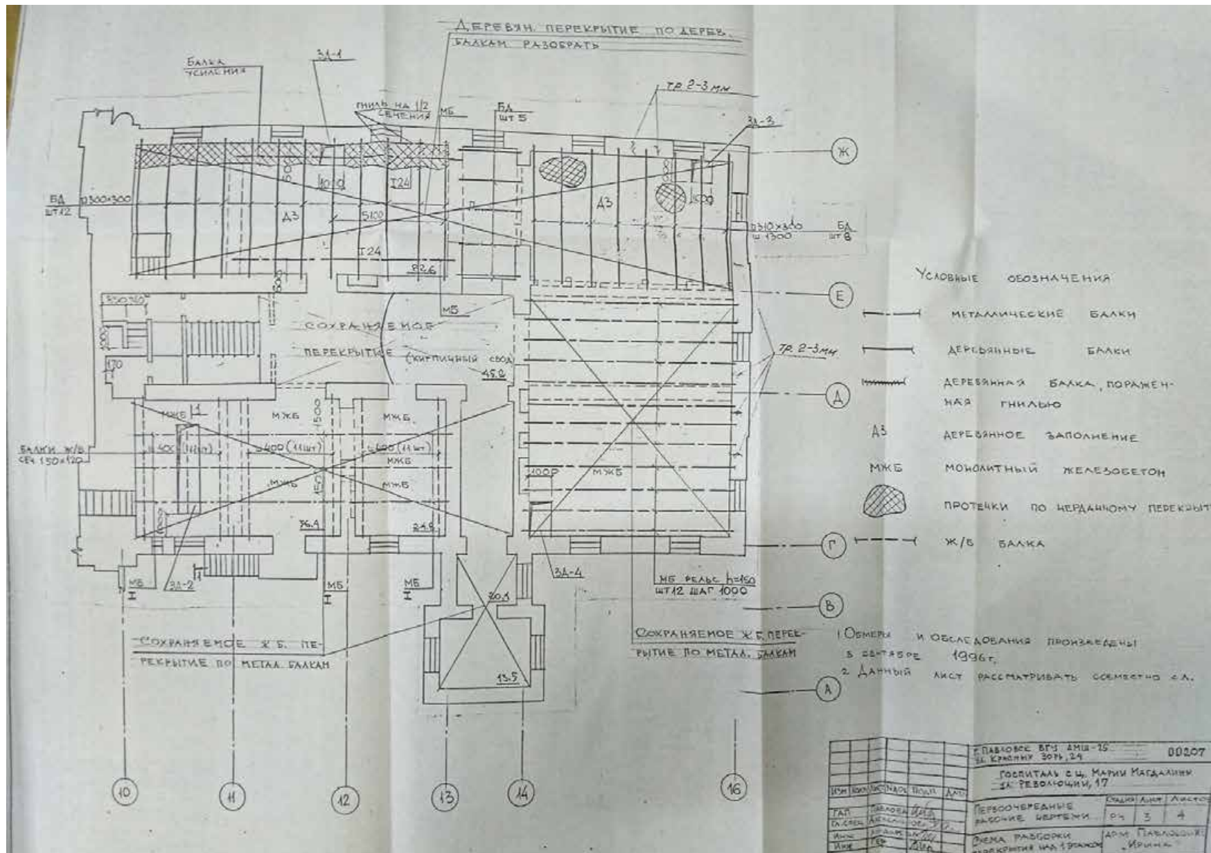
Ил. 49. Госпиталь с ц. Св. Марии Магдалины. ул. Революции, 17. Схема разборки перекрытий над 1 этажом южного корпуса. 1996 г. КГИОП. № 249. Пр-4. г. Павловск. Госпиталь с ц. Св. Марии Магдалины. Проект реставрации и приспособления под детскую музыкальную школу №25. Предварительные работы. Первоочередные рабочие чертежи. Т.1. Кн.2. / ИЧП АРМ Павловой И.Е. "ИРИНА". СПб., 1996.
