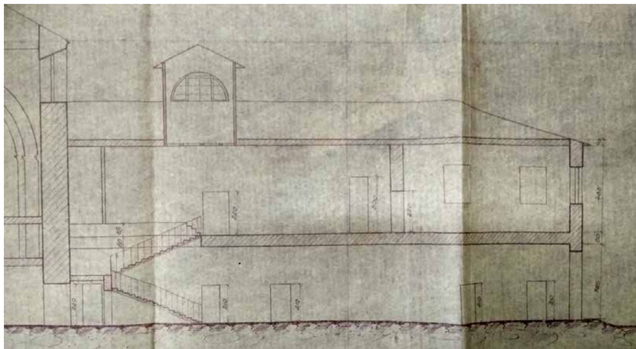
Ил. 35. Павловская ателье "Металлоигрушка". Главный корпус. Продольный разрез. Обмерные чертежи. 1945 г. КГИОП. № 249. Пр-1. Проект восстанов- ления з-да Артели "Точмех" в г. Павловске. Ленинградской обл. Часть 1. Строительно- обмерочные чертежи. / Роскопромпроект. 1946 г.
