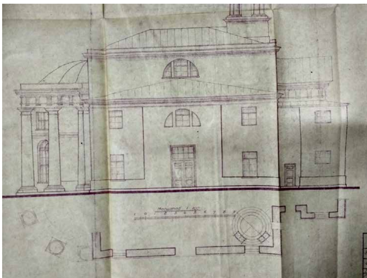
Ил. 29. Павловская ателье "Металлоигрушка". Главный производственный корпус. Боковой /северный/ фасад. 1945 г. КГИОП. № 249. Пр-1. Проект восстановления 3-да Артели "Точмех" в г. Павловске. Ленинградской обл. Часть Архитектурная. / Роскопромпроект. 1946 г.
