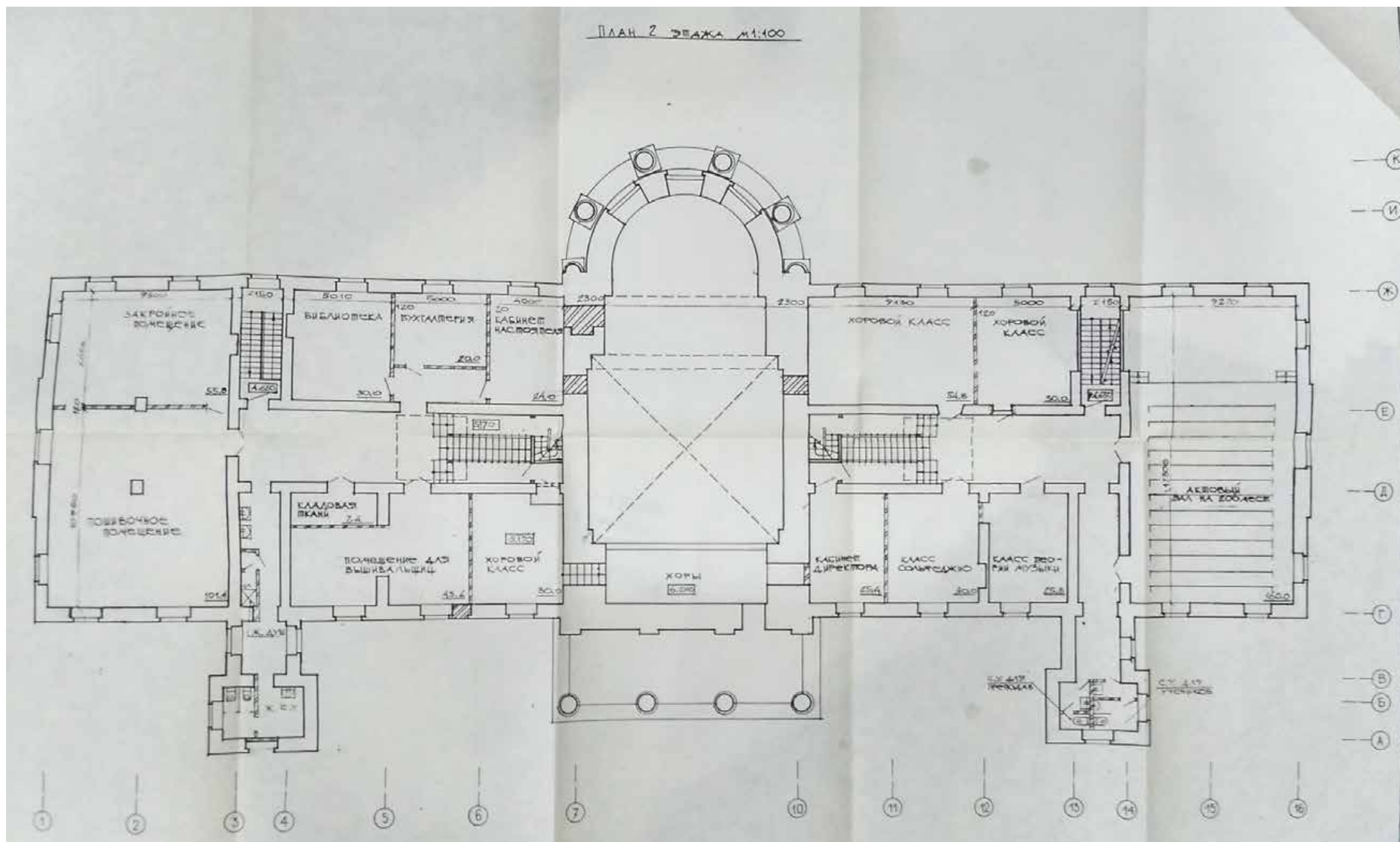
Ил. 67. Госпиталь с церковью Св. Марии Магдалины в г. Павловске. Эскиз. План приспособления помещений 2-го этажа. 1997 г. КГИОП. № 249. Пр-6. г. Павловск. Госпиталь с ц. Св. Марии Магдалины. Проект реставрации и приспособления. Проектные работы. Эскизный проект реставрации и приспособления. СФР. Т.3. Кн.1. / ИЧП АРМ Павловой И.Е. "ИРИНА". СПб., 1997.
