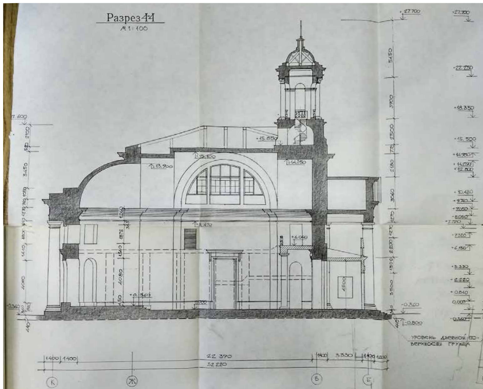
Ил. 60. Госпиталь с церковью Св. Марии Магдалины в г. Павловске. Эскизный проект. Разрезы 4-4. Продольный разрез церкви. 1997 г. КГИОП. № 249. Пр-6. г. Павловск. Госпиталь с ц. Св. Марии Магдалины. Проект реставрации и приспособления. Проектные работы. Эскизный проект реставрации и приспособления. СФР. Т.3. Кн.1. / ИЧП АРМ Павловой И.Е. "ИРИНА". СПб., 1997.
