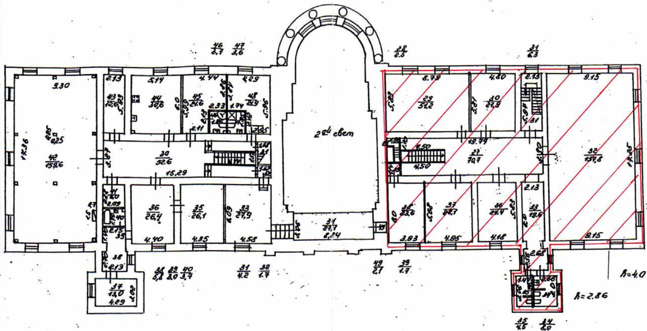
Ил. 71. Санкт-Петербург, г. Павловск. Садовая ул., д. 17, Лит. А. План 2-го этажа. 2006 г. ПИБ Пушкинского района г. Санкт-Петербурга.
