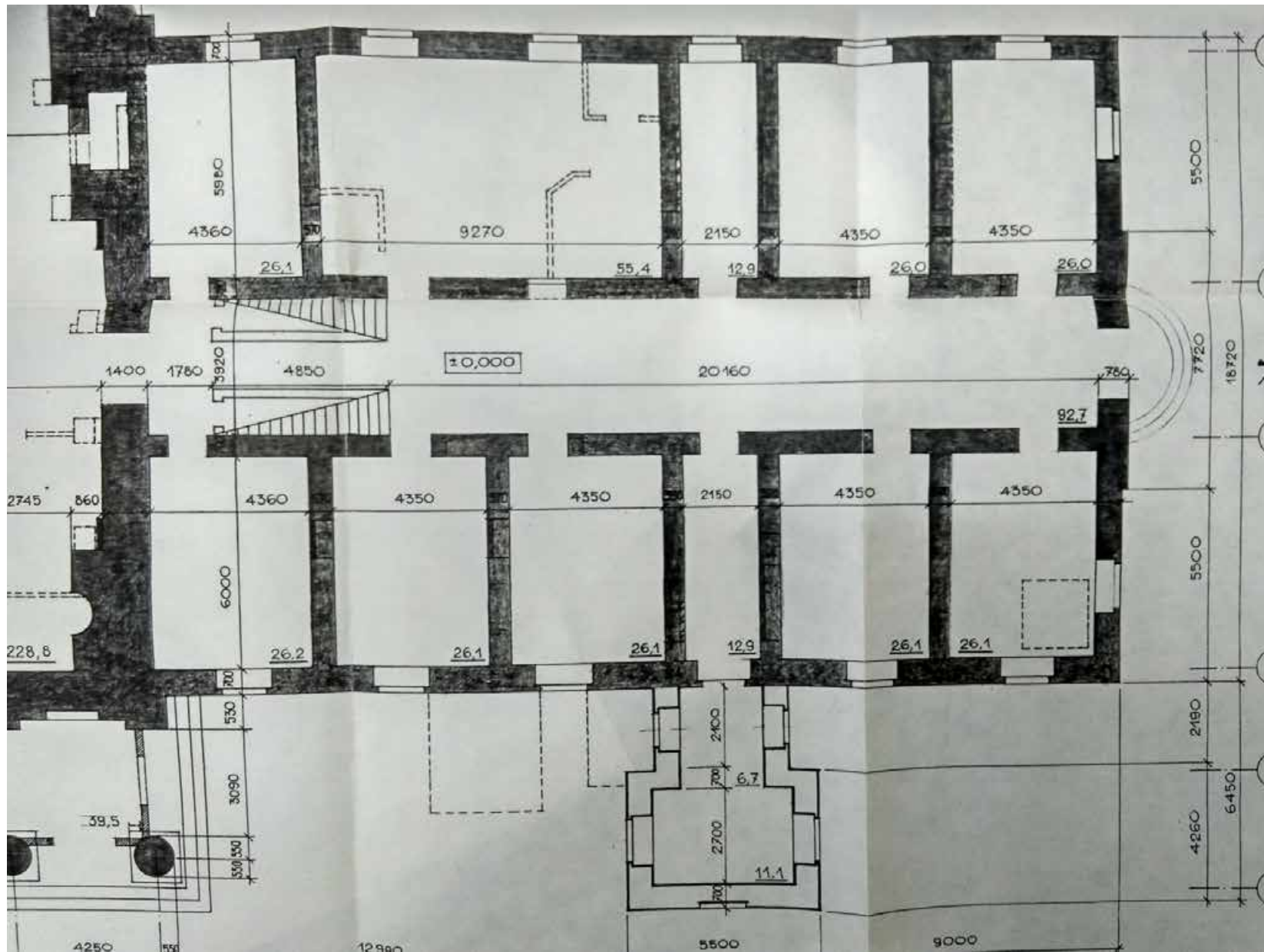
Ил. 52. Госпиталь с церковью Св. Марии Магдалины в г. Павловске. Эскизный проект. План 1-го этажа южного корпуса. 1997 г. КГИОП. № 249. Пр-6. г. Павловск. Госпиталь с ц. Св. Марии Магдалины. Проект реставрации и приспособления. Проектные работы. Эскизный проект реставрации и приспособления. СФР. Т.3. Кн.1. / ИЧП АРМ Павловой И.Е. "ИРИНА". СПб., 1997.
