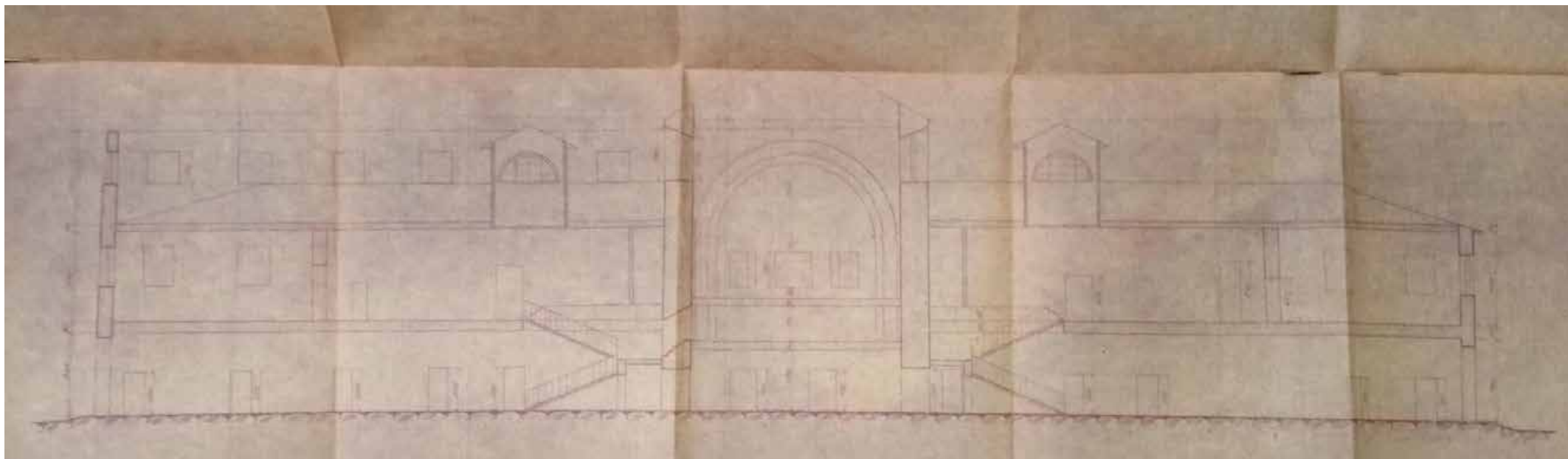
Ил. 35. Павловская ателье "Металлоигрушка". Главный корпус. Продольный разрез. Обмерные чертежи. 1945 г. КГИОП. № 249. Пр-1. Проект восстанов- ления з-да Артели "Точмех" в г. Павловске. Ленинградской обл. Часть 1. Строительно- обмерочные чертежи. / Роскопромпроект. 1946 г.
