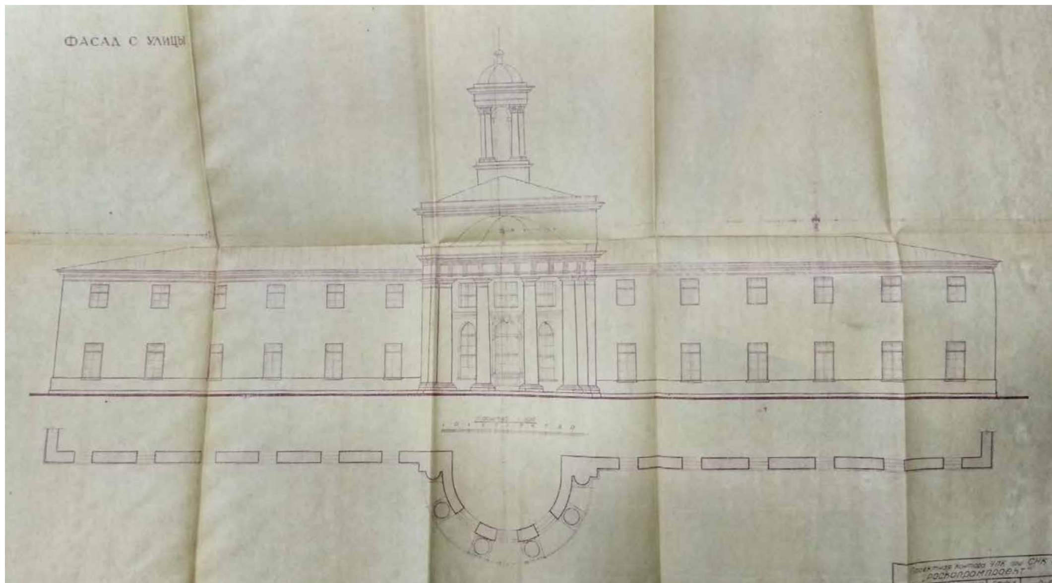
Ил. 27. Павловская ателье "Металлоигрушка". Главный производственный корпус. Фасад с улицы /восточный фасад/. 1945 г. КГИОП. № 249. Пр-1. Проект восстановления з-да Артели "Точмех" в г. Павловске. Ленинградской обл. Часть Архитектурная. / Роскопромпроект. 1946 г.
