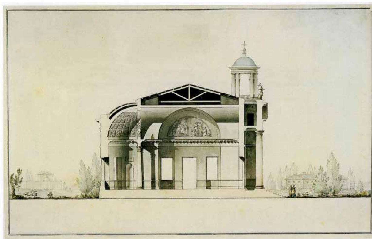
Ил. 9. Московская Славянка. Церковь Преображения Господня. Продольный разрез. Арх. Дж. Кваренги. 1780 г. Оpubл.: Джакомо Кваренги. Архитектурная графика. Коллекция ГМИ СПб. Научный каталог. Автор-сост. А.М. Павелкина. СПб., 1998. С.60.
