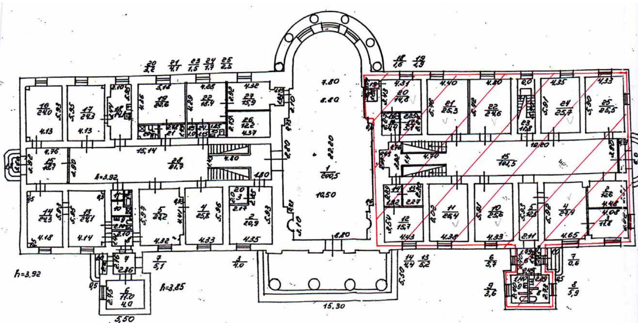
Ил. 70. Санкт-Петербург, г. Павловск. Садовая ул., д. 17, Лит. А. План 1-го этажа. 2006 г. ПИБ Пушкинского района г. Санкт-Петербурга.
