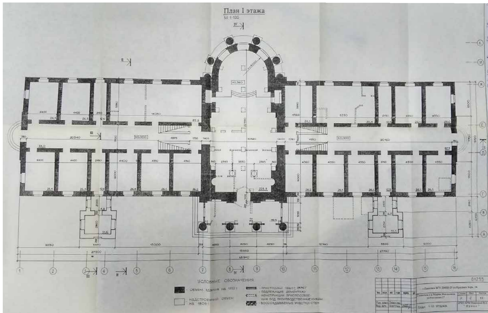
Ил. 51. Госпиталь с церковью Св. Марии Магдалины в г. Павловске. Эскизный проект. План 1-го этажа. 1997 г. КГИОП. № 249. Пр-6. г. Павловск. Госпиталь с ц. Св. Марии Магдалины. Проект реставрации и приспособления. Проектные работы. Эскизный проект реставрации и приспособления. СФР. Т.3. Кн.1. / ИЧП АРМ Павловой И.Е. "ИРИНА". СПб., 1997.
