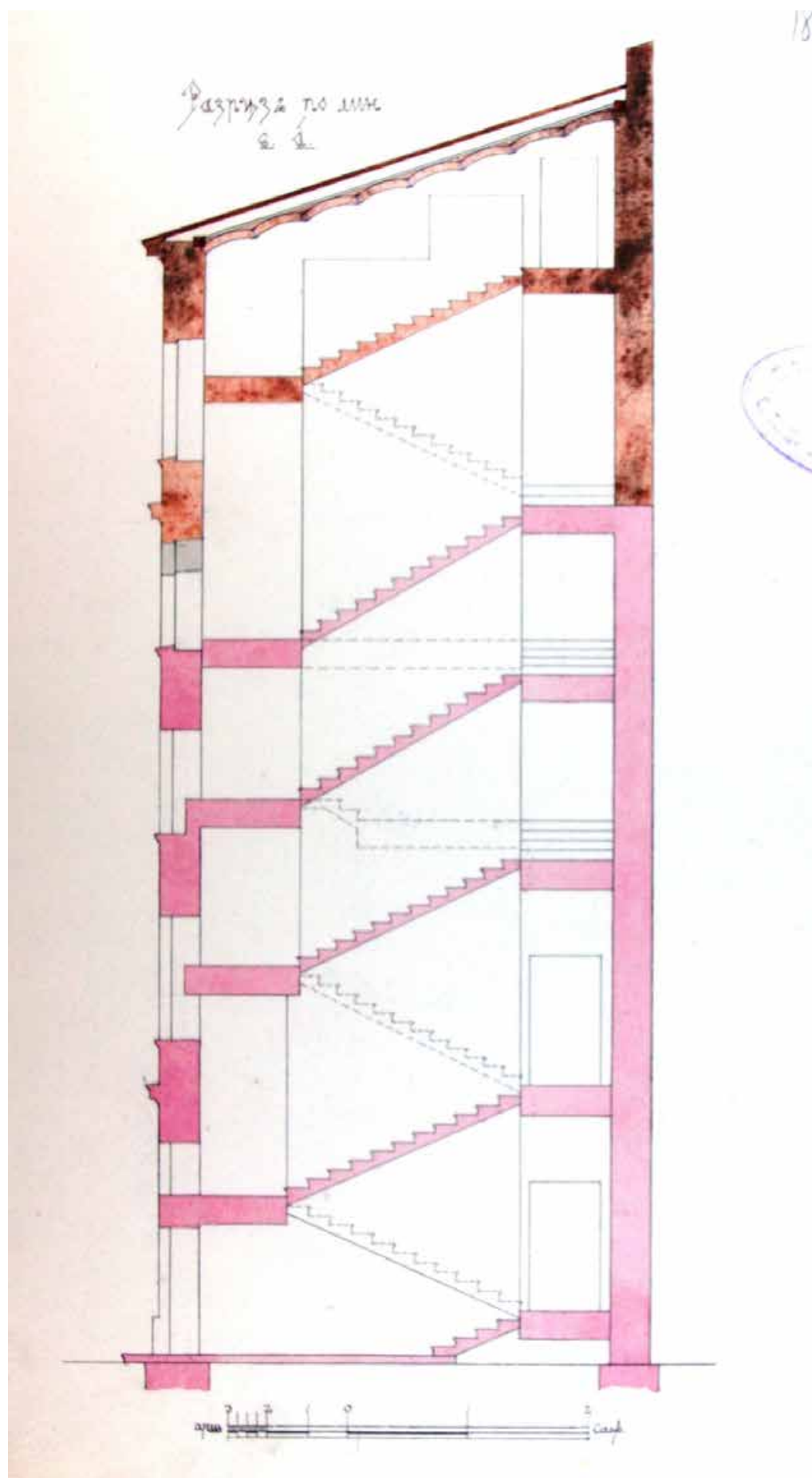
12. Разрез по линии в-о флигеля А дома князя Гагарина. Арх. Н. Л. Бенуа. 1898
