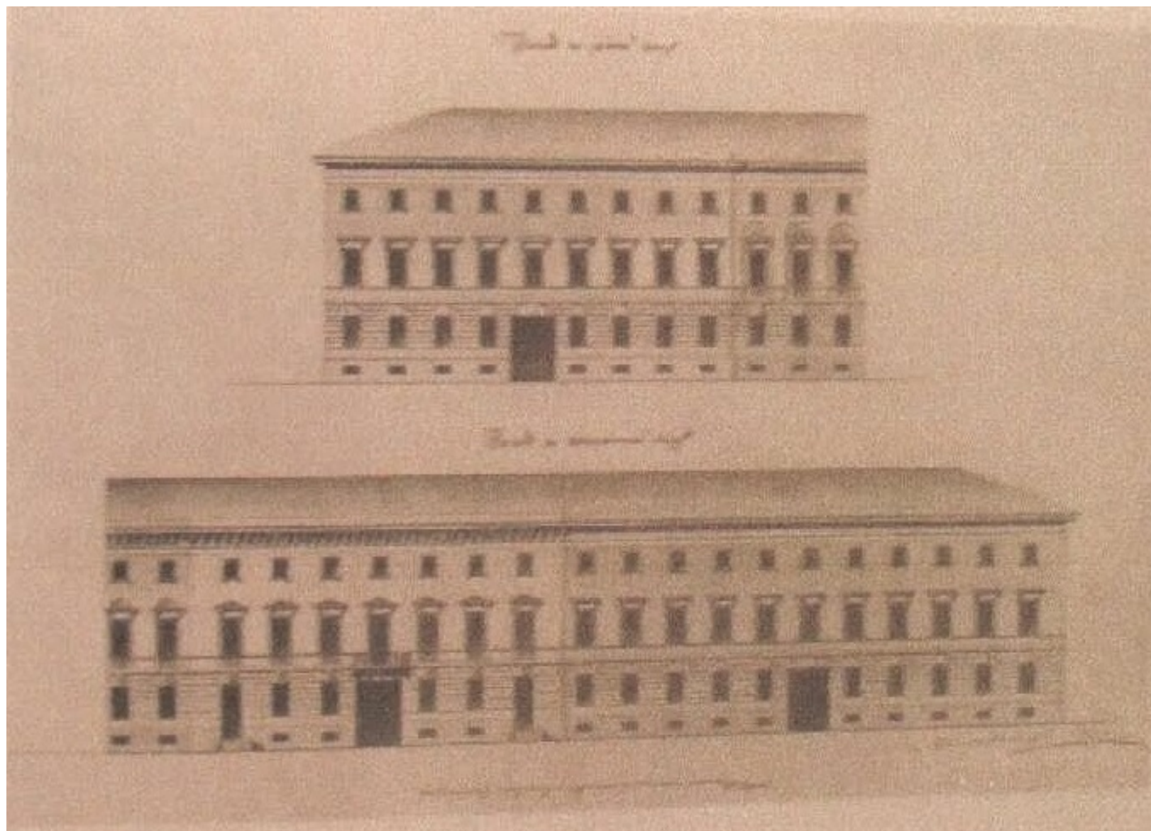
3. Проект фасадов обывательских домов на Михайловской площади К.И.Росси. 1820-е
