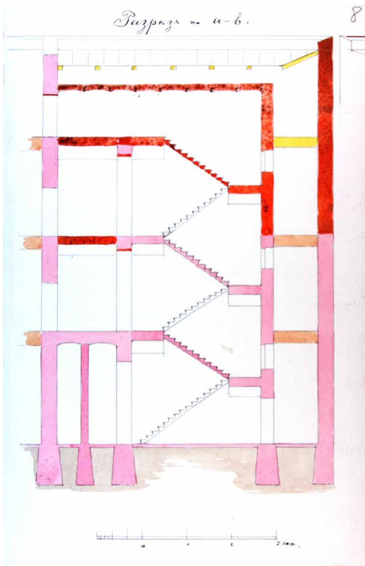
9. Разрез по линии а-в флигеля А дома князей Гагариных. Арх. Н. Л. Бенуа. 1895
