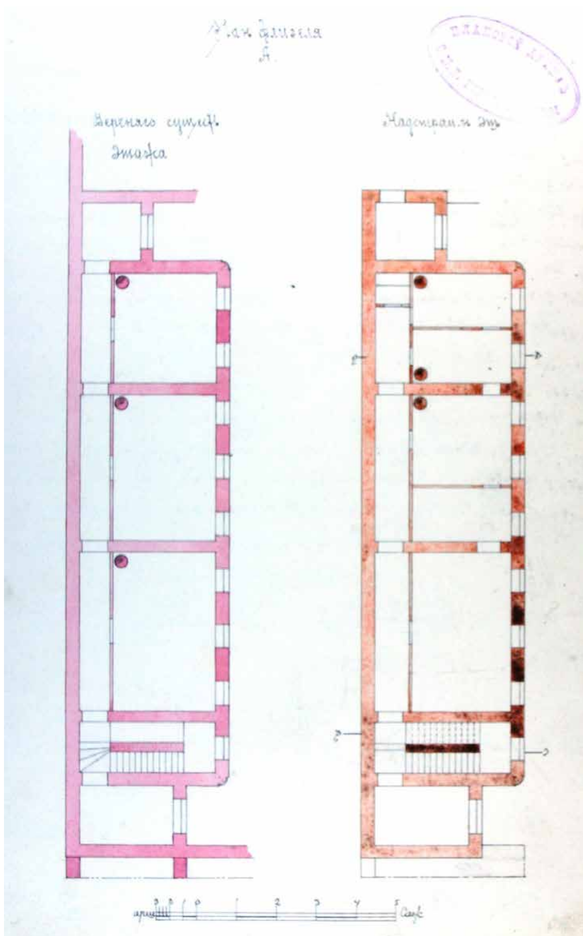
11. План флигеля А дома князя Гагарина. Арх. Н. Л. Бенуа. 1898
