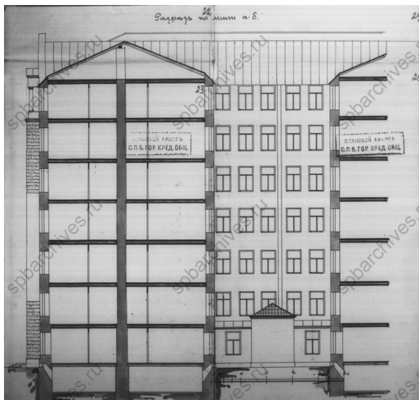
28. Разрез по линии аб. 1912 г. Чертежи дома Э.Э.Арнольда по 18-й линии В.О., 196. ЦГИА СПб. Фонд 515. Опись 4. Дело 2980
