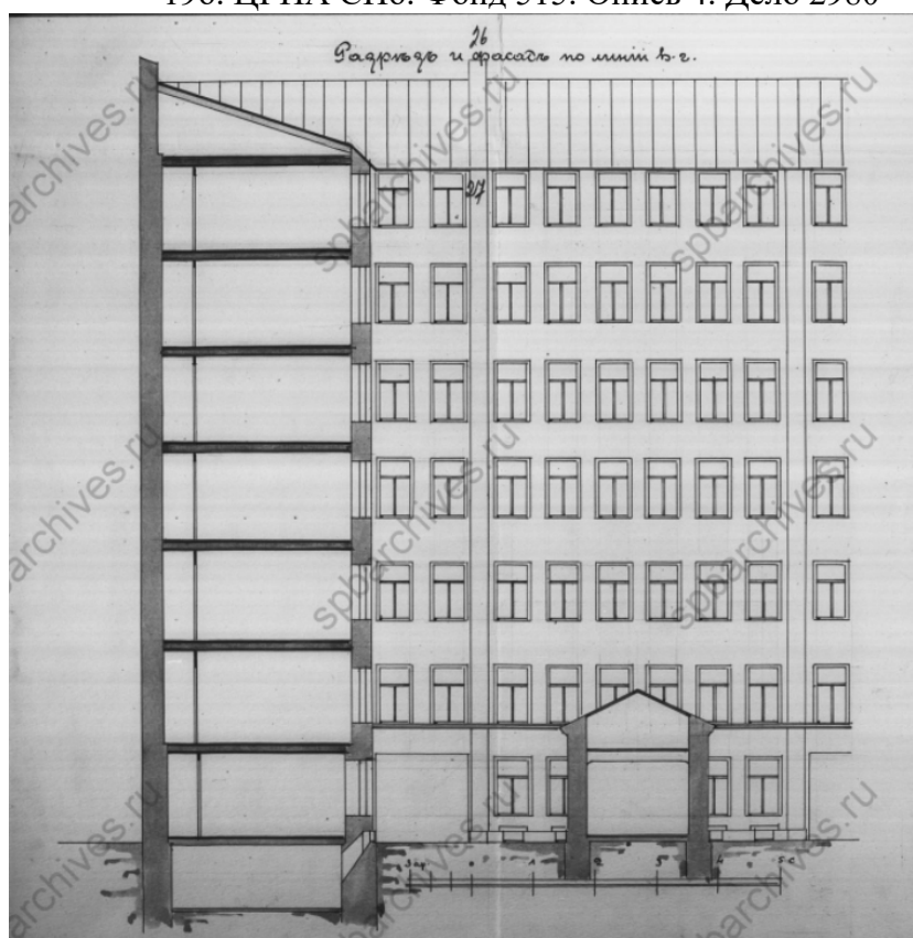
29. Разрез и фасад по линии вг. 1912 г. Чертежи дома Э.Э.Арнольда по 18-й линии В.О., 196. ЦГИА СПб. Фонд 515. Опись 4. Дело 2980
