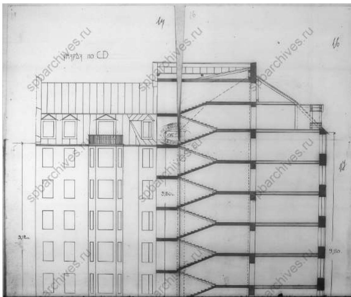
Разрез дома, принадлежащего В.П. Кончиллову, находящегося в Рождественской части уч.1 по Консисторской ул. под № 5.. ЦГИА СПб. Ф.513. оп.102. д.9119.
