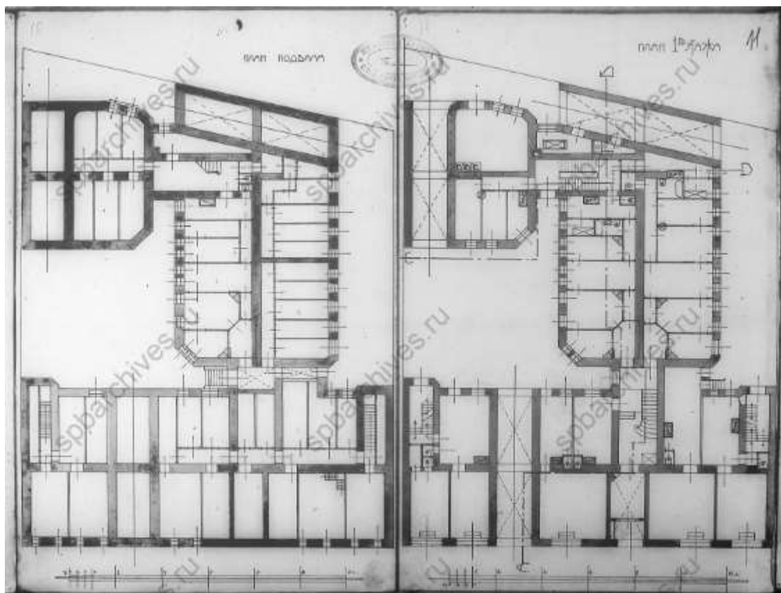
План подвала и 1-ого этажа дома, принадлежащего В.П. Кончиелову, находящегося в Рождественской части уч.1 по Консисторской ул. под № 5. ЦГИА СПб. Ф.513. оп.102. д.9119.
