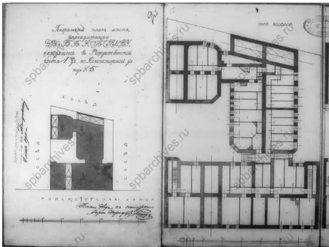
Генеральный план места, принадлежащего В.П. Кончиелову, находящегося в Рождественской части уч.1 по Консисторской ул. под № 5 .1910. ЦГИА СПб. Ф.513. оп.102. д.9119.
