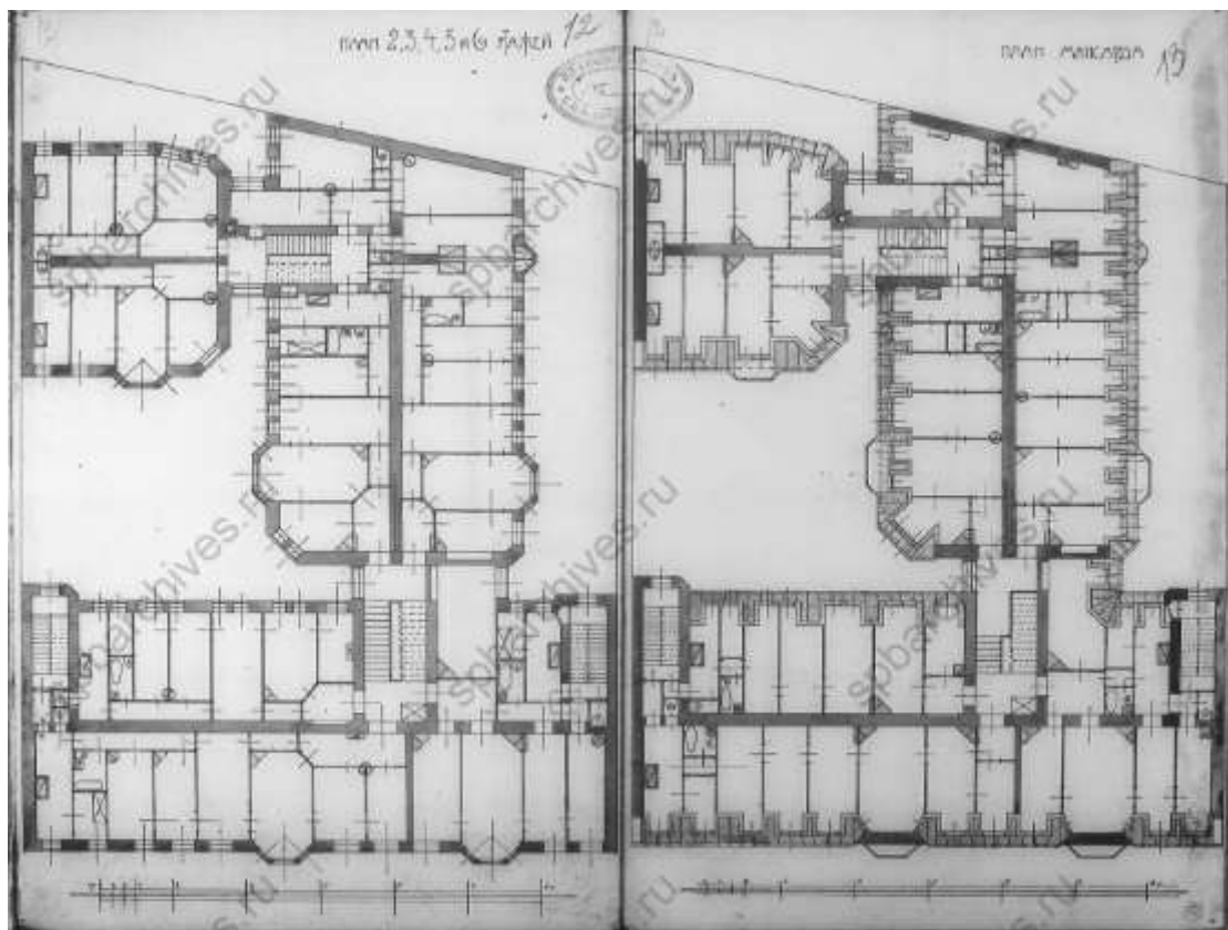
План 2,3,4,5 и 6-ого этажей и мансарды дома, принадлежащего В.П. Кончиелову, находящегося в Рождественской части уч.1 по Консисторской ул. под № 5.. ЦГИА СПб. Ф.513. оп.102. д.9119.
