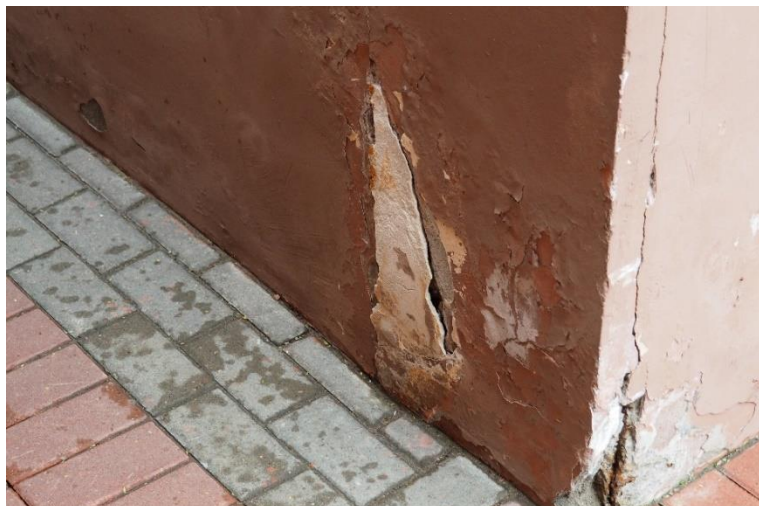
23. «Машинное отделение №6 с котельной» в составе ансамбля «Комплекс главной станции Санкт-Петербургских городских водопроводов», ул. Таврическая, д. 10, лит. А. Западный фасад. Фрагмент. Фото 08.08.2022г.
