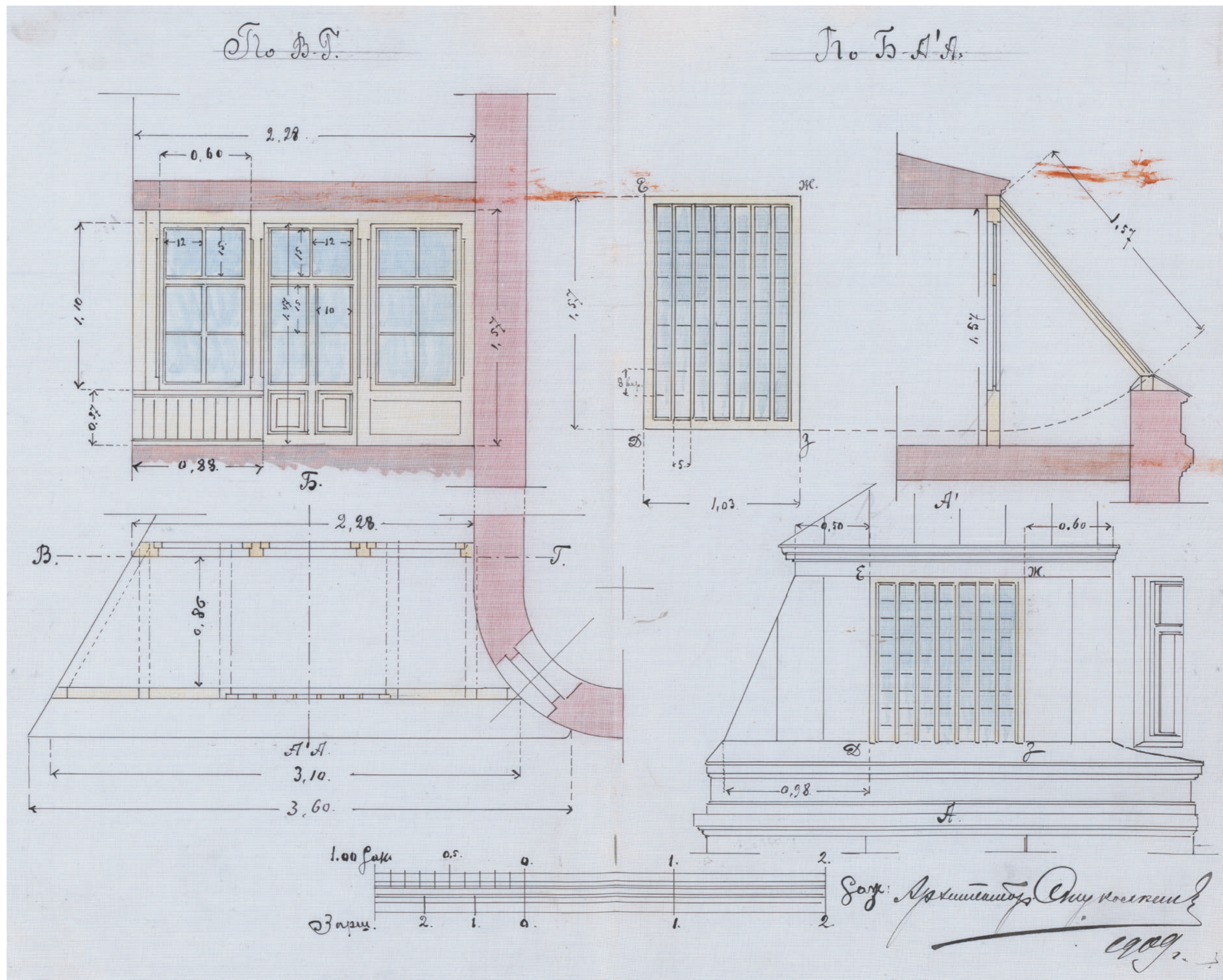
Ил. 36 А. Стекло́нная галере́я дома №20 по Фонтанке. План, фасады А, Б, разрезы по ВГ, по Б-А' А. Архитектор Стуколкин, 1909 г. РГИА. Ф. 475. Оп. 1. Д. 518. Л. 3.
