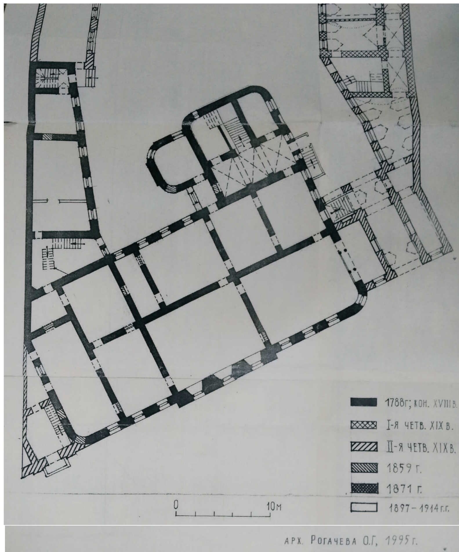
Ил. 80. Дом Голицына (Дом Министерства Императорского Двора). Строительная история лицевого дома с пристройками. План 1-го этажа. Архитектор О.Г. Рогачева, 1995 г. Опубл.: КГИОП. п.179. №667 п. Паспорт. Дом Министерства Императорского Двора (Дом Голицына). С.-Петербург, Центральный район, наб. р. Фонтанки, д. 20. / Автор: Рогачева О. Г. СПб., 1995 г.
