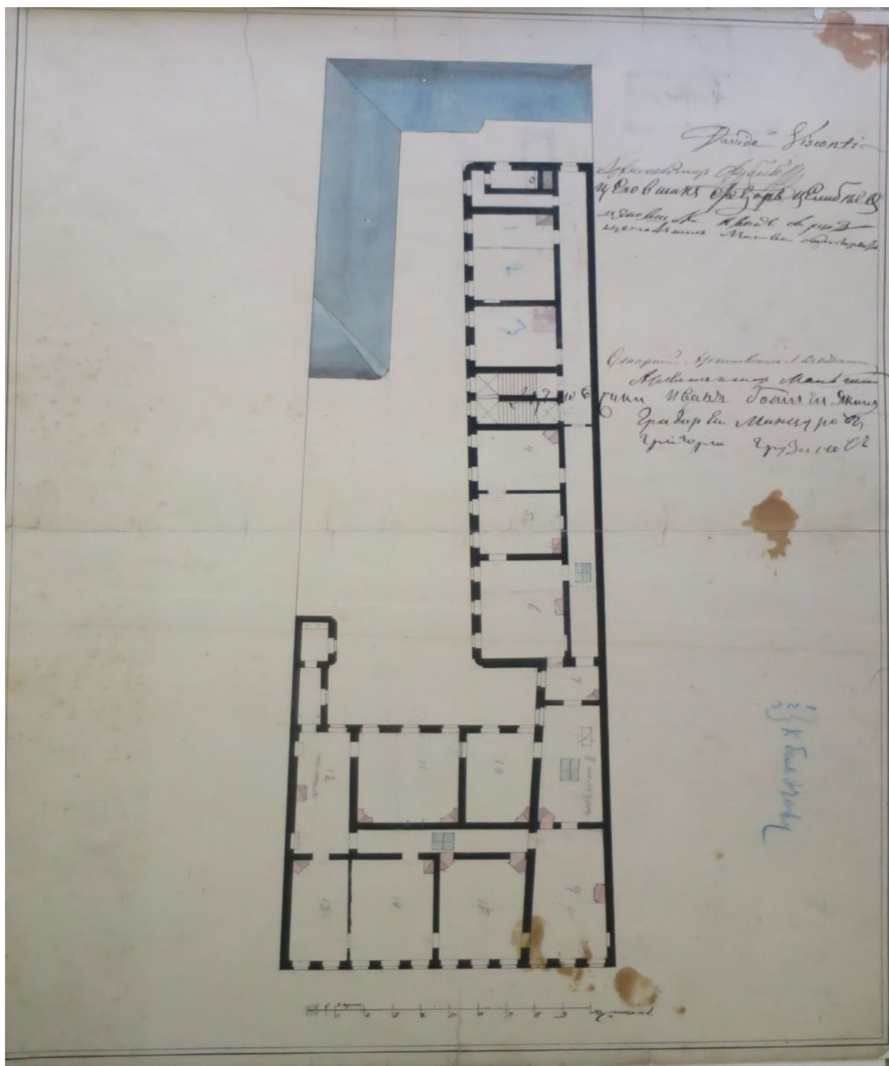
17. Дом купца Ф.И. Ильин на Фонтанке. Обмерный (фиксационный (?)) чертеж. План третьего этажа. Подписано Д. Висконти. Без даты (начало XIX в.). Архив КГИОП. 429/Г-4. 16832.
