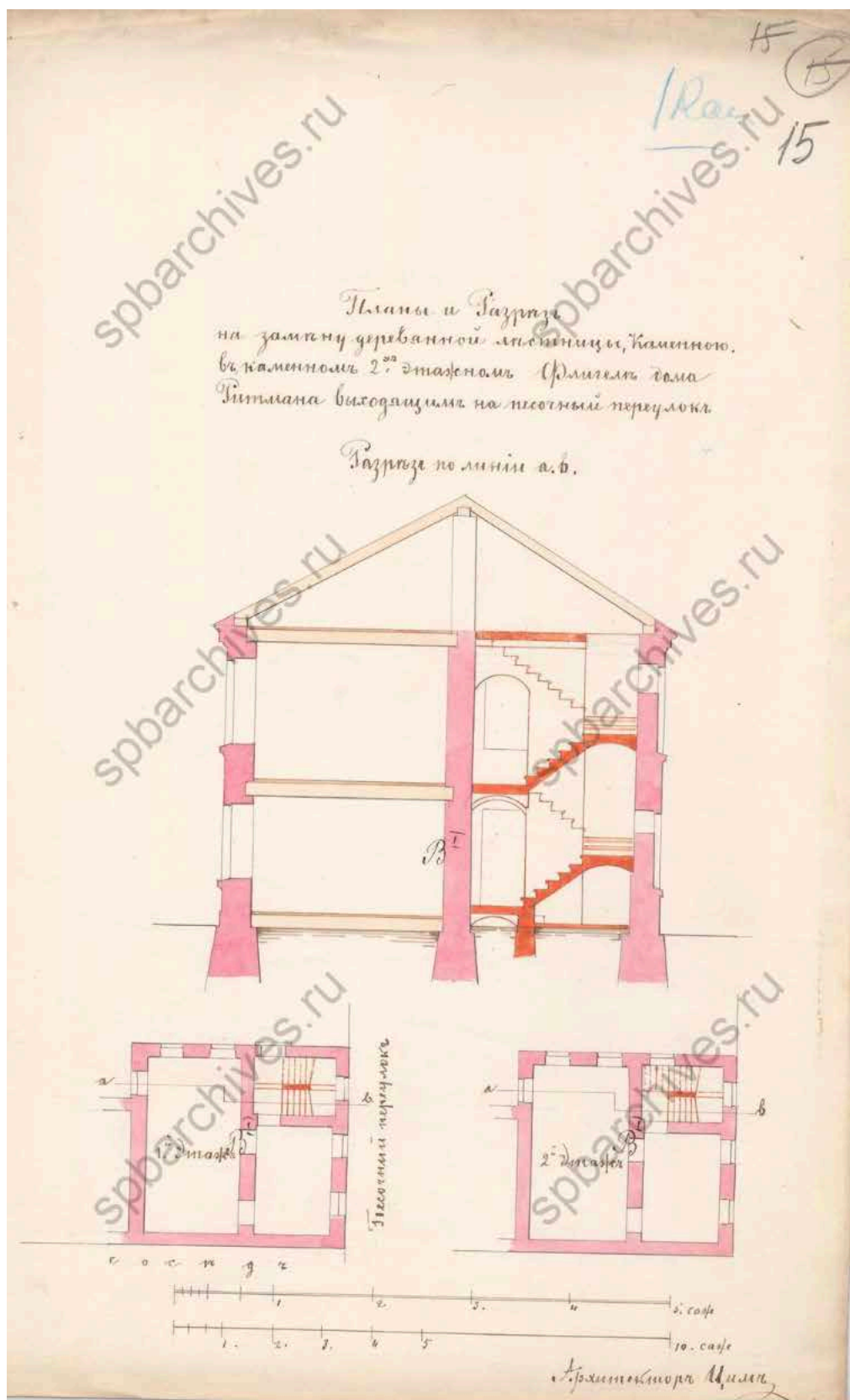
35. Планы и разрез. ЦГИА СПб. Фонд 513. Опись 102. Дело 1465 Чертежи дома на участке, принадлежавшем Ошеметковой, И.Фрику, Г.Ритману, совладельцам И.П.Козлову и С.Н.Белорукову по 1-й линии В.О., 16 и Соловьевскому пер., 15
