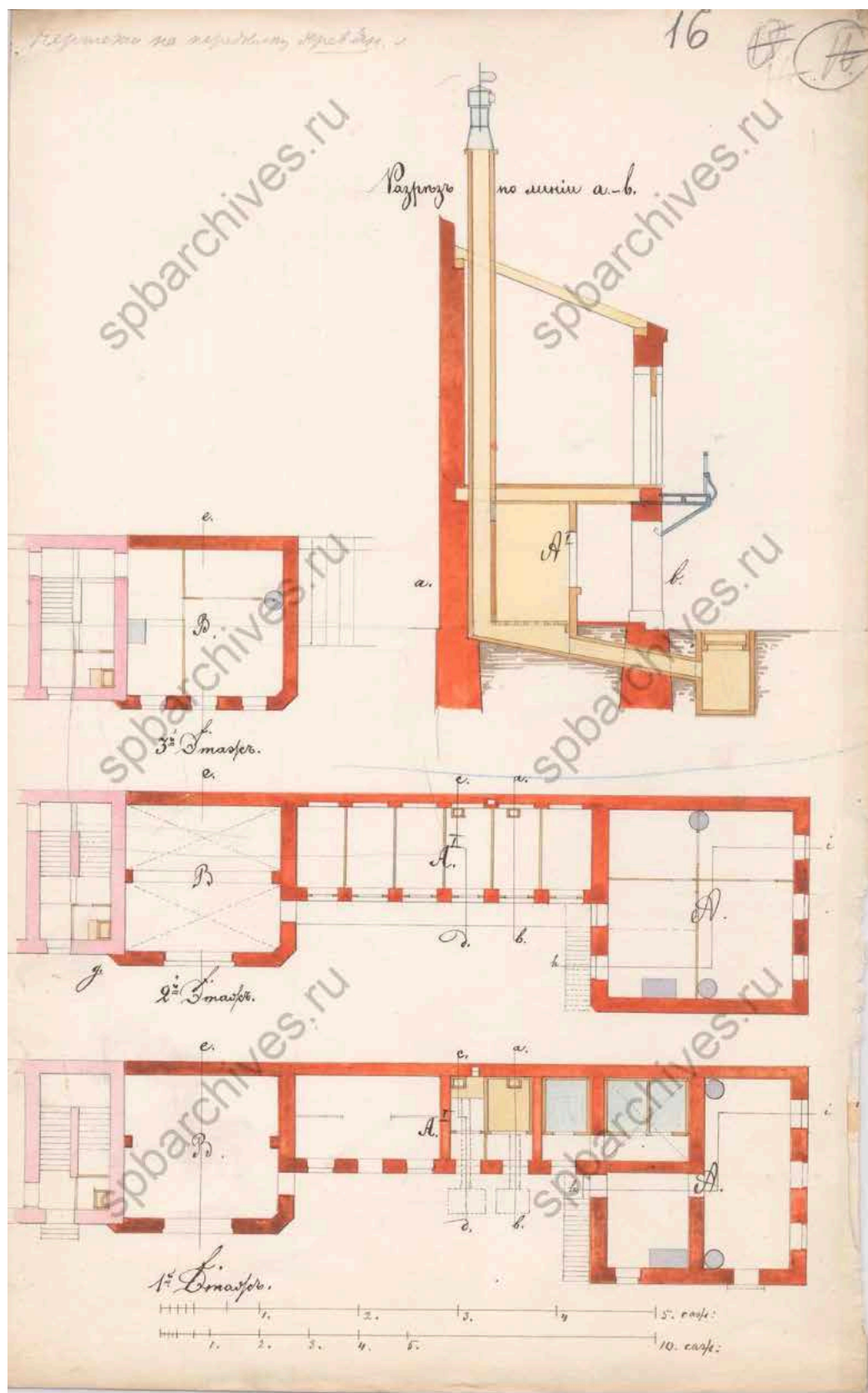
36. Планы и разрез. ЦГИА СПб. Фонд 513. Описание 102. Дело 1465
