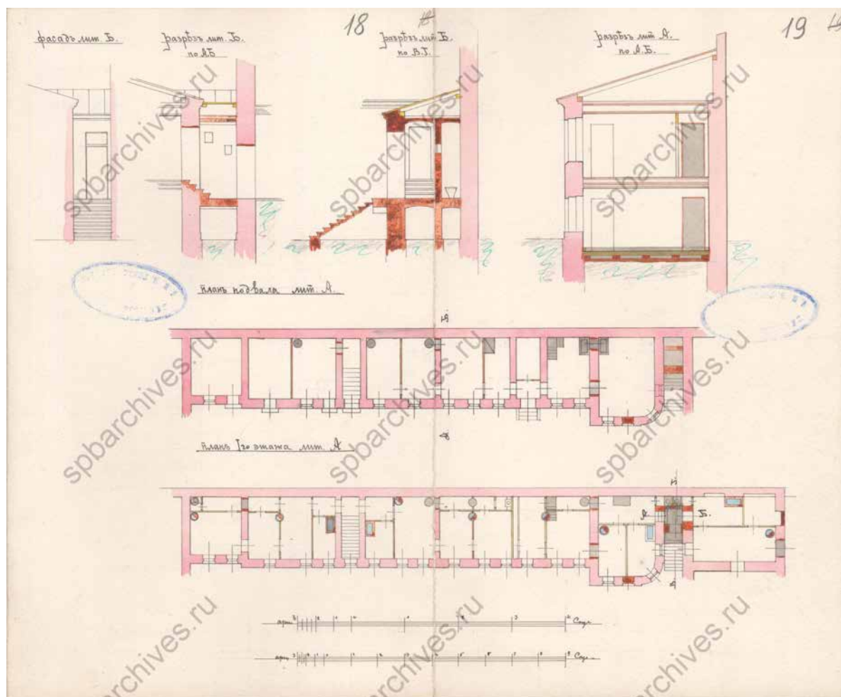
38. Планы и разрезы. ЦГИА СПб. Фонд 513. Опись 102. Дело 1465
