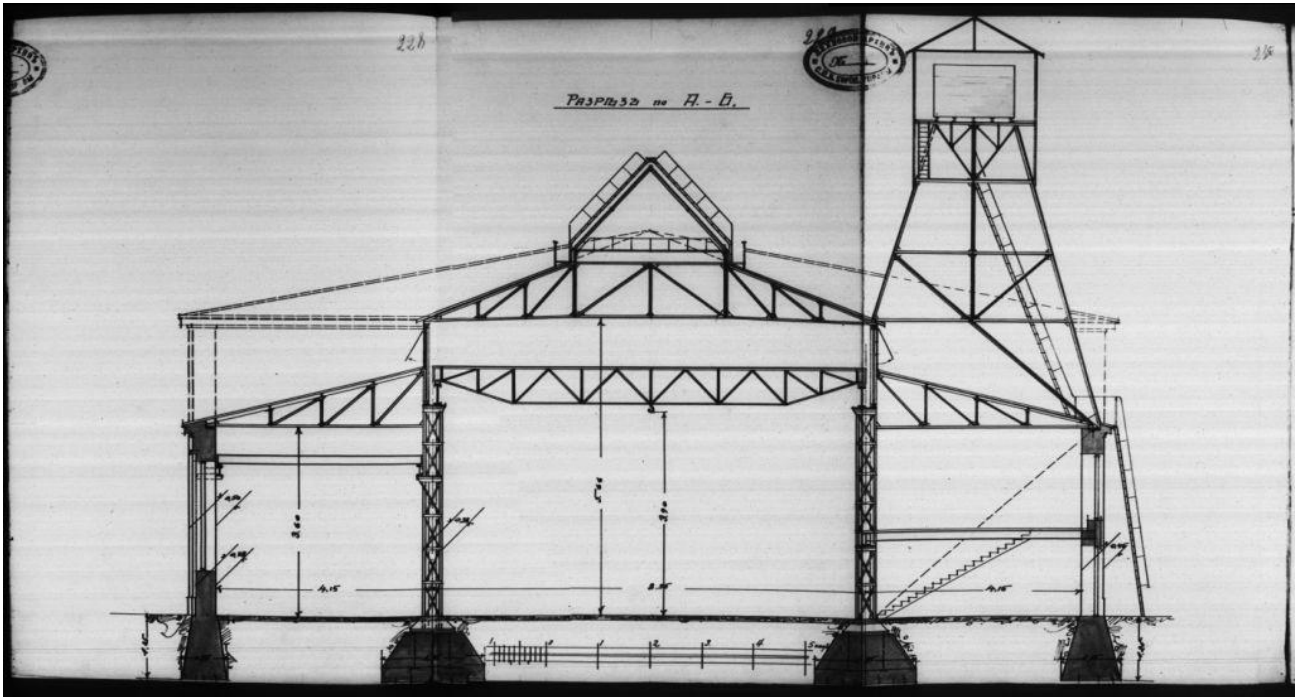
Илл. 27. Проект постройки чугунолитейного цеха. Разрез. Архитектор Ф. Лидваль. 1912 г. ЦГИА СПб Ф. 513. Оп. 102. Д. 2859. Л. 228-230.
