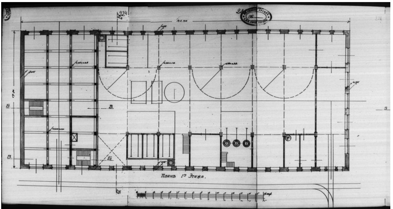
Илл. 26. Проект постройки чугунолитейного цеха. План. Архитектор Ф. Лидваль. 1912 г. ЦГИА СПб Ф. 513. Оп. 102. Д. 2859. Л. 224-226.
